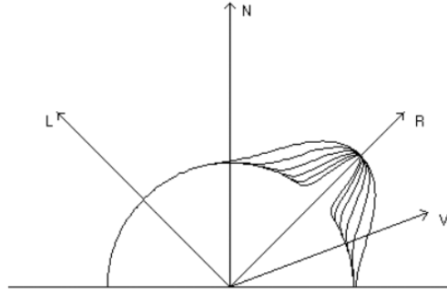
Slika 9.6: Utjecaj faktora n na zrcalnu komponentu svjetlosti.
