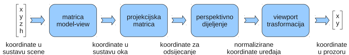
Slika 6.17: Proces obrade vrhova pri generiranju konačne slike
