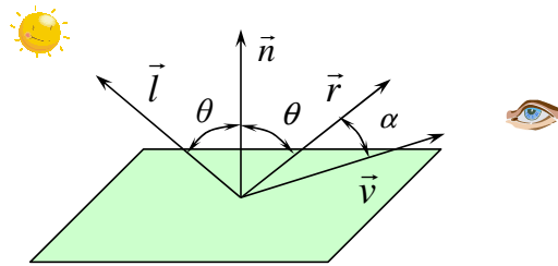
Slika 9.5: Određivanje zrcalne komponente svjetlosti.
