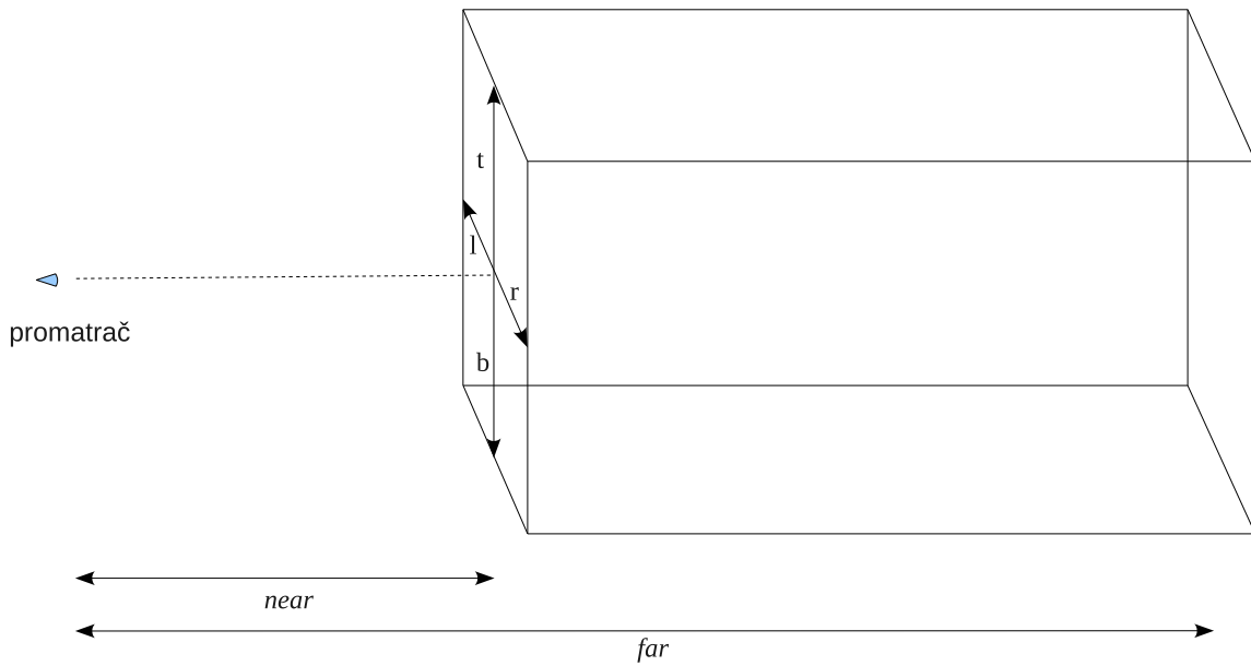
Slika 6.21: Model koji koristi naredba glOrtho
