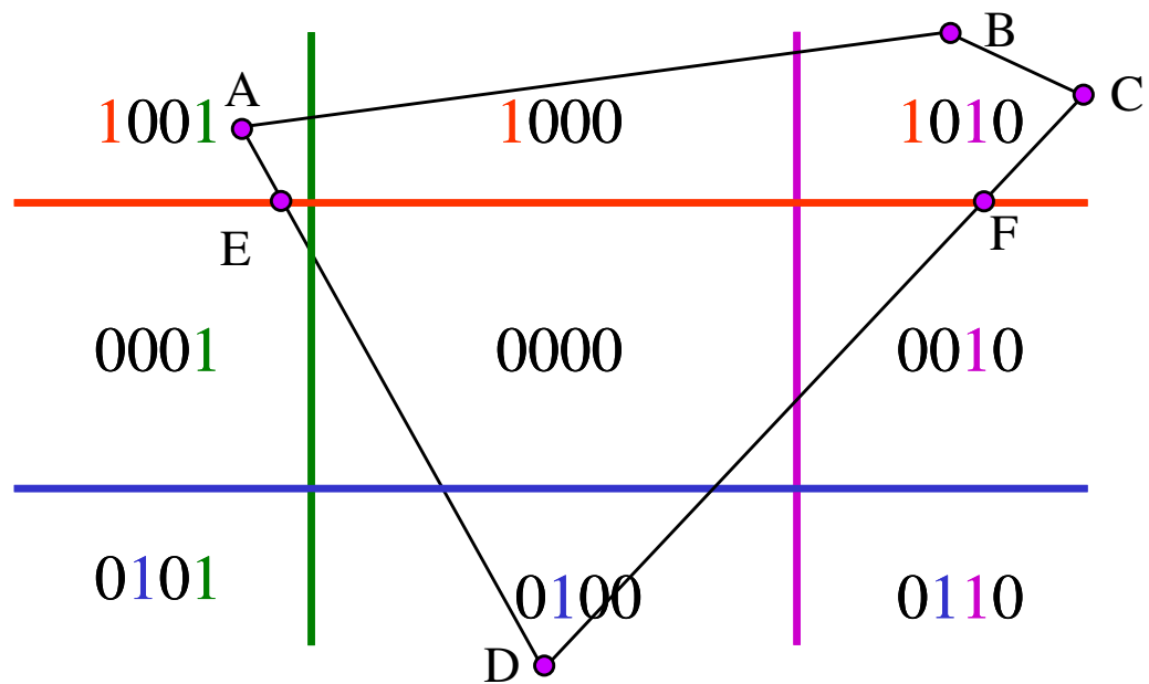
Slika 8.21: Primjer odsijecanja poligona kod algoritma Cohen Sutherlanda.
