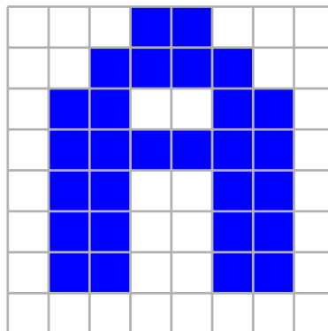
Slika 7.10: Prikaz slova A definiranog rasterskom maskom
