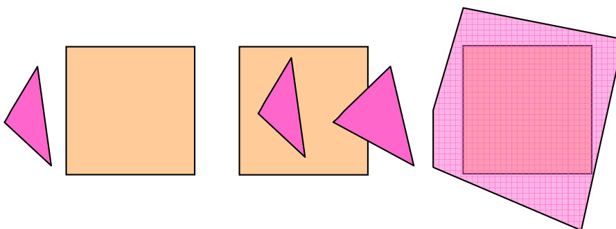
Slika 8.15: Warnockov postupak mogući slučajevi: poligon je izvan prozora (1), poligon je u prozoru ili siječe prozor (2), poligon prekriva prozor (3)
