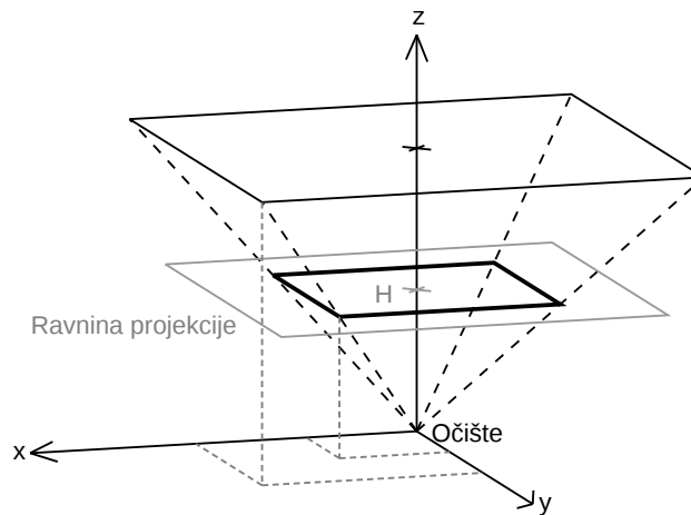
Slika 6.4: Perspektivna projekcija, analiza x -koordinate
