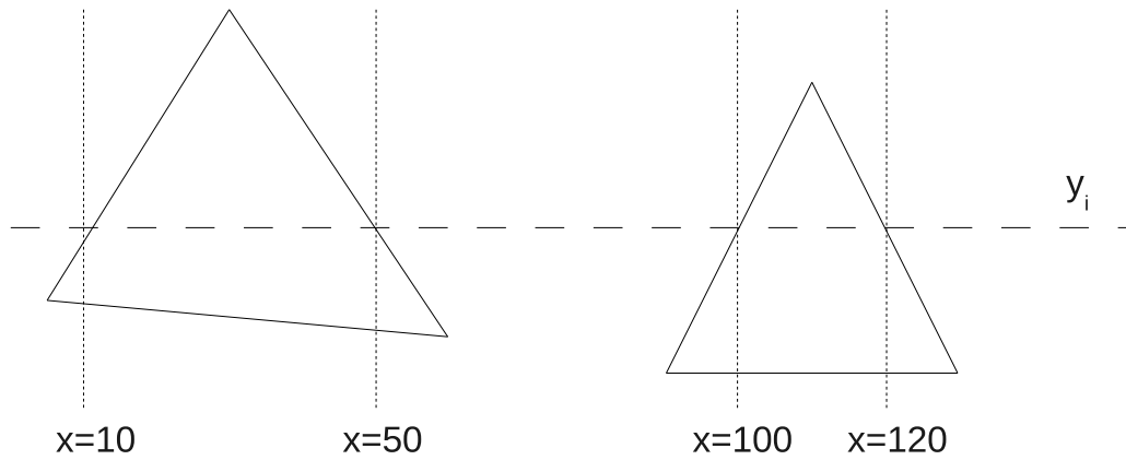
Slika 8.9: Watkinsov postupak: dva disjunktna trokuta
