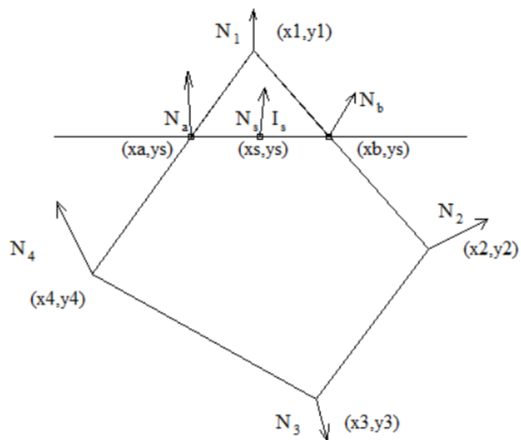
Slika 9.12: Interpolacija normala kod Phongovog sjenčanja, detaljniji primjer
