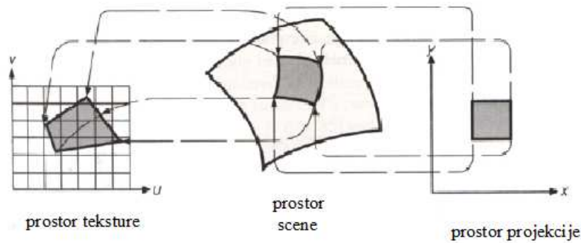
Slika 12.4: Određivanje vrijednosti slikovnog elementa u prostoru projekcije.
