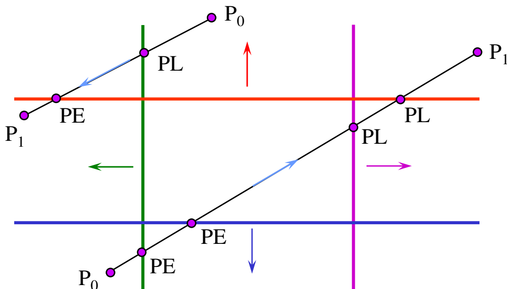
Slika 8.24: Razvrstavanje sjecišta na PE i PL .
