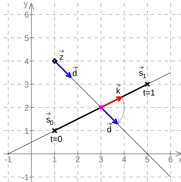
Slika B.2: Utvrđivanje orijentacije sjecišta
