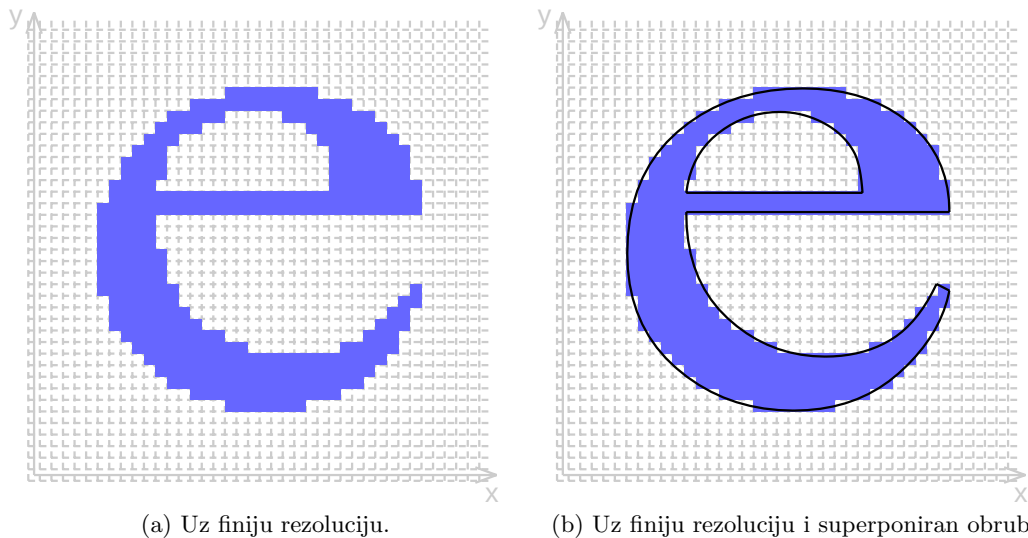
Slika 7.15: Rezultat popunjavanja unutrašnjosti slova uz dovoljnu rezoluciju rastera.
