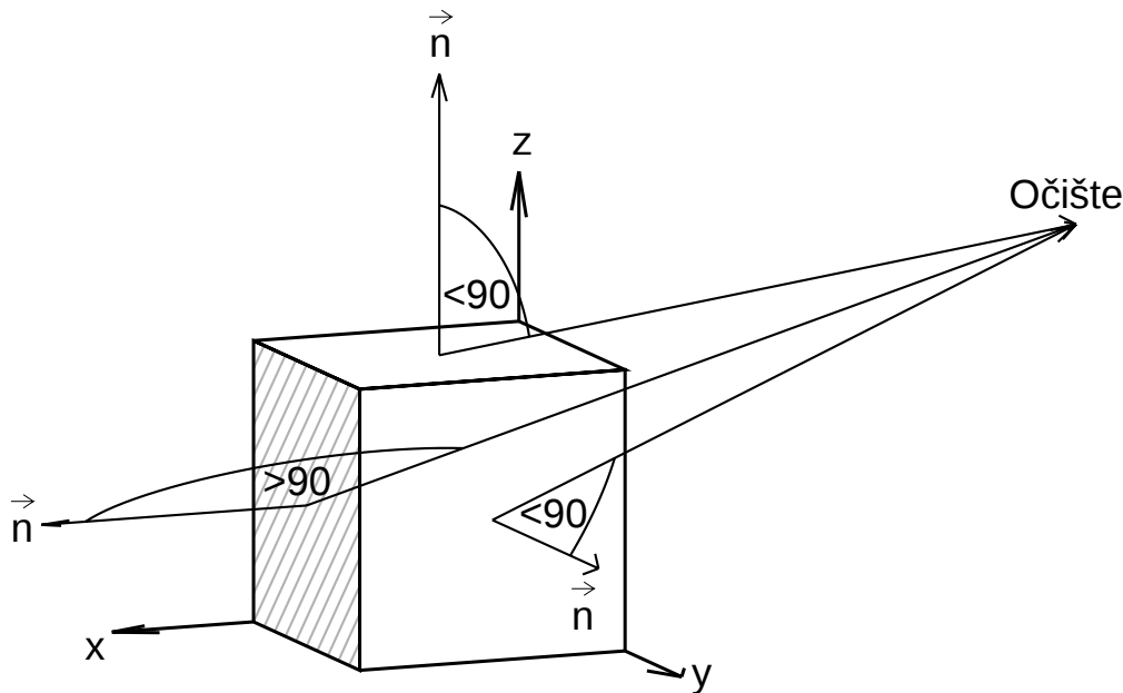
Slika 8.2: Uklanjanje poligona na osnovi kuta između vektora normale poligona i vektora prema promatraču
