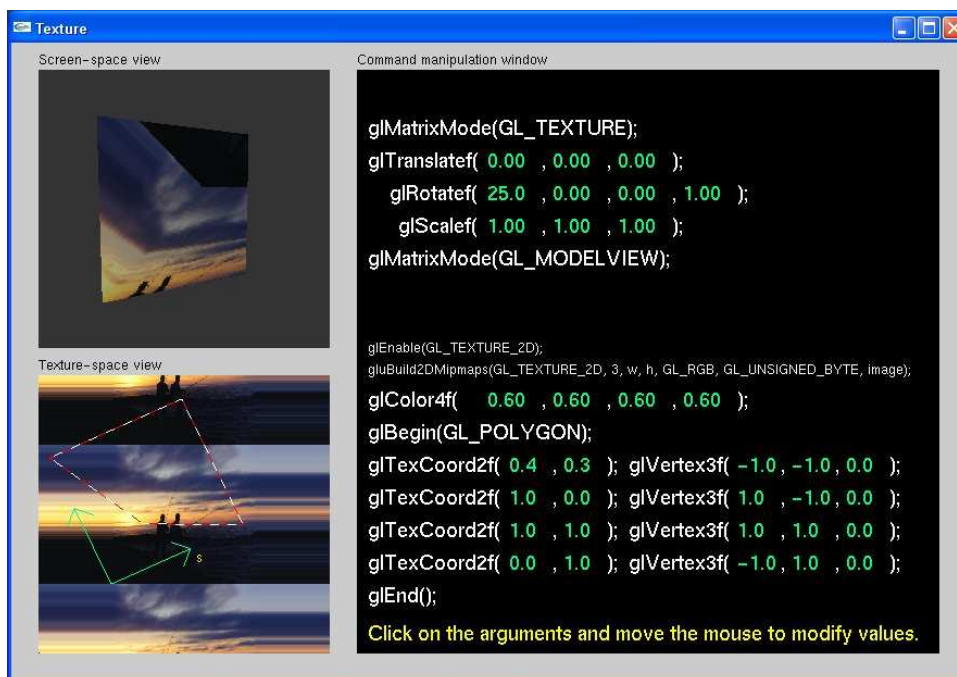
Slika 12.11: Podešavanje područja tekstuure u OpenGLu.
