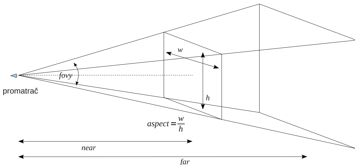
Slika 6.20: Model koji koristi naredba gluPerspective
