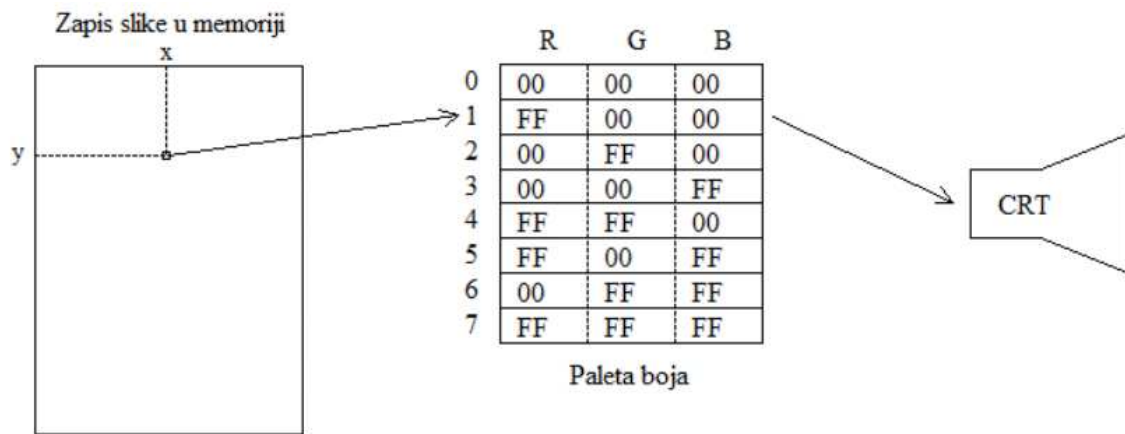
Slika 11.16: Pamćenje boja u paleti boja
