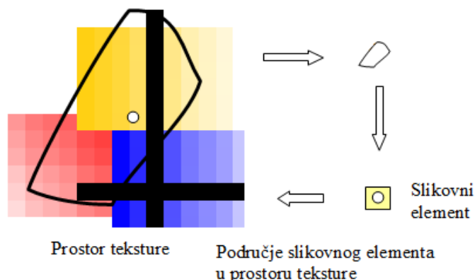
Slika 12.6: Problem neželjenog učinka aliasa pri preslikavanju teksture.
