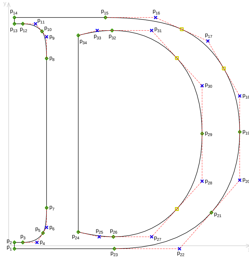
Slika 7.13: Glyph pridružen slovu D s označenim točkama i njihovim statusima. Zeleni rombovi predstavljaju on -točke, plavi križići off -točke a žučkasti kvadratići virtualne točke
