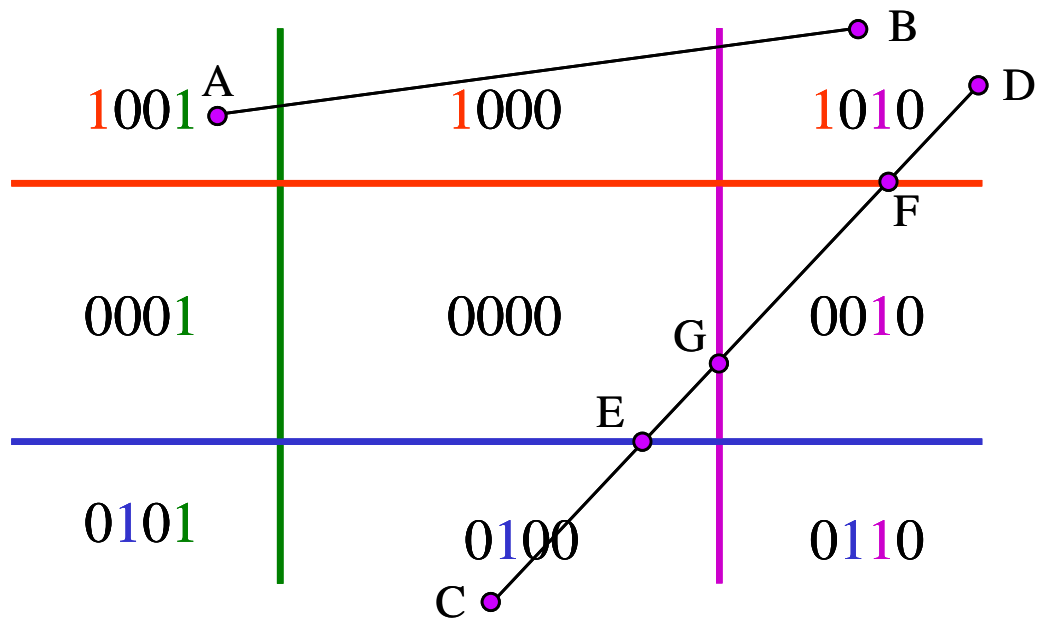
Slika 8.20: Primjer odsijecanja dužine kod algoritma Cohen Sutherlanda.
