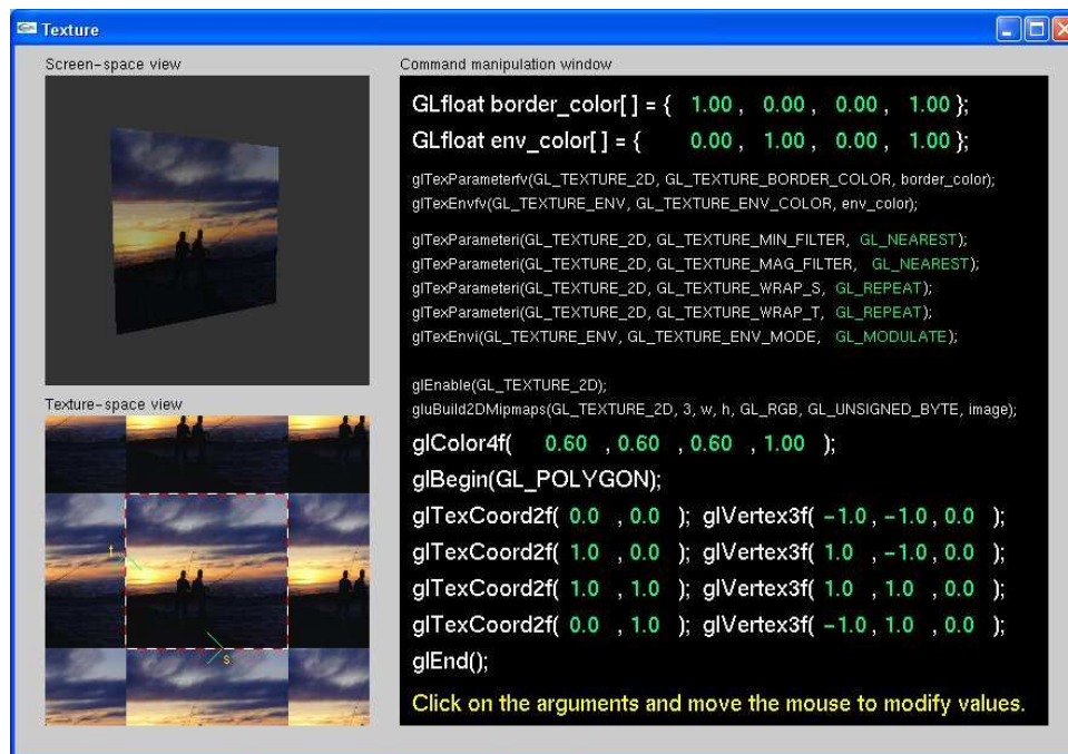
Slika 12.10: Preslikavanje tekstuure u OpenGL-u.
