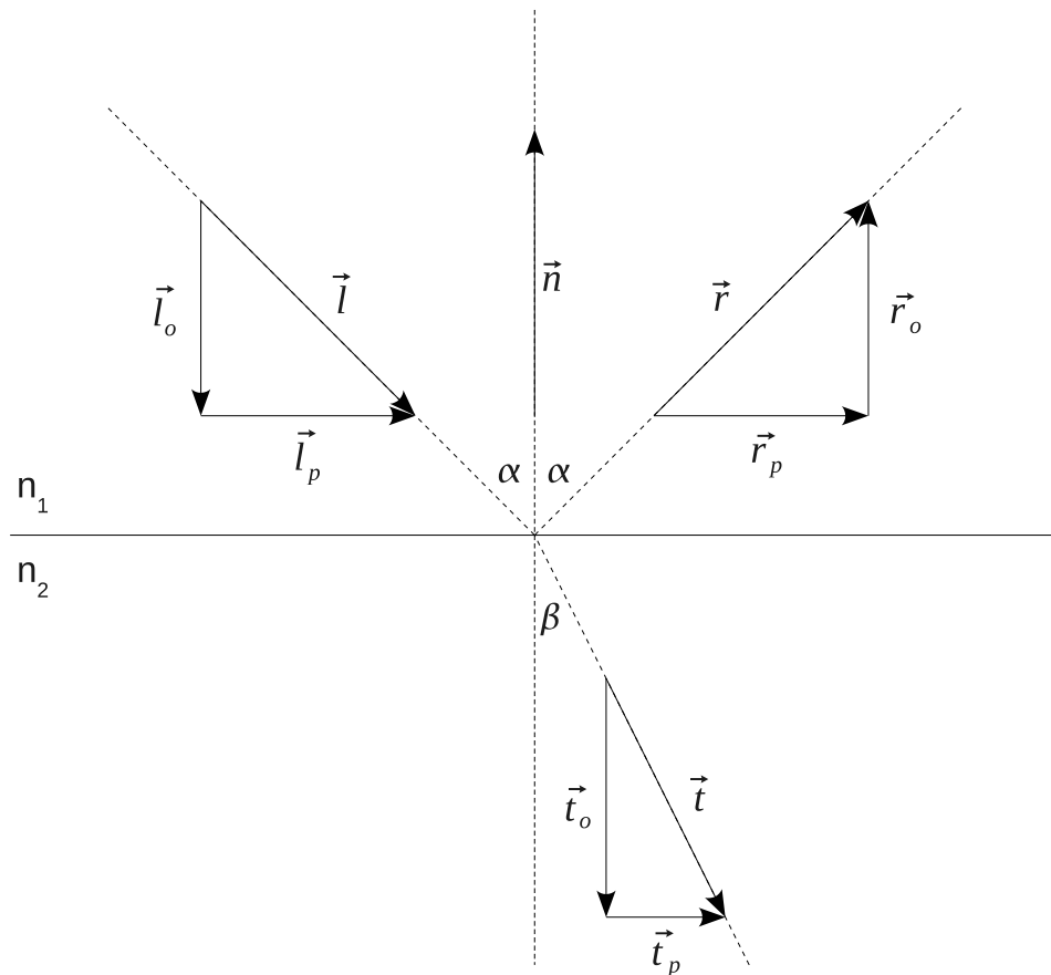
Slika 10.4: Izračun reflektirane i lomljene zrake
