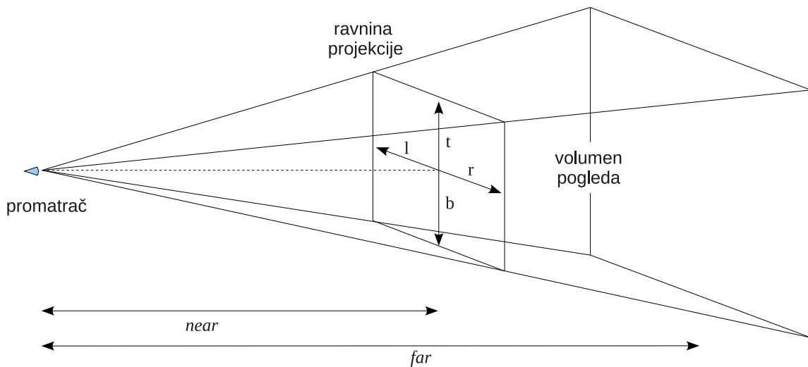
Slika 6.18: Model koji koristi naredba glFrustum
