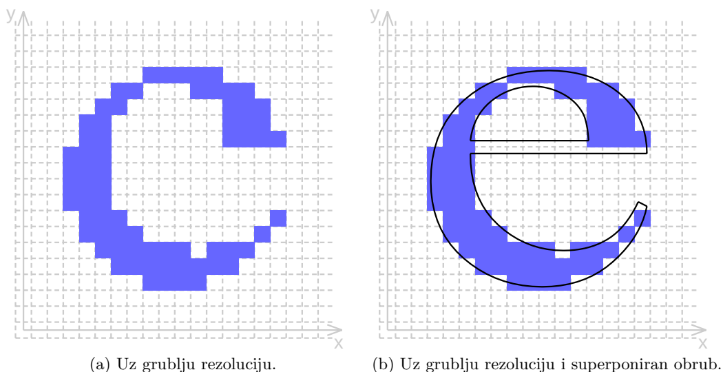
Slika 7.16: Rezultat popunjavanja unutrašnjosti slova uz nedovoljnu rezoluciju rastera.
