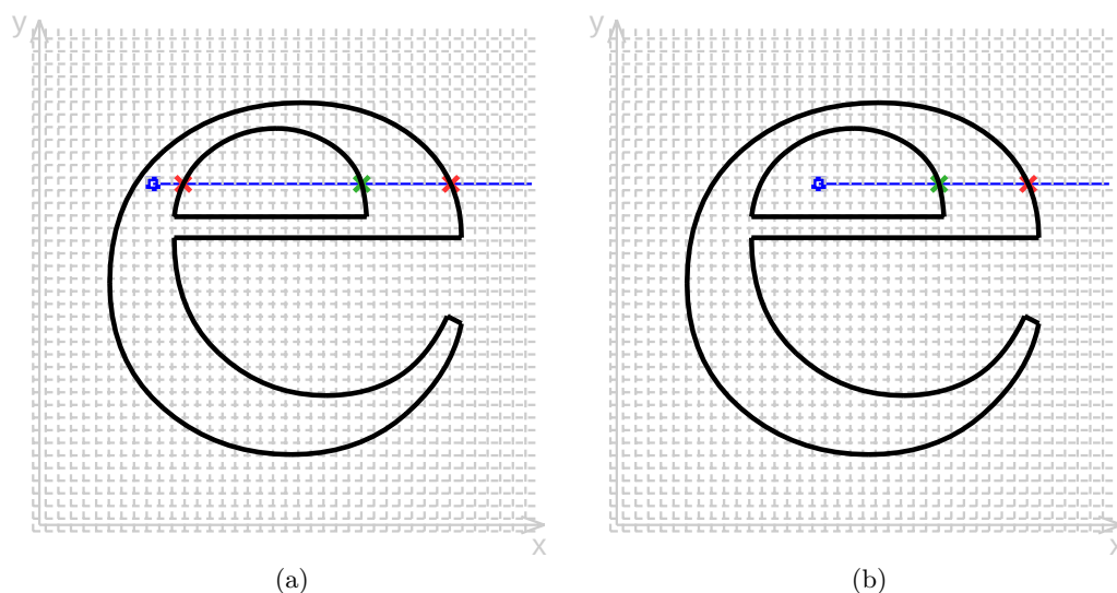
Slika 7.14: Postupak popunjavanja unutrašnjosti slova.
