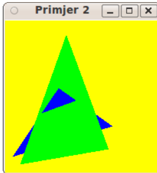
Slika 8.12: Watkinsov postupak: trokuti koji se probadaju
