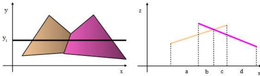
Slika 8.7: Linija pretrage (lijevo) i rasponi uzorka (desno) u postupku Watkinsa
