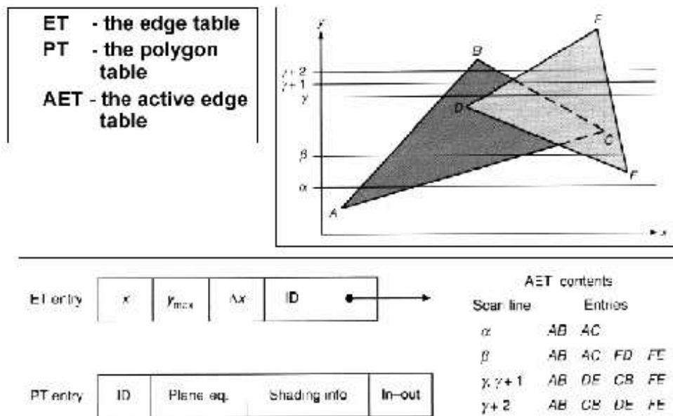
Slika 8.8: Podatkovne strukture u postupku Watkinsa
