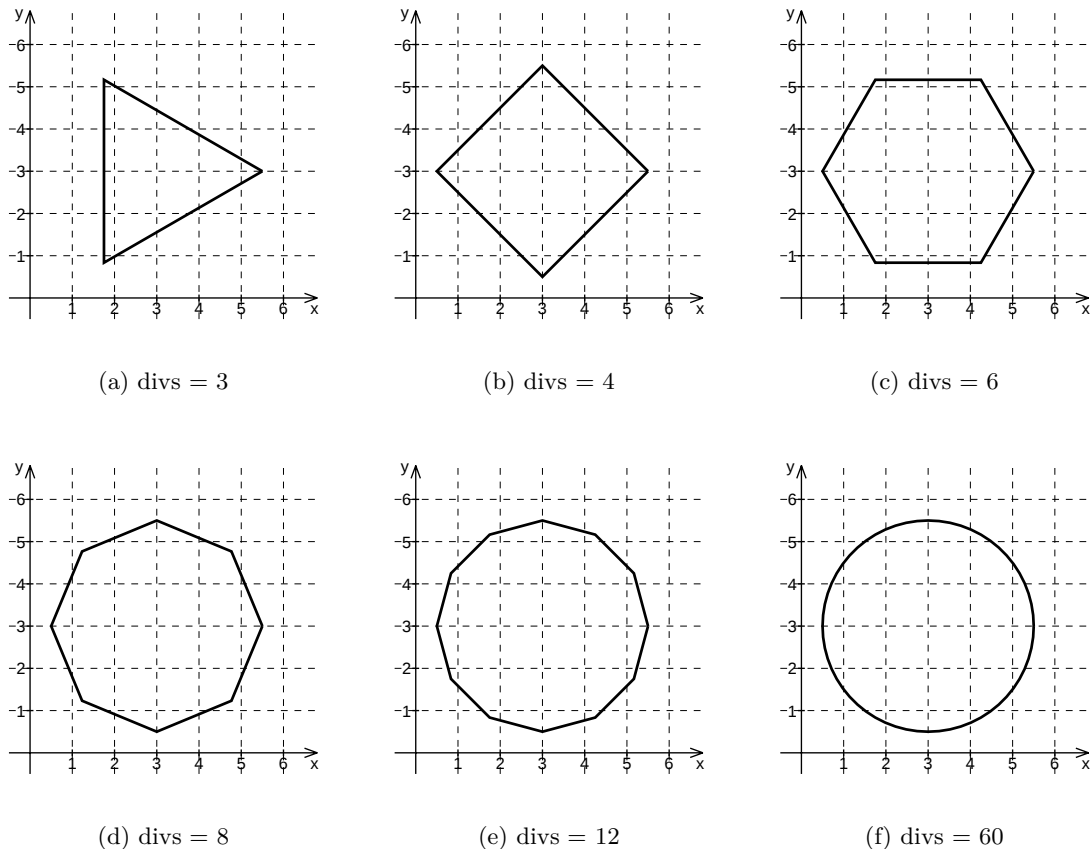
Slika 7.3: Utjecaj broja točaka na prikaz kružnice.
