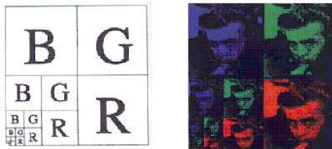
Slika 12.8: Efikasno pohranjivanje Mip-Map tekstura.
