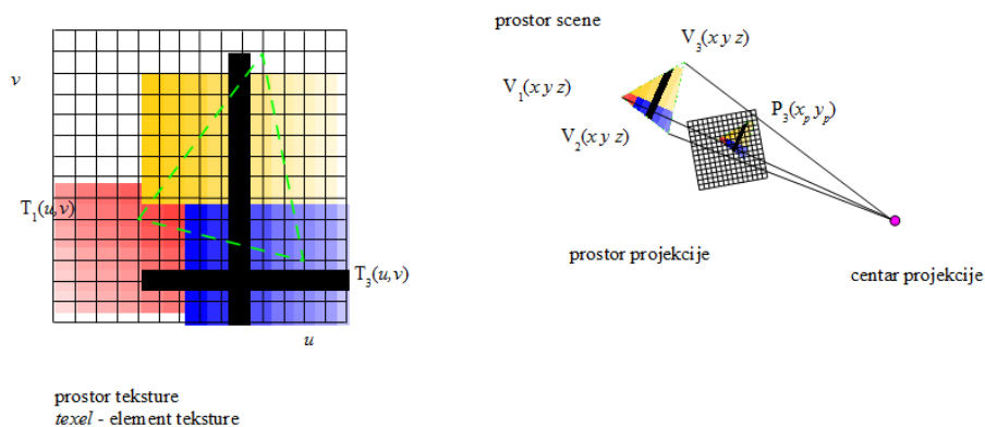
Slika 12.3: Preslikavanje tekture na trokut.
