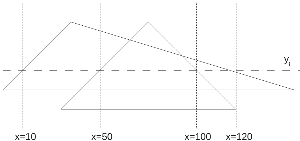
Slika 8.10: Watkinsov postupak: preklapajući trokuti
