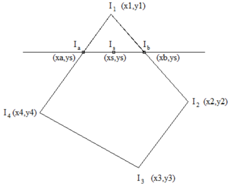
Slika 9.10: Interpolacija intenziteta kod Gouraudovog sjenčanja
