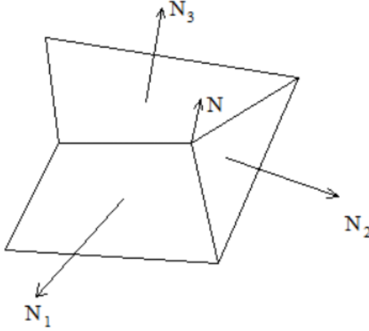
Slika 9.9: Izračun srednje normalne u vrh tijela
