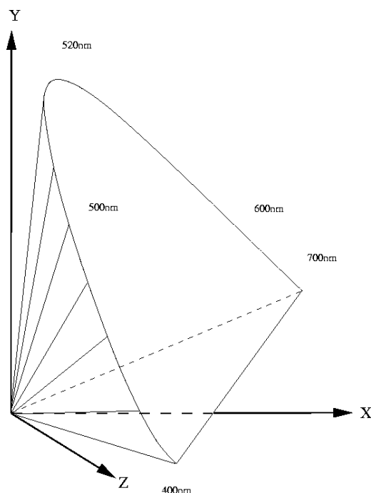
Slika 11.7: Komponente XYZ potrebne za prikaz svih boja
