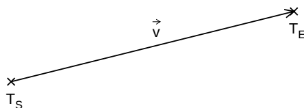
Slika 2.1: Vektor između dviju točaka
