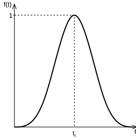
Slika 7.4: Primjer težinske funkcije zvonolikog oblika
