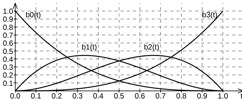
Slika 3.8: Dobivene kubne bazne funkcije.
