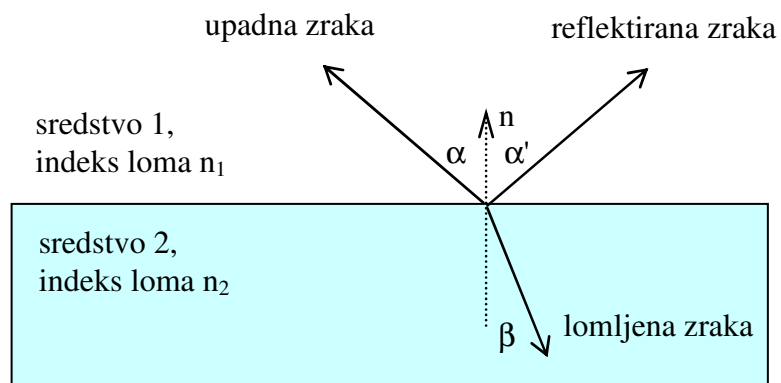
Slika 9.1: Refleksija i refrakcija svjetlosti na površini.
