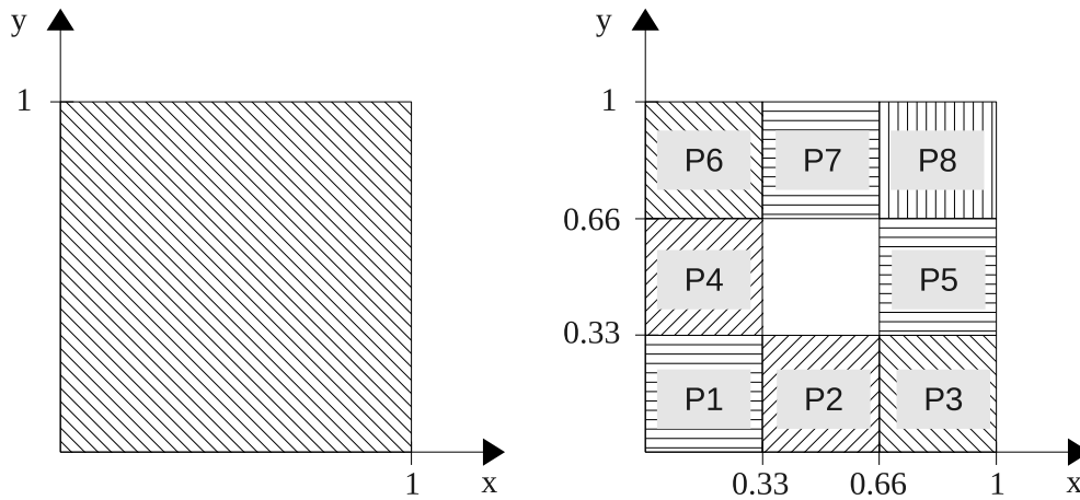
Slika 13.17: Konstrukcija ITS fraktala
