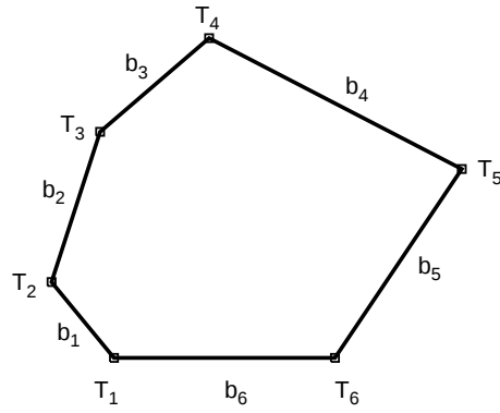
Slika 4.3: Poligon
