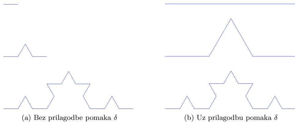
Slika 13.20: Kochina krivulja generirana L-sustavom
