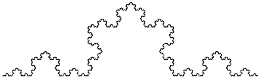
Slika 13.3: Kochina krivulja – rezultat uz dubinu rekurzije 6
