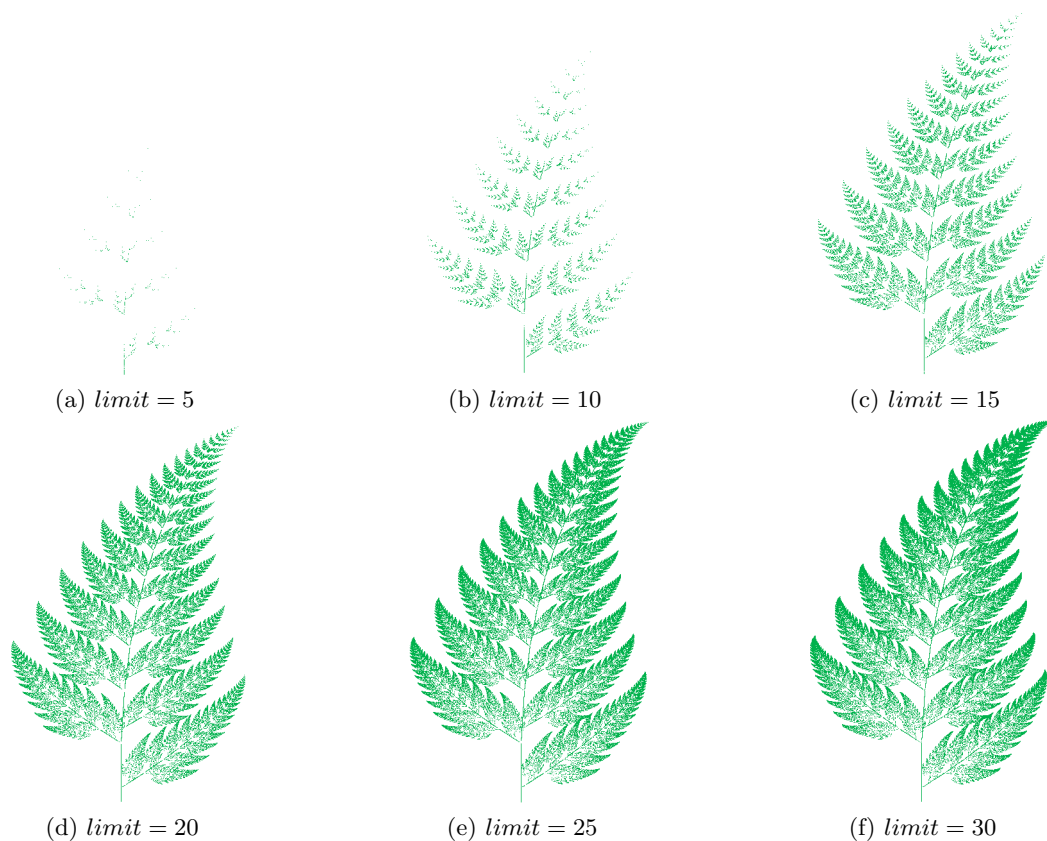
Slika 13.15: Primjeri lista paprati generiranog ITS-om
