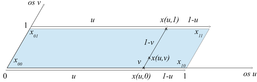
Slika 3.10: Izvod bilinearne interpolacije.
