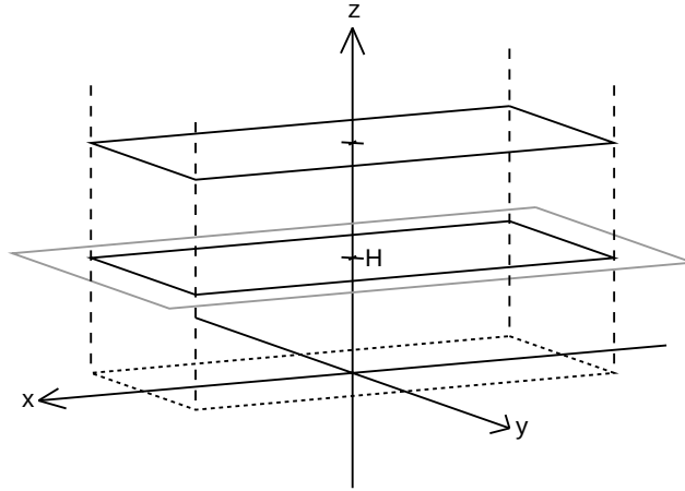
Slika 6.1: Paralelna projekcija
