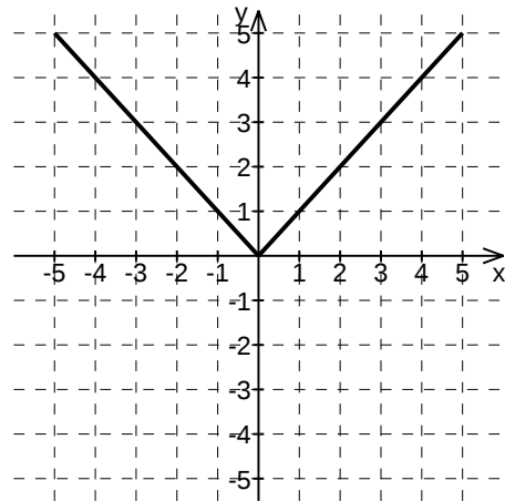
(b) Ima C^0 ali nema C^1
