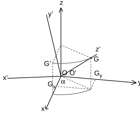
Slika 6.9: Rotacija oko z -osi
