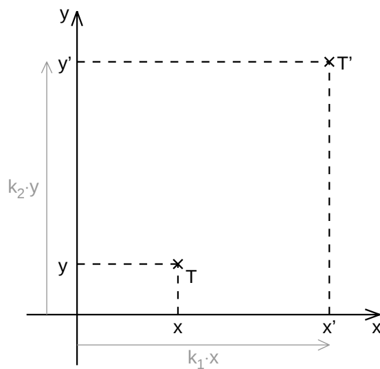
Slika 5.4: Skaliranje točke
