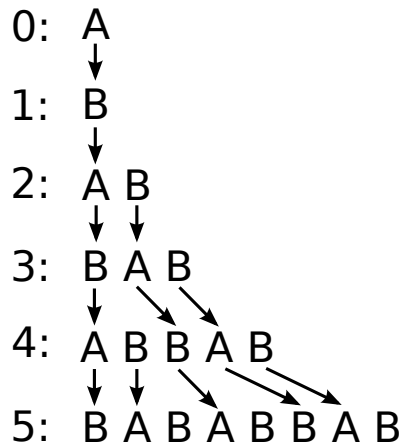
Slika 13.19: L-sustav za Fibonaccijeve brojeve
