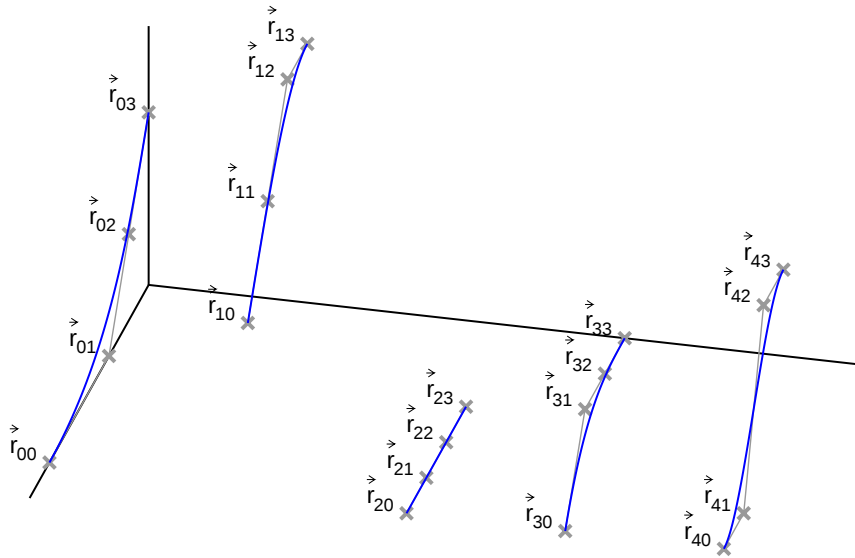
Slika 7.17: 5 aproksimacijskih Bezierovih krivulja
