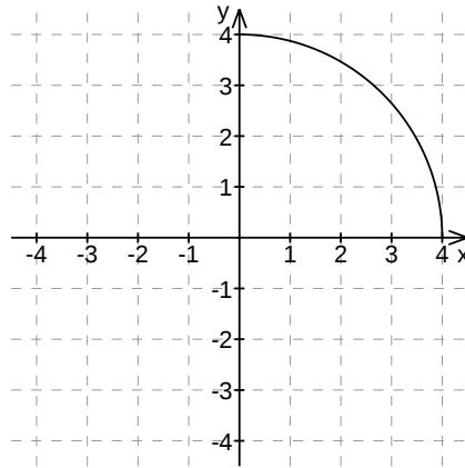
Slika 7.9: Segment kružnice.
