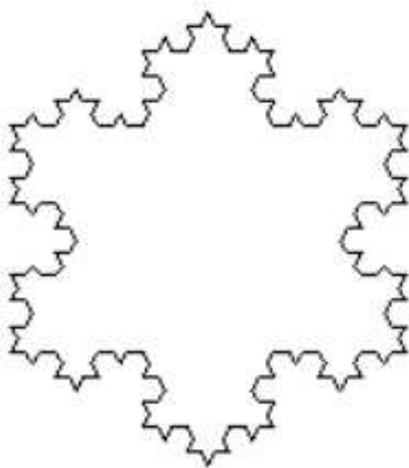
Slika 13.6: Kochina pahuljica - kraj
