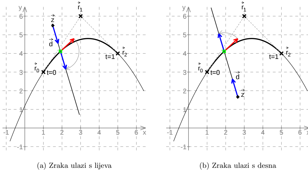
Slika B.5: Različite orijentacije sjecišta.
