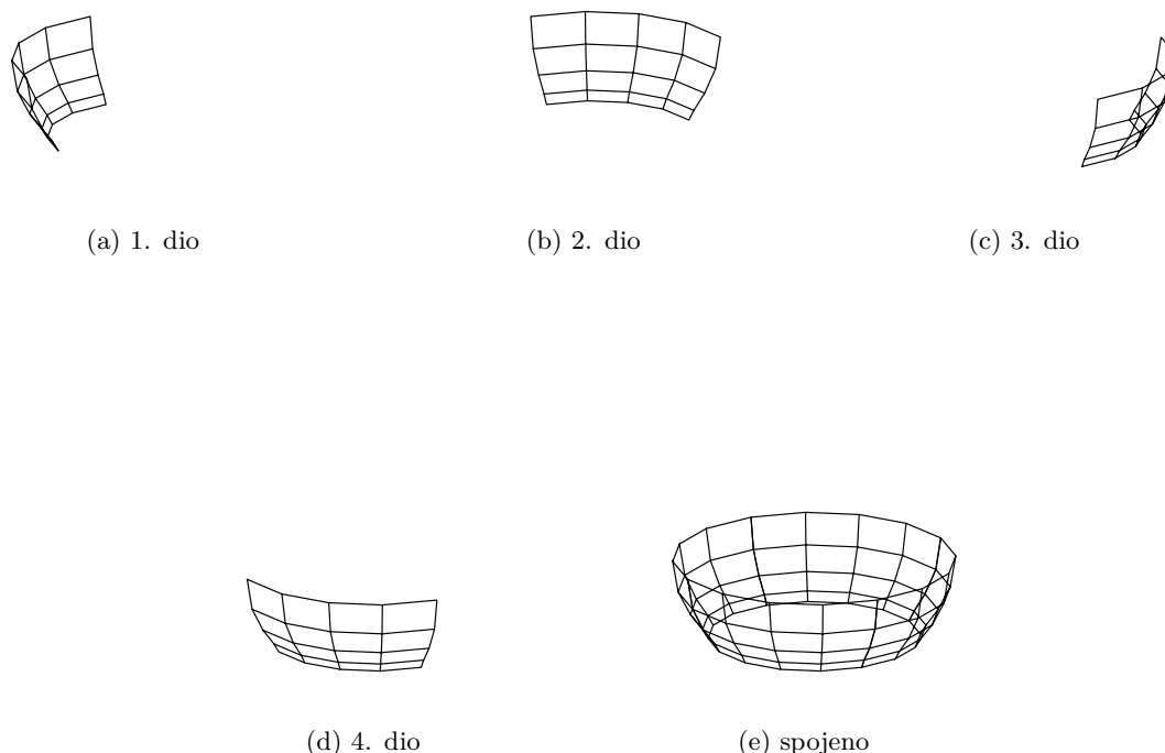
Slika 7.20: Dio oplošja čajnika izrađen od četiri Bezierove površine.
