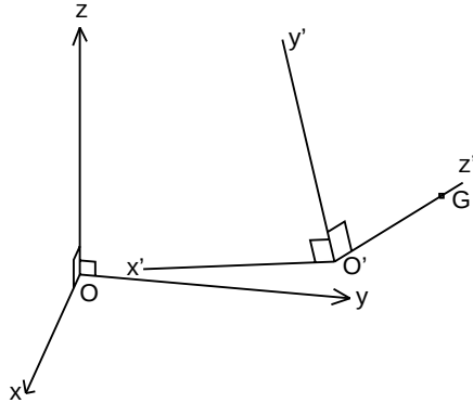
Slika 6.6: Dva koordinatna sustava
