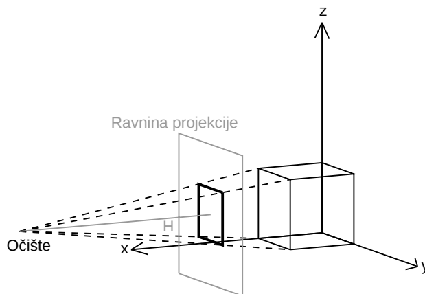
Slika 6.3: Perspektivna projekcija
