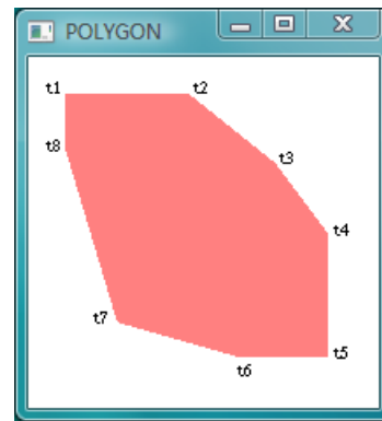
Slika 1.11: primitiv GL_POLYGON
