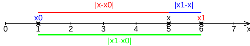
Slika 3.1: Linearna interpolacija i baricentrične koordinate
