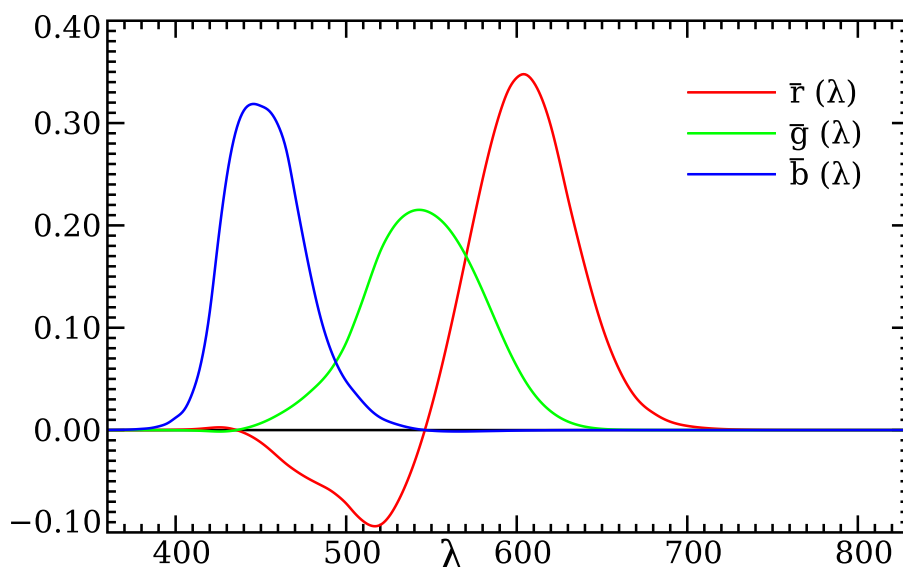
Slika 11.6: Komponente RGB potrebne za prikaz svih boja
