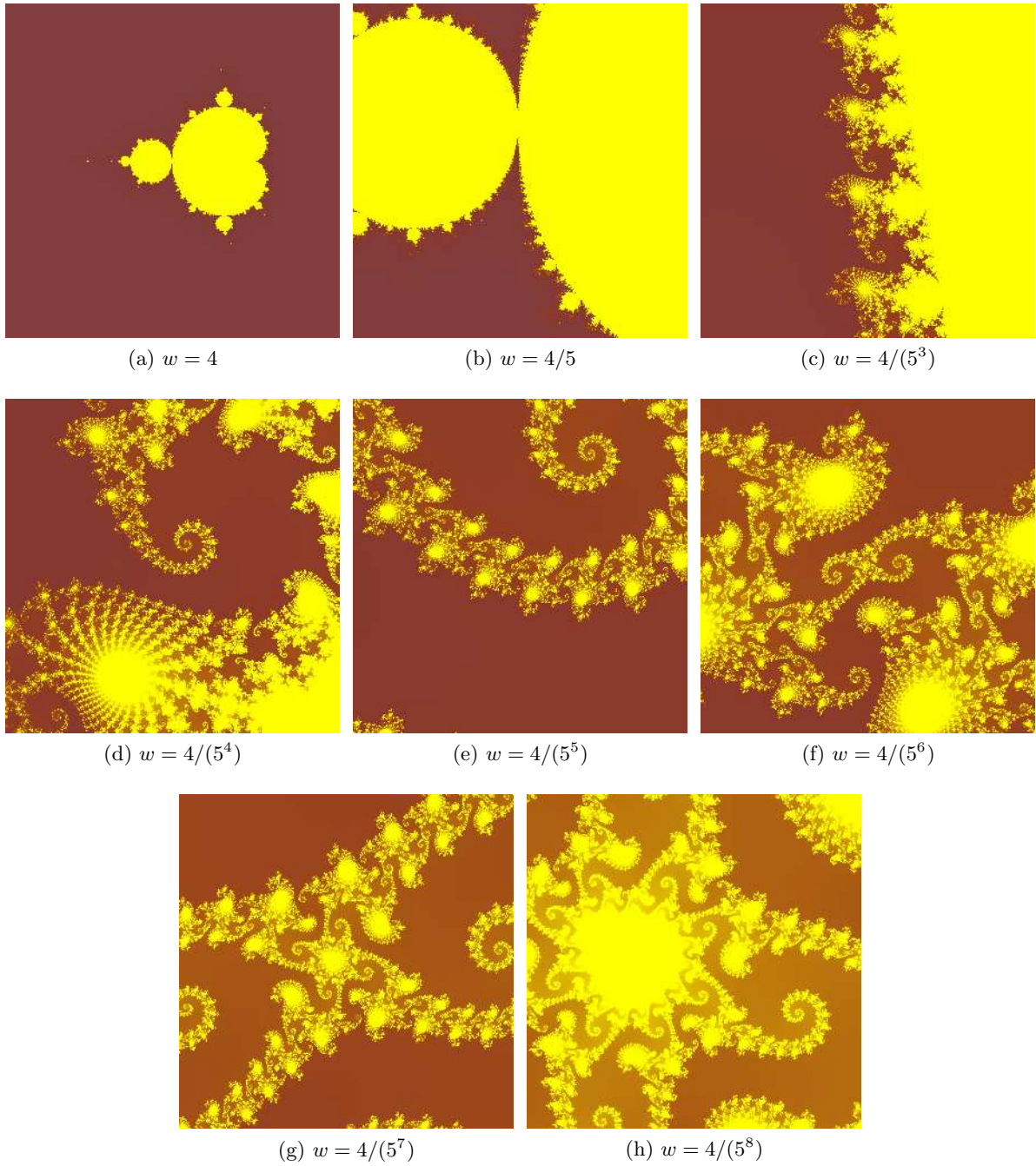
Slika 13.11: Mandelbrotov fraktal uz različita uvećanja
