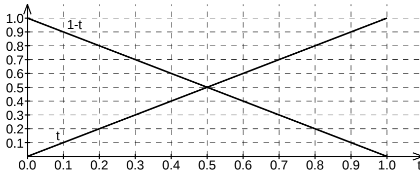
Slika 3.2: Težinske funkcije kod linearne interpolacije
