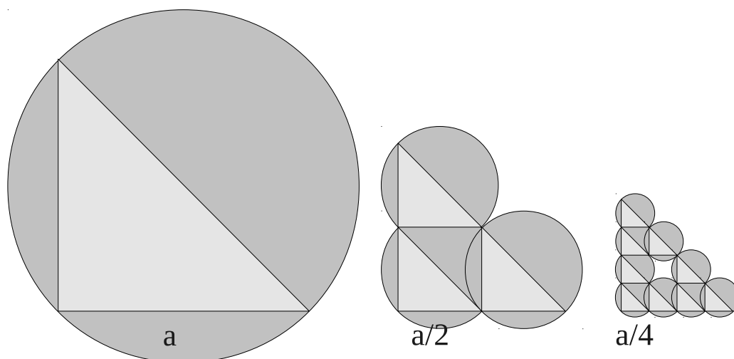
Slika 13.29: Određivanje Hausdorffove dimenzije trokuta Sierpinskog
