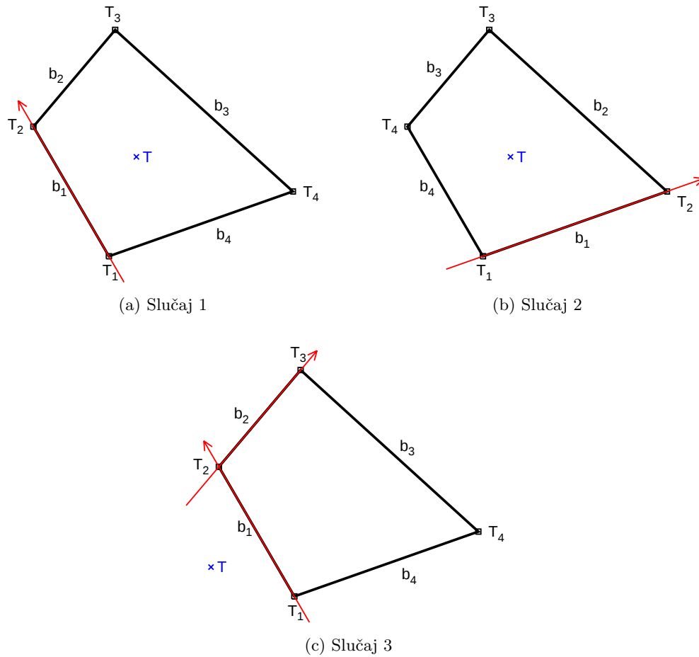
Slika 4.6: Odnos točke i poligona
