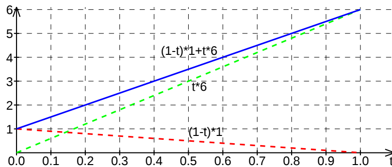
Slika 3.3: Linearna interpolacija razložena na sastavne dijelove
