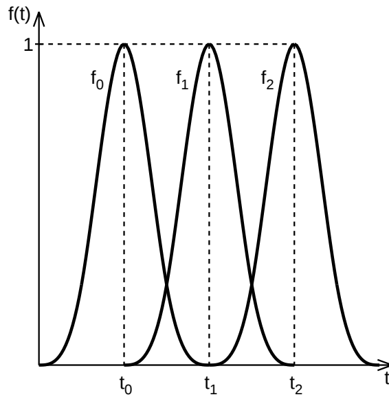
Slika 7.5: Težinske funkcije uz tri točke krivulje
