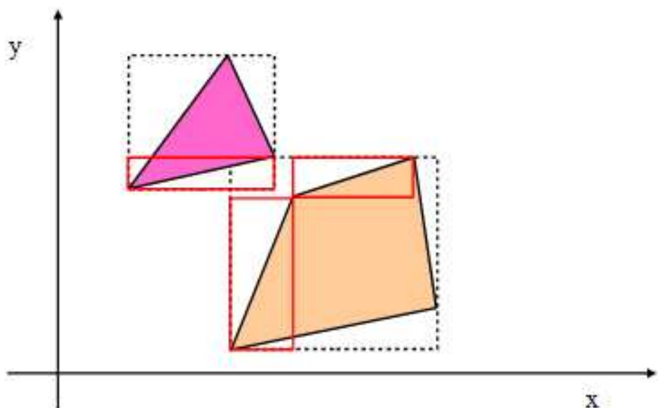
Slika 8.6: Poligoni se potencijalno preklapaju, ali niti jedan brid prvog objekta sigurno se ne preklapa s niti jednim bridom drugog objekta
