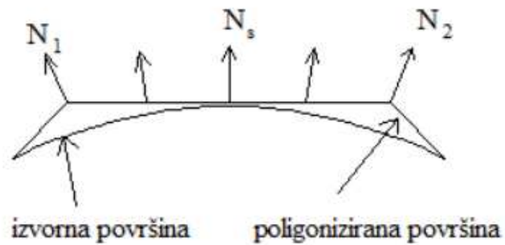
Slika 9.11: Interpolacija normala kod Phongovog sjenčanja
