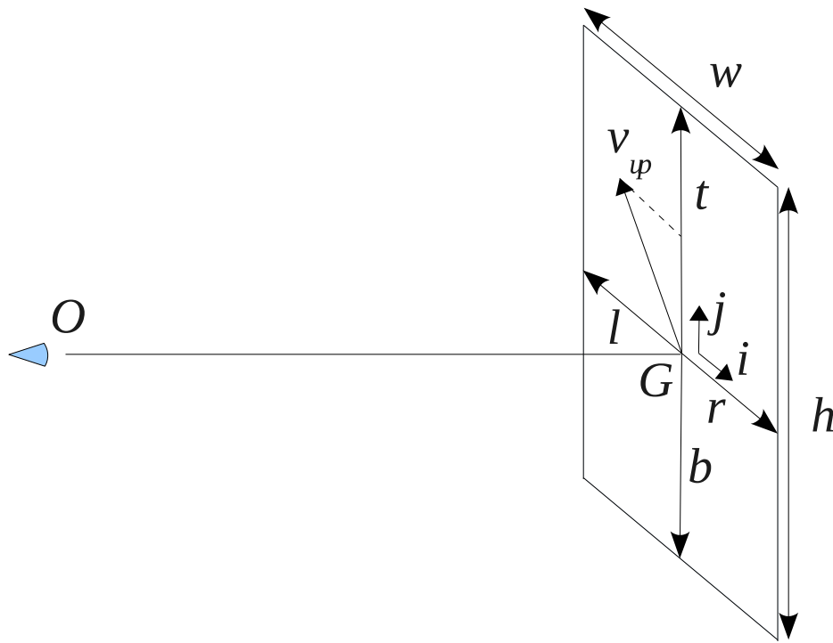
Slika 10.2: Definiranje ravnine ekrana
