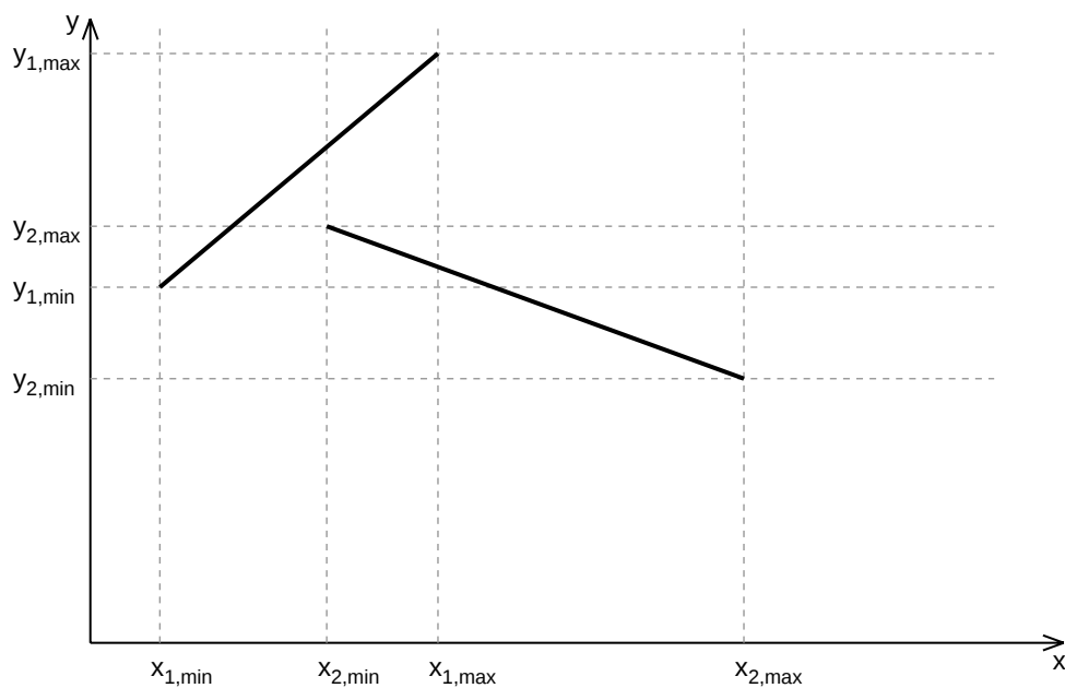
Slika 8.5: Primjer kada se dvije dužine potencijalno preklapaju
