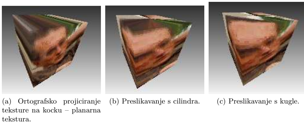
Slika 12.15: Projekcijska planarna tekstura.
