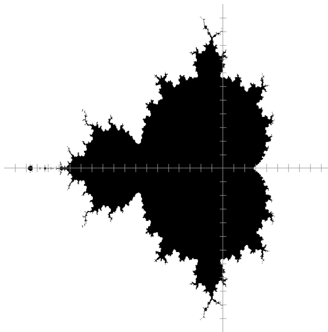
Slika 13.9: Mandelbrotov skup
