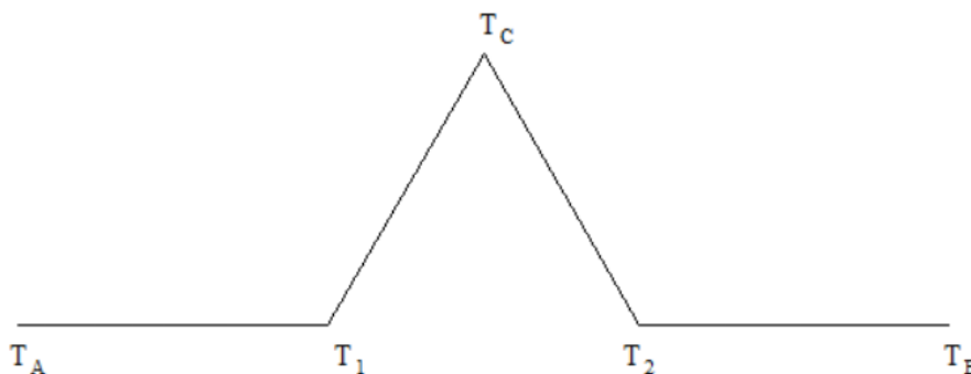
Slika 13.1: Kochina krivulja – početak konstrukcije
