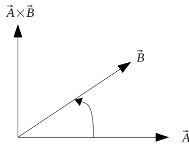
Slika 2.3: Vektorski produkt
