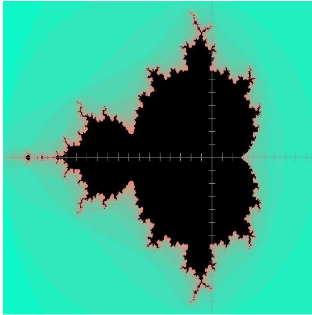
Slika 13.10: Mandelbrotov skup uz bojanje prema brzini divergencije
