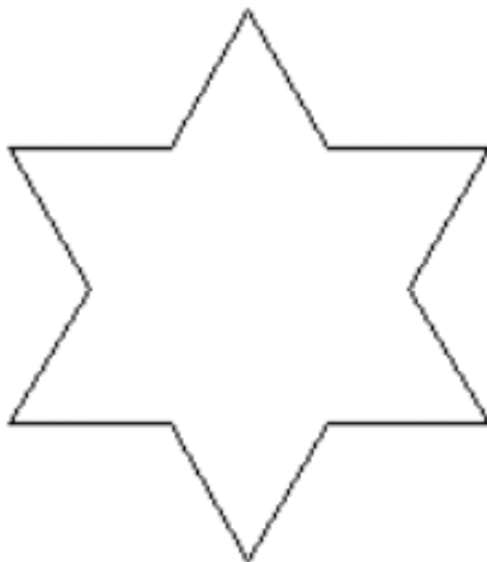
Slika 13.4: Kochina pahuljica - početak
