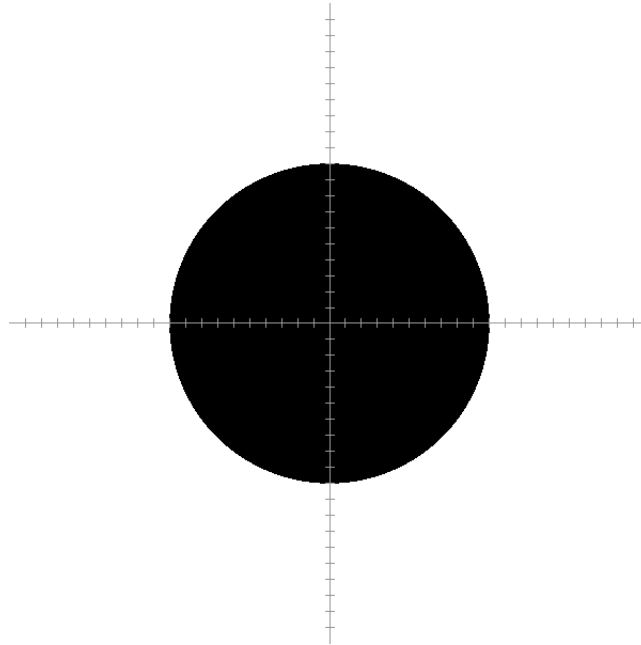
Slika 13.12: Julijev skup za funkciju z_{n+1} = z_n^2
