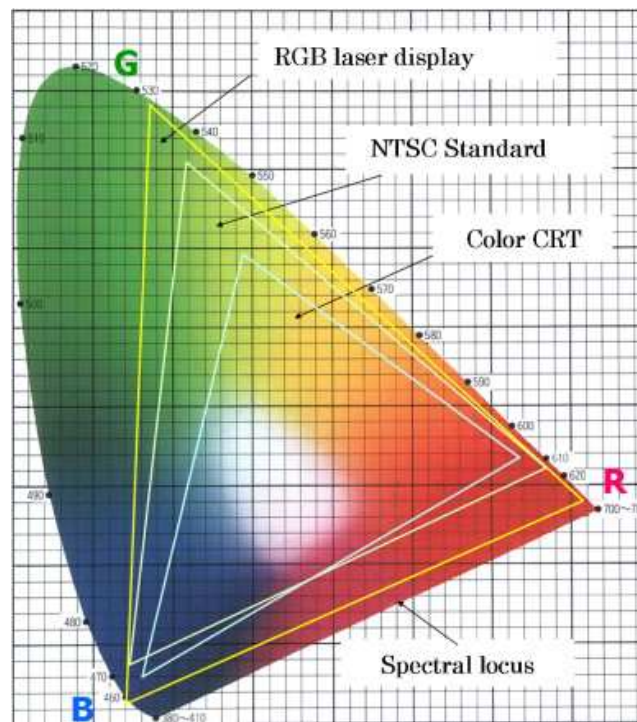
Slika 11.10: GAMUT uređaja
