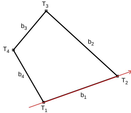
Slika 4.5: Orijentacija vrhova poligona – u smjeru suprotnom od smjera kazaljke na satu. Vrh T_3 je iznad brida b_1 .
