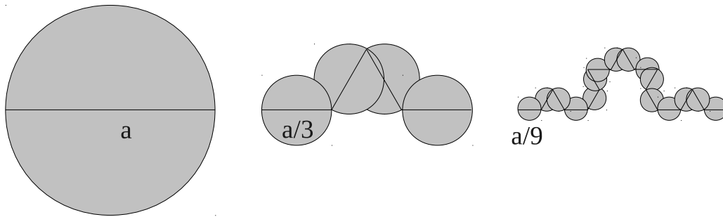
Slika 13.28: Određivanje Hausdorffove dimenzije Kochine krivulje
