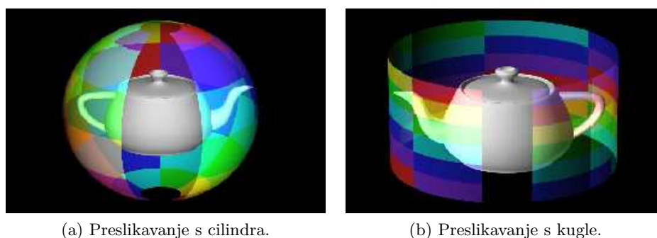
Slika 12.16: Preslikavanje tekstuure.
