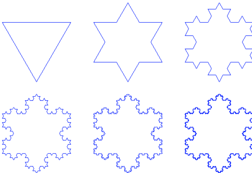
Slika 13.21: Kochina pahuljica generirana L-sustavom
