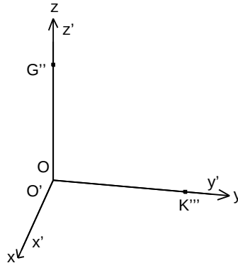
Slika 6.16: Poklopljeni sustavi
