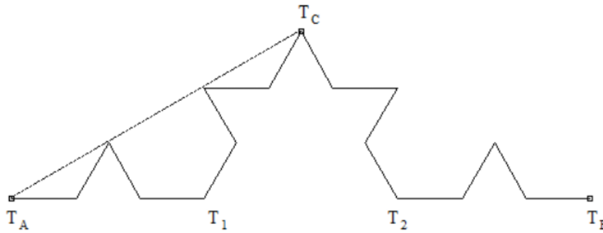
Slika 13.2: Kochina krivulja – drugi korak rekurzije
