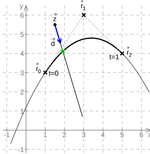
Slika B.4: Utvrđivanje sjecišta zrake i kvadratne aproksimacijske Bezierove krivulje
