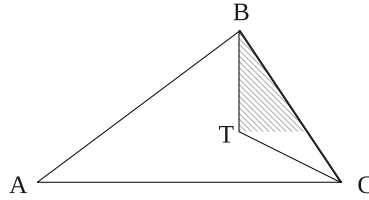
Slika 2.8: Baricentrične koordinate preko omjera površina trokuta
