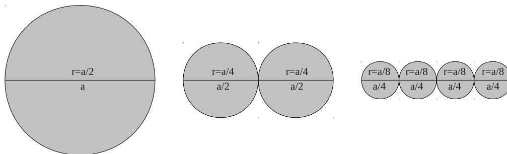
Slika 13.26: Određivanje Hausdorffove dimenzije segmenta linije
