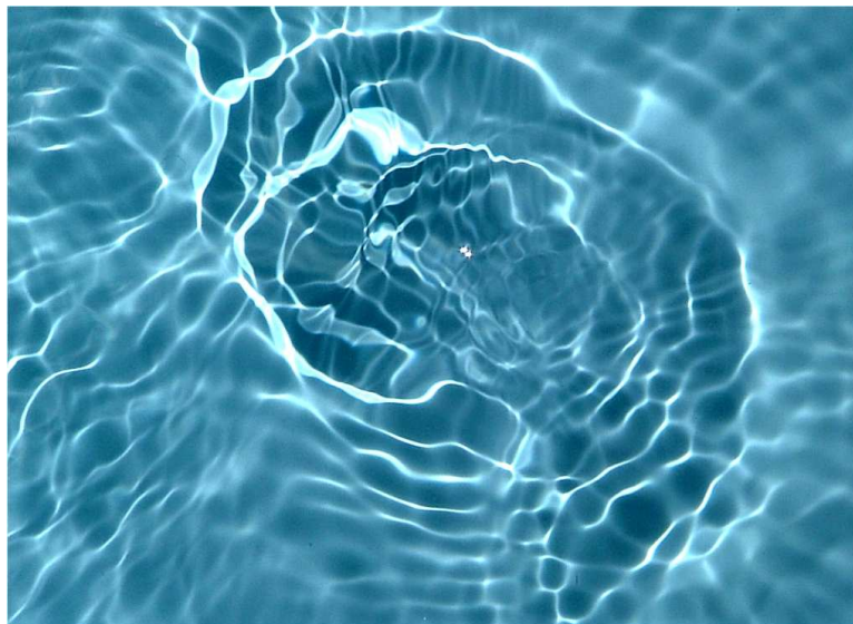
Slika 9.2: Primjer učinka kaustike na površini vode.
