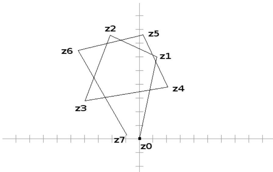
Slika 13.7: Ispitivanje pripadnosti točke Mandelbrotovom skupu
