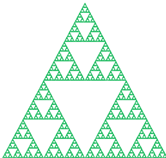
Slika 13.16: Trokut Sierpinskog
