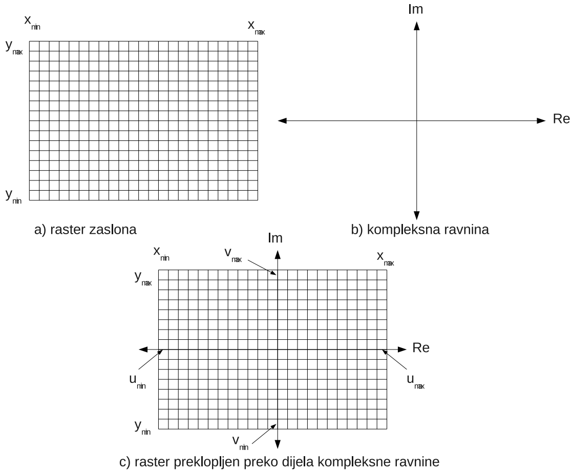
Slika 13.8: Crtanje Mandelbrotovog skupa
