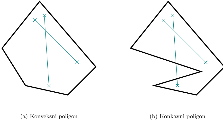
Slika 4.2: Razlika između konveksnog i konkavnog poligona
