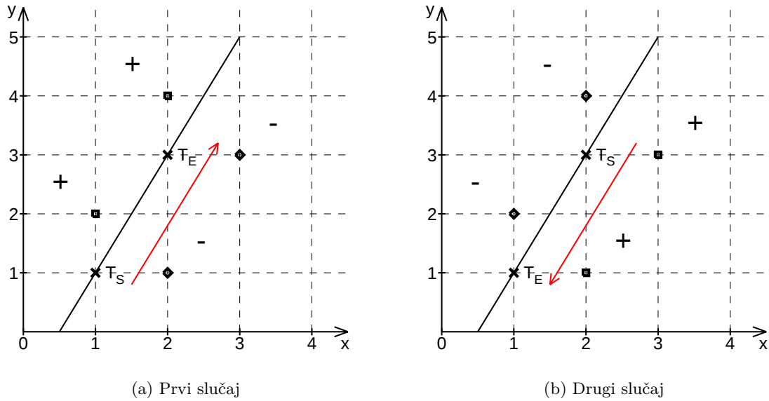
Slika 2.5: Odnos točke i pravca
