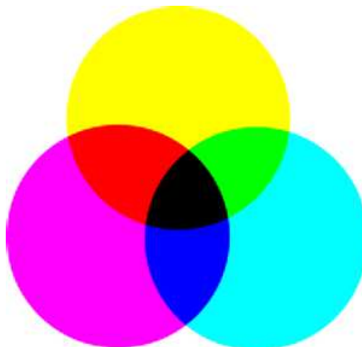
Slika 11.11: CMY-model boja
