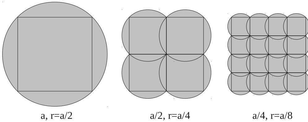
Slika 13.27: Određivanje Hausdorffove dimenzije segmenta kvadrata
