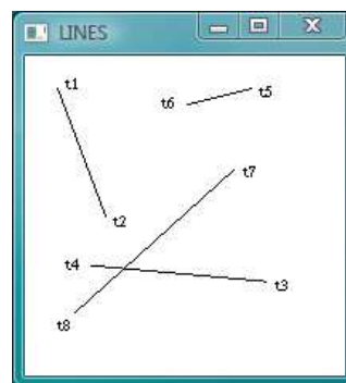
Slika 1.3: primitiv GL_LINES
