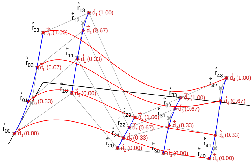
Slika 7.18: 4 aproksimacijske Bezierove krivulje čiji su kontrolni poligoni definirani točkama na aproksimacijskim Bezierovim krivuljama
