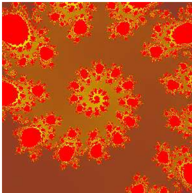
(d) c.re = -0.500036 , c.im = -0.520156
