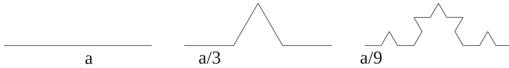
Slika 13.23: Opseg Kochine krivulje
