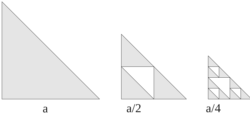
Slika 13.24: Površina i opseg trokuta Sierpinskog
