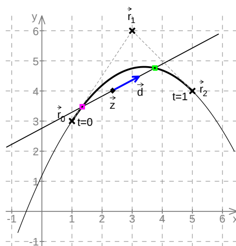
(e) Jedno sjecište
