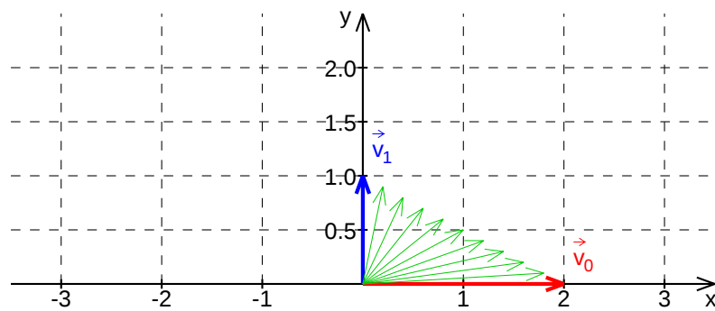
(b) Interpolacija između vektora (2, 0) i (0, 1)
