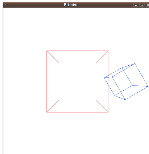
Slika 6.19: Dvije kocke
