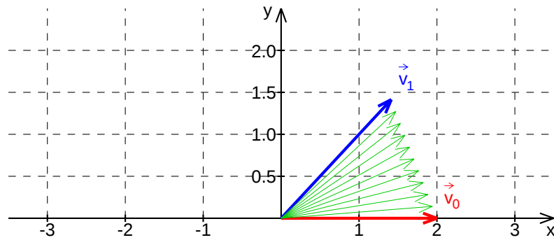
(a) Interpolacija između vektora (2, 0) i (\sqrt{2}, \sqrt{2})
