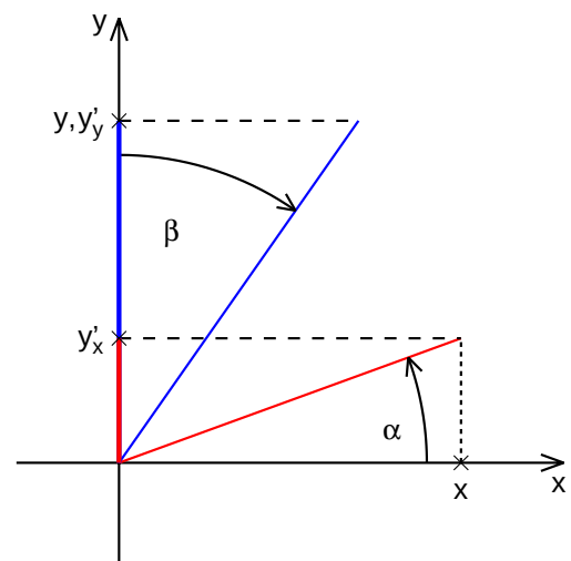
(b) Utjecaj smika na komponentu y
