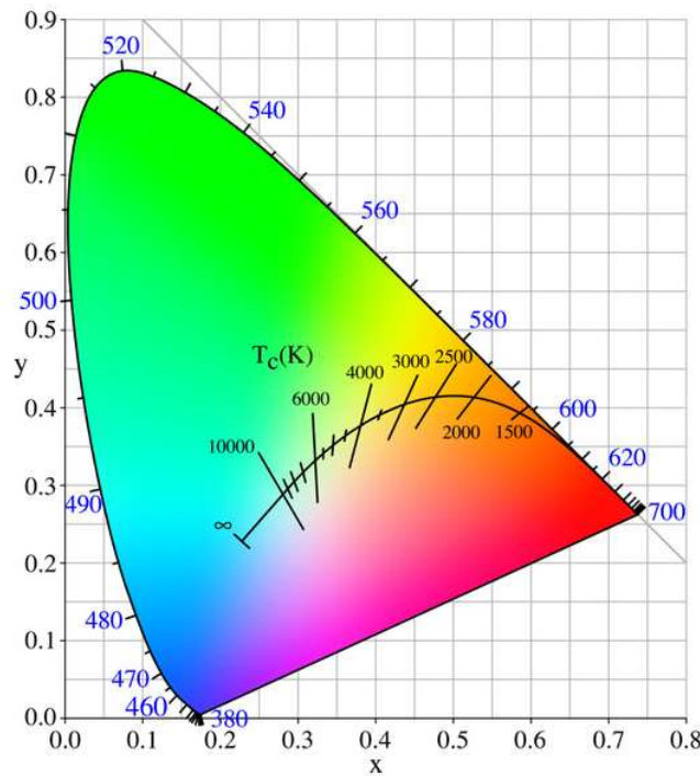
Slika 11.8: Dijagram kromatičnosti
