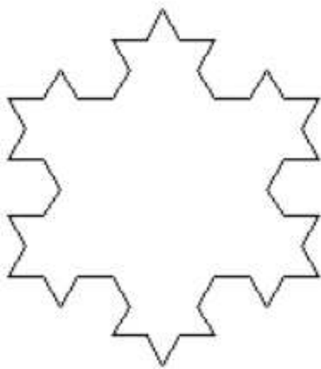
Slika 13.5: Kochina pahuljica - drugi korak rekurzije
