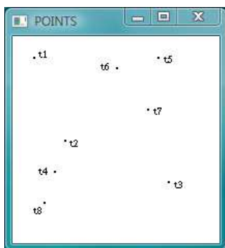
Slika 1.2: primitiv GL_POINT
