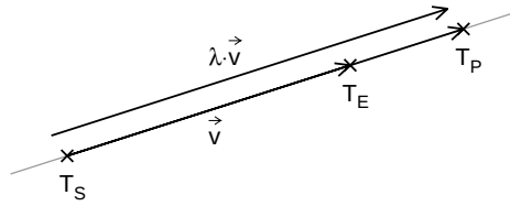
Slika 2.4: Pravac dobiven skaliranjem vektora
