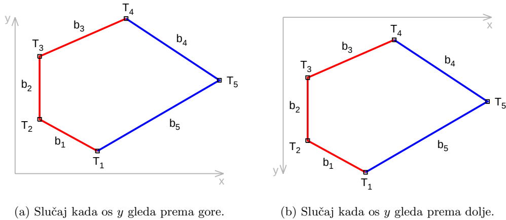
Slika 4.7: Podjela bridova na lijeve i desne kod konveksnog poligona. Crvenom bojom su prikazani lijevi bridovi a plavom desni.
