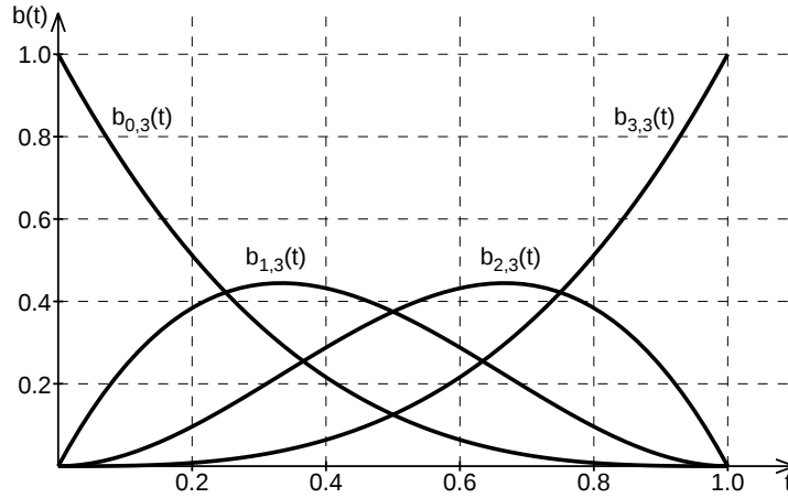
Slika 7.7: Bernsteinove težinske funkcije za Bezierovu krivulju trećeg stupnja
