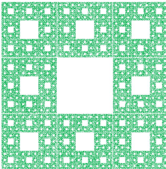
Slika 13.18: Rezultat konstrukcije ITS fraktala – tepih Sierpinskog
