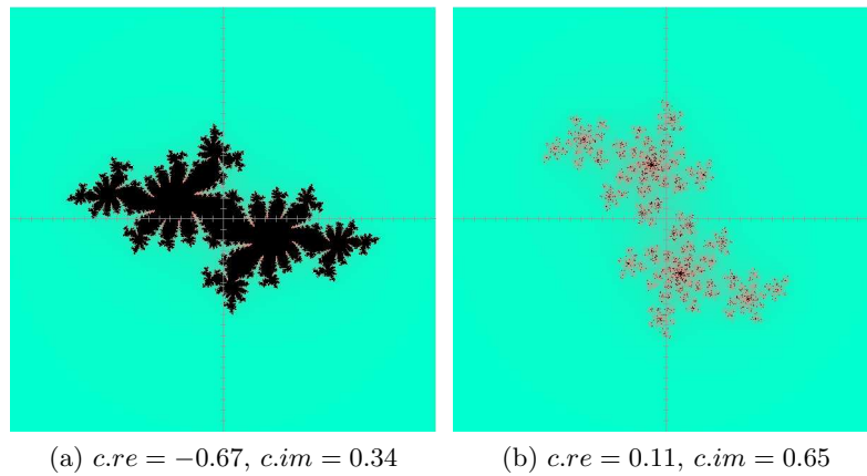
Slika 13.13: Povezan i nepovezan Julijev skup
