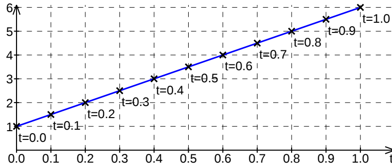
Slika 3.4: Razdioba vrijednosti kod linearne interpolacije
