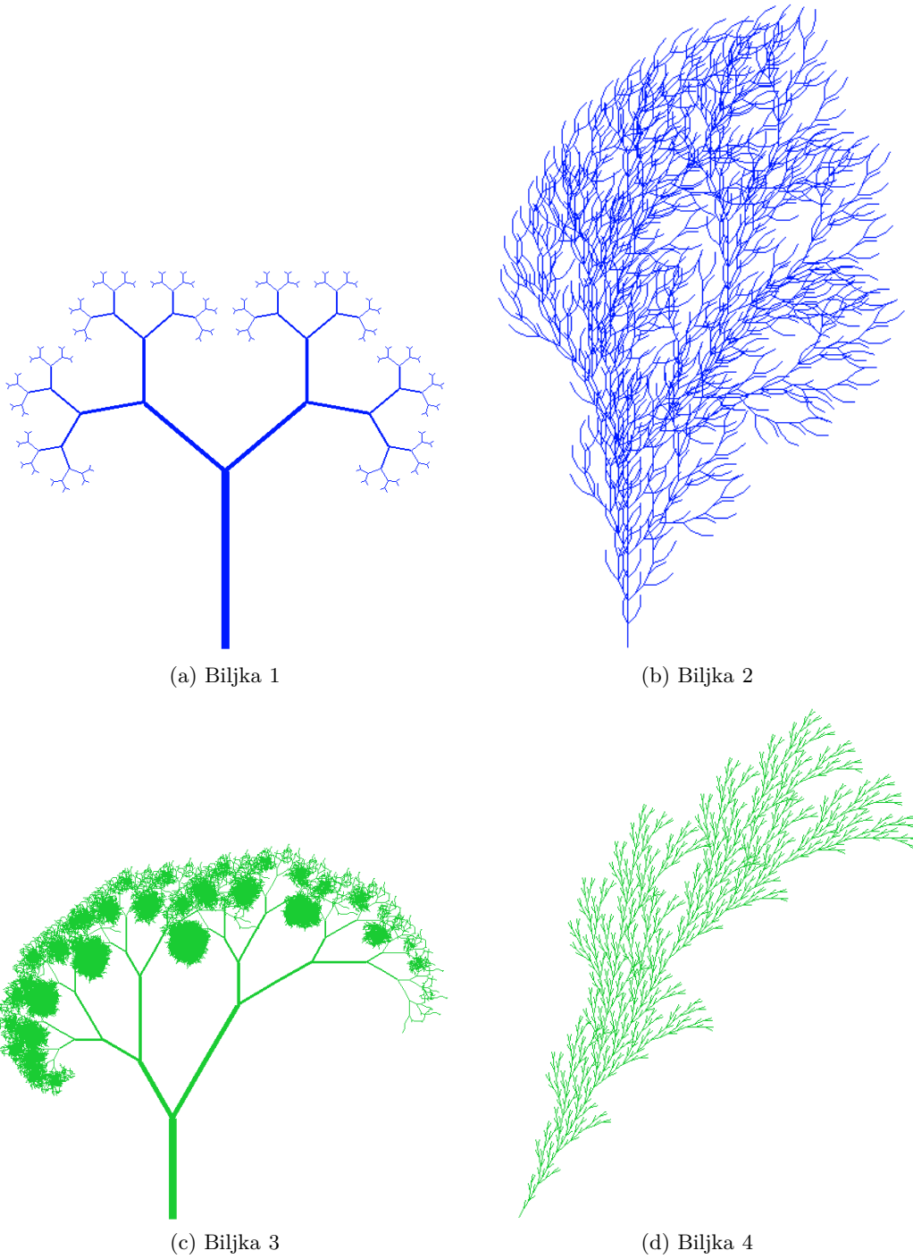
Slika 13.22: L-sustavom s grananjem
