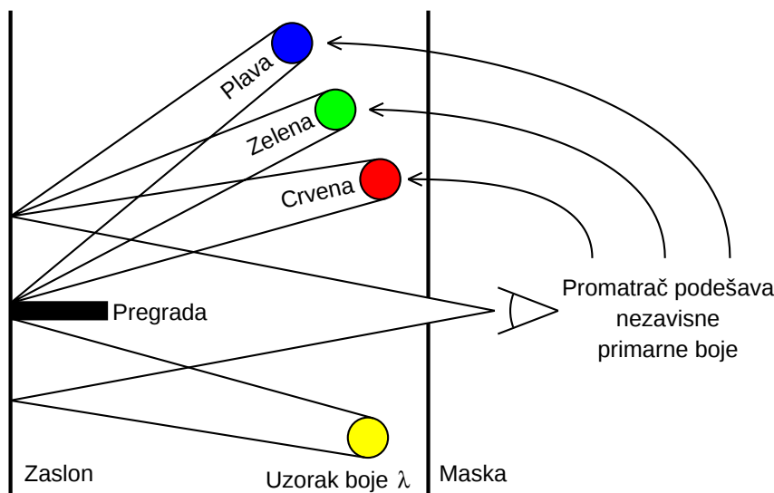
Slika 11.5: Pokus podudaranja ispitnog uzorka boje
