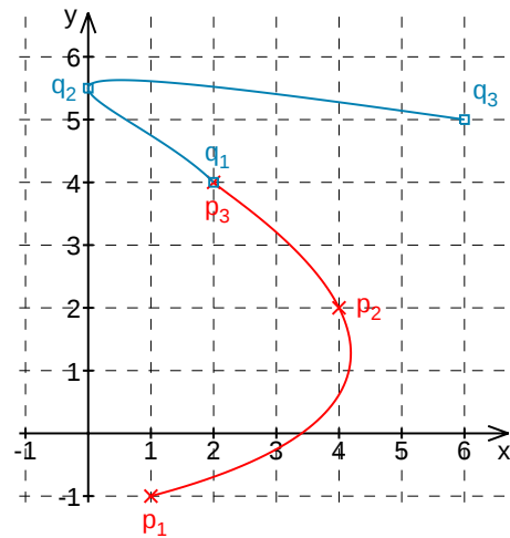
(d) Ima G^0 i G^1 ali nema C^1
