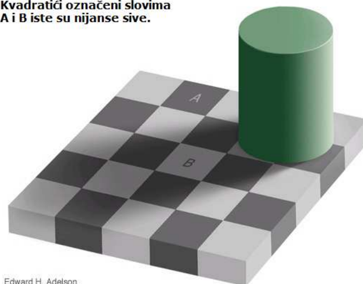
Slika 11.2: Kvadratići iste nijanse sive.
