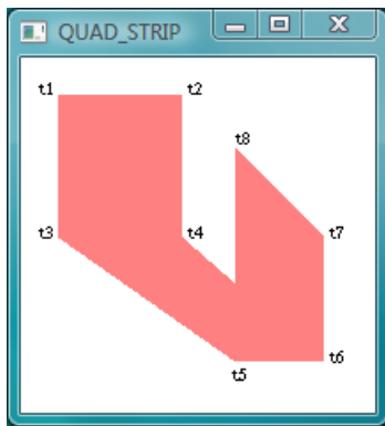
Slika 1.10: primitiv GL_QUAD_STRIP
