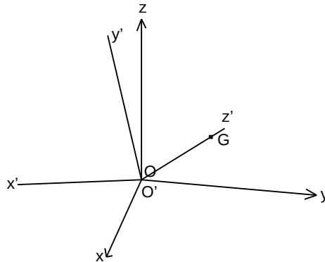
Slika 6.8: Dva koordinatna sustava nakon primjene transformacije \Theta_1
