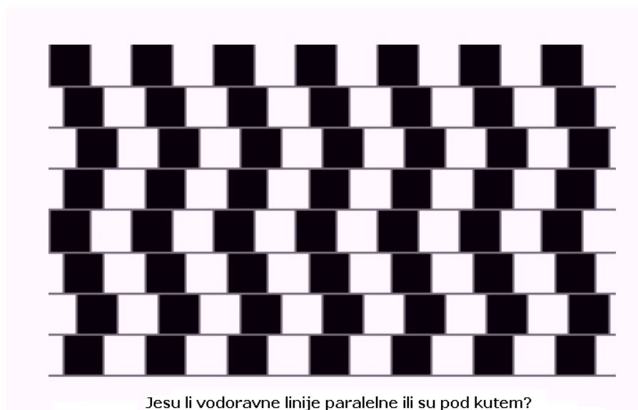
Slika 11.1: Paralelne linije?
