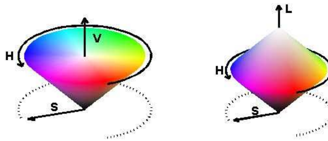
Slika 11.12: HSV i HSL prostori boja
