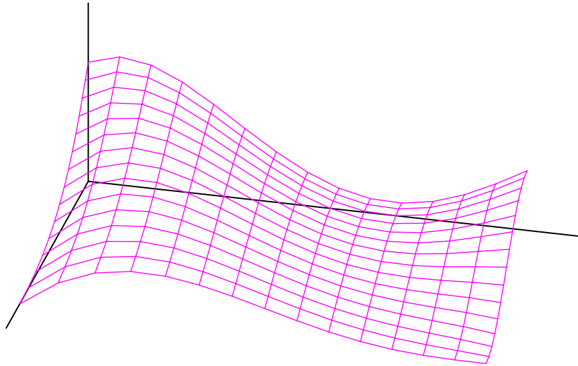
Slika 7.19: Prikaz Bezierove površine diskretnim krpicama
