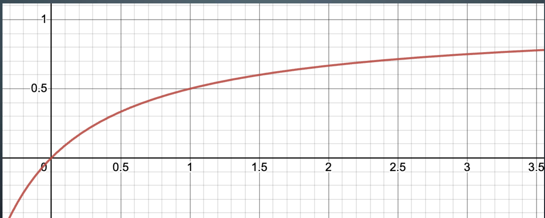
Slika 5. Dodatna isplatna funkcija za a = 1
