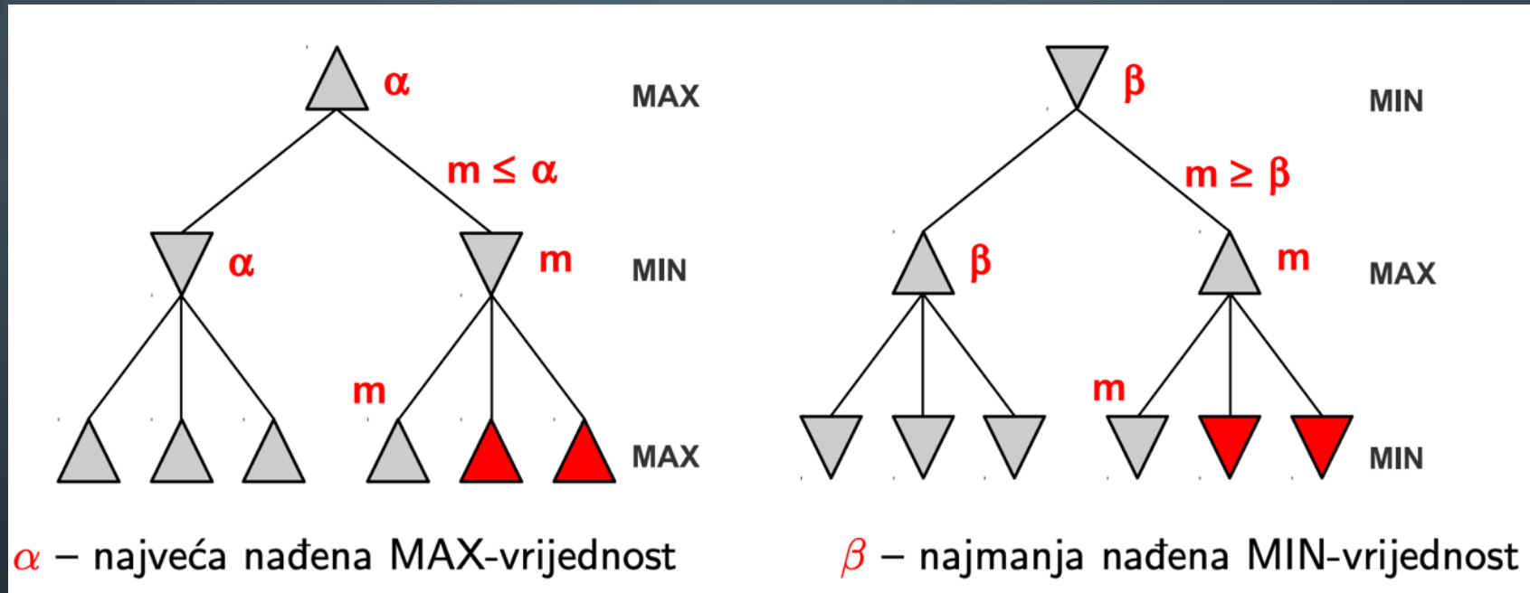
Slika 6. Prikaz alfa-beta podrezivanja [4]
