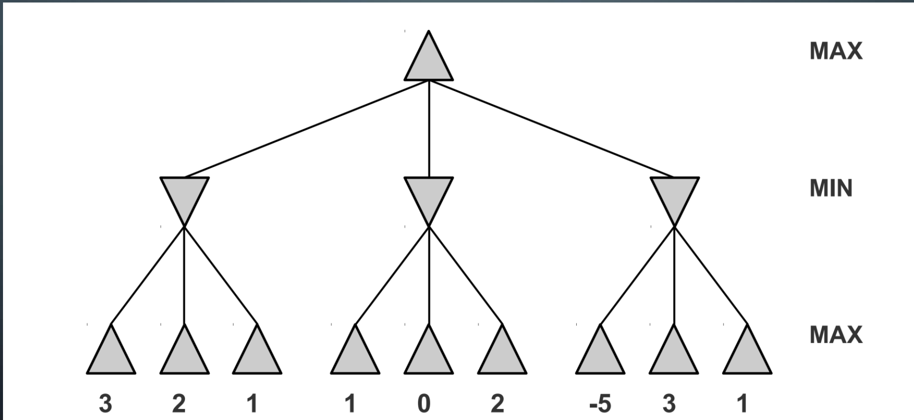
Slika 4. Metoda minimaks [4]
