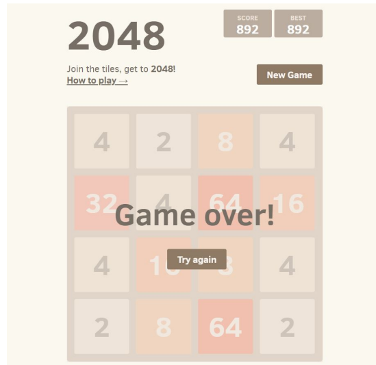
Slika 2.3: Kraj igre [1]
