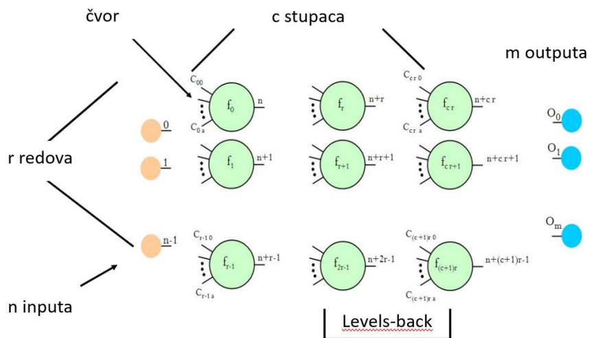
Slika 4.1: CGP mreža [6]
