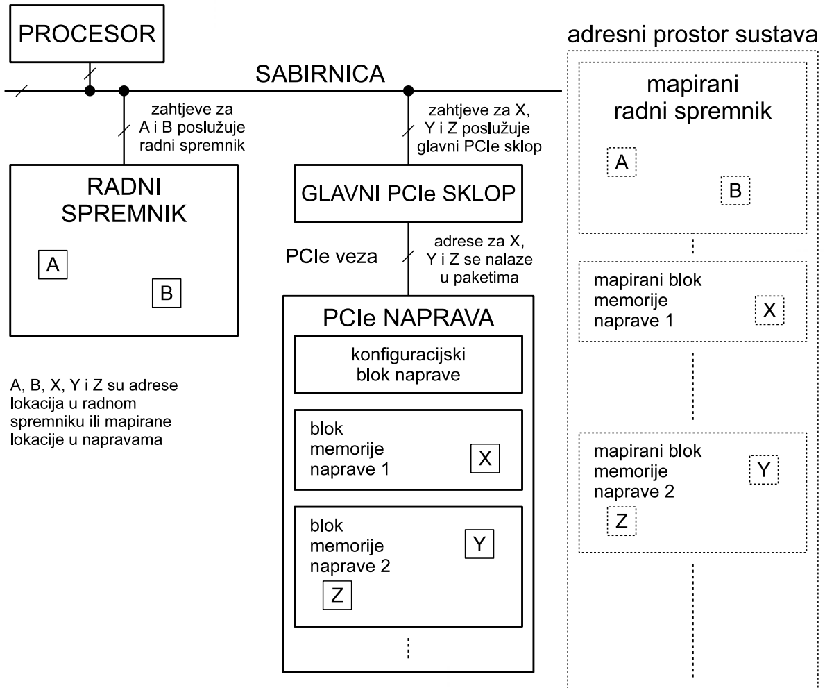
Slika 4.13. Primjer sustava s jednom PCIe napravom
