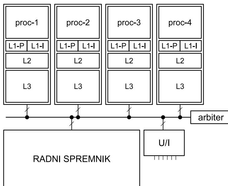
Slika 7.1. Primjer simetričnog višeprocessorskog sustava
