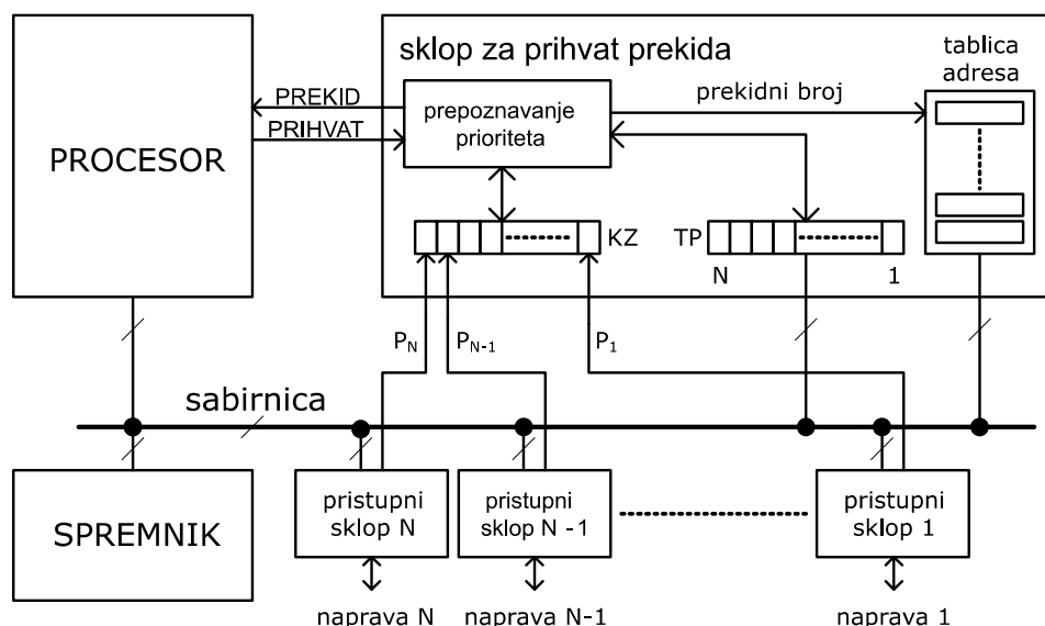
Slika 2.1. Procesor sa sklopom za prihvatanje prekida
