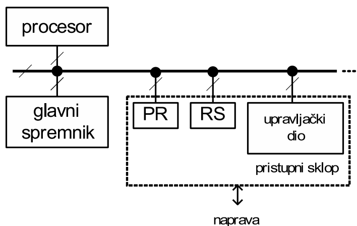
Slika 3.1. Jednostavni model pristupnog sklopa UI naprave
