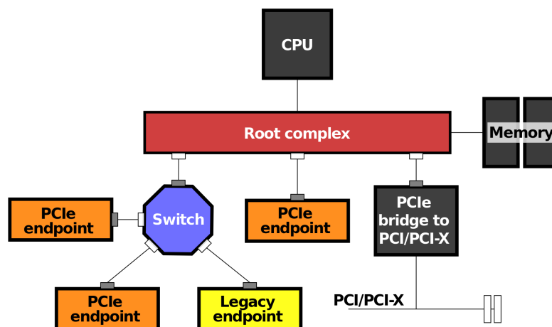
Slika 4.10. Primjer povezivanja naprava na PCIe (slika s Wikipedije)
