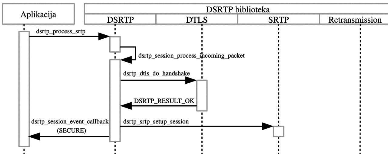
Slika 5.5: Završetak DTLS dogovaranja i uspostavljanje SRTP sjednice - sekvencijski dijagram
