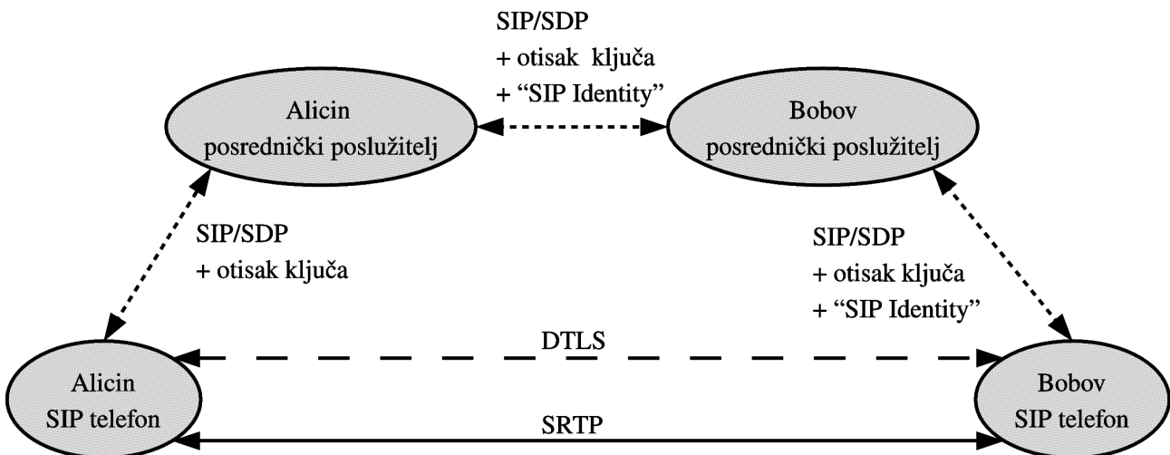
Slika 4.3: SIP trapezoid kada se DTLS-SRTP koristi za zaštitu RTP prometa
