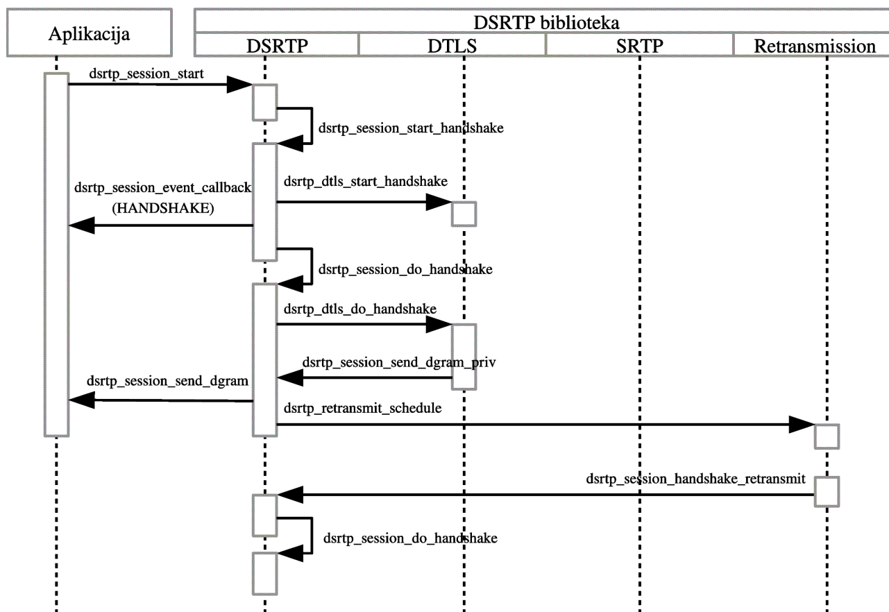
Slika 5.3: Pokretanje DTLS dogovaranja unutar DTLS-SRTP sjednice - sekvencijski dijagram
