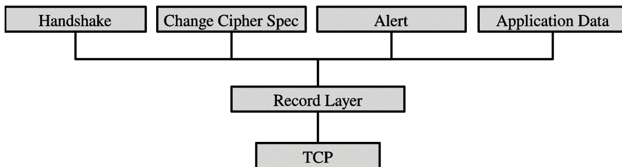
Slika 4.1: Višeslojna struktura TLS protokola
