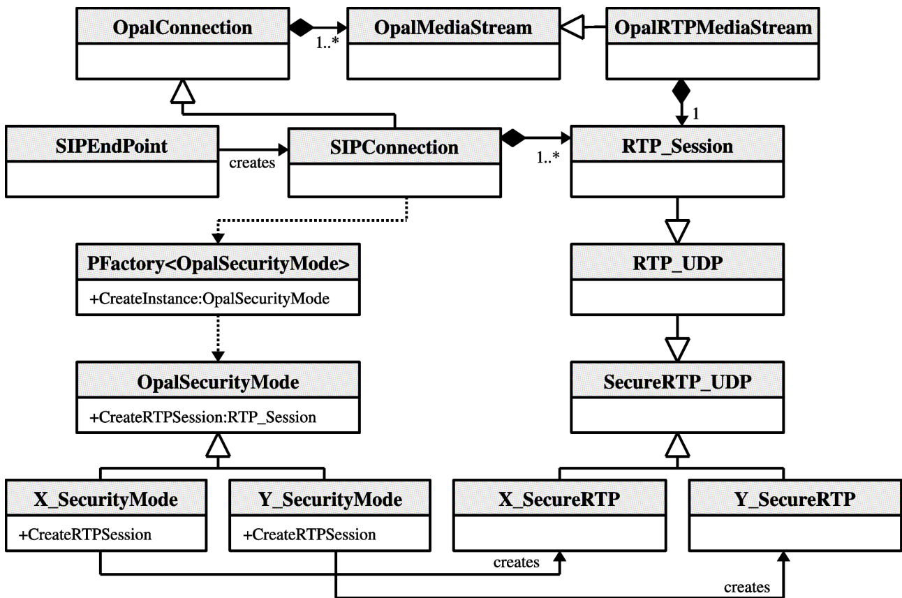
Slika 6.5: Dijagram klasa SIP podsustava OpalVoip biblioteke
