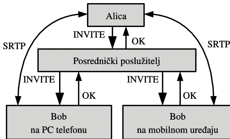
Slika 3.3: SIP grananje
