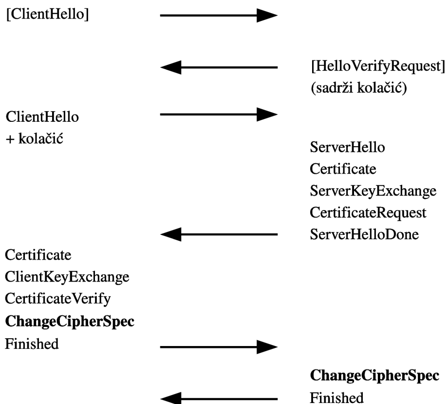
Slika 4.2: DTLS dogovaranje
