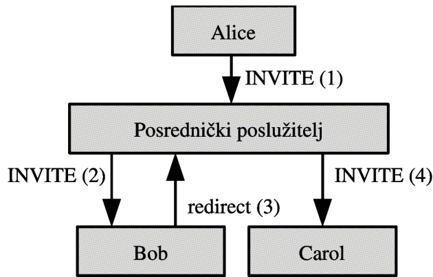
Slika 3.2: SIP preusmjerenje
