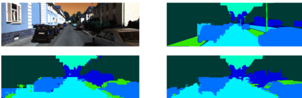
Slika B.4: Rezultati na KITTI skupu podataka, RGB mreža
