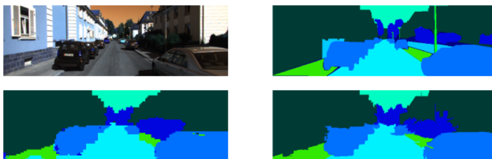
Slika B.6: Rezultati na KITTI skupu podataka, RGBD mreža
