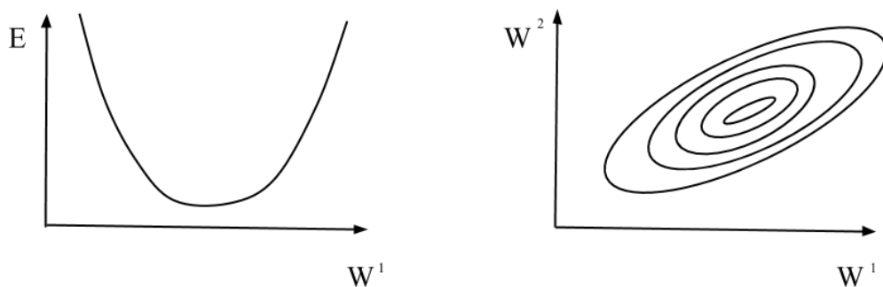
Slika 3.1: Vertikalni i horizontalni presjek funkcije troška
