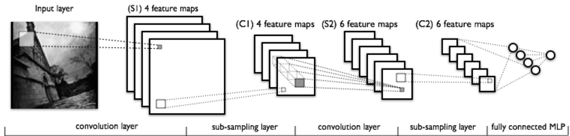
Slika 2.10: LeNet mreža
