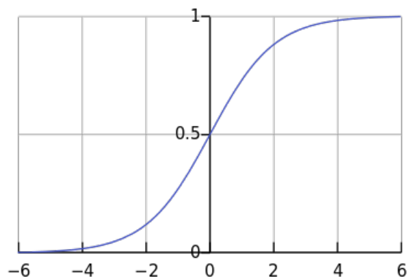
Slika 2.6: Logistička sigmoid funkcija
