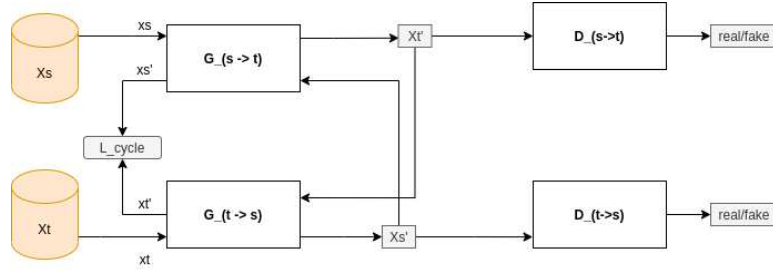
Slika 4.3: Arhitektura CycleGAN [Zhu et al. (2017)] modela za prevođenje domene. Arhitektura se sastoji od dva uvjetna GAN-a, podataka iz izvorne domene S , podataka iz ciljne domene T i kružnog gubitka L_{cycle} . Taj gubitak je definiran kao L1 udaljenost između izvorne slike i njene rekonstrukcije. Rekonstrukcija se dobiva prevođenjem izvorne slike u stan u domenu te ponovnim vraćanjem sintetičke slike u izvornu domenu.
