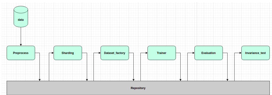
Slika 6.2: Komunikacijski dijagram faza cjevovoda. Komponente cjevovoda komuniciraju preko zajedničkog sučelja. Zbog toga je olakšano dodavanje novih komponenti koji jedino trebaju znati koristiti protokol sučelja, a ne moraju se zamarati implementacijskim detaljima komponenti s kojima direktno komuniciraju. Komponente u zajednički repozitorij upisuju artefakte, tj. objekte koje su namijenjene za pregledavanje i izlaze koje koriste druge komponente.
