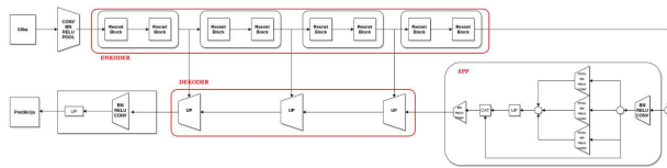
Slika 5.1: Single Scale SwiftNet, crvenom bojom označeni su moduli kodera i dekodera. Između kodera i dekodera nalazi se SPP modul, a na kraju modela nalazi se slojevi za fino podešavanje modela na zadani skup podataka.
