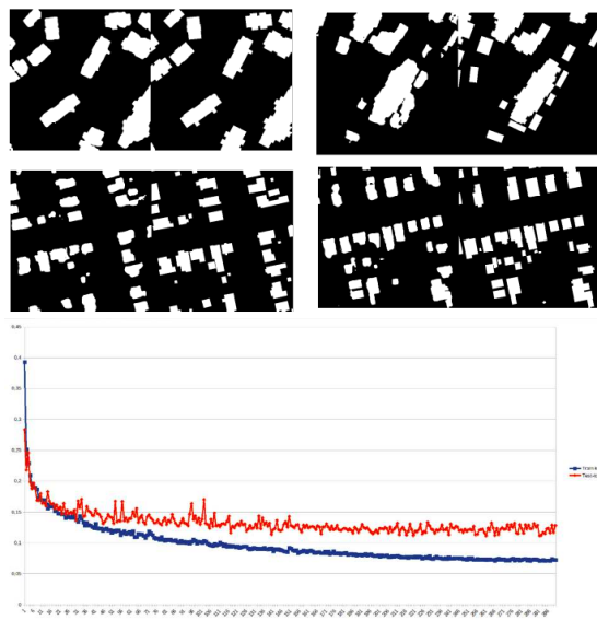
Slika 6.6: Na gornjoj slici mogu se vidjeti 4 primjera parova predikcija i oznaka na testnim podacima. Na donjoj slici je prikazana funkcija gubitka tijekom 300 epoha. Crvenom krivuljom prikazano je kretanje gubitka na skupu za validiranje, a s plavom kretanje gubitka na skupu za učenje. Nakon nekog vremena dolazi do zasićenja procesa.
