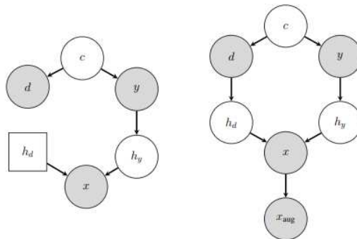
Slika 3.1: Simulacija intervencije pomoću augmentacije. Na lijevoj slici prikazan je generativni model u kojem je napravljena intervencija na značajkama domene, dok je na desnoj slici prikazan graf kojem je dodana još jedna varijabla x_{aug} koja predstavlja proces augmentacije podataka.
