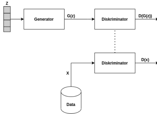
Slika 4.2: Osnovna arhitektura GAN modela. Generator generira lažne primjere, dok diskriminator klasificira primjere u stvarne ili lažne.
