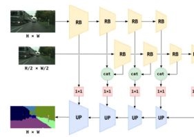
Slika 5.2: SwiftNet s 2-razinskom piramidom. K -razinska piramida interpolira slike na k različitih rezolucija što rezultira povećanjem receptivnog polja aktivacija. Parametri kodera su dijeljeni. Značajke istih rezolucija se spajaju lateralnim vezama i kombiniraju sa semantički bogatijim značajkama.
