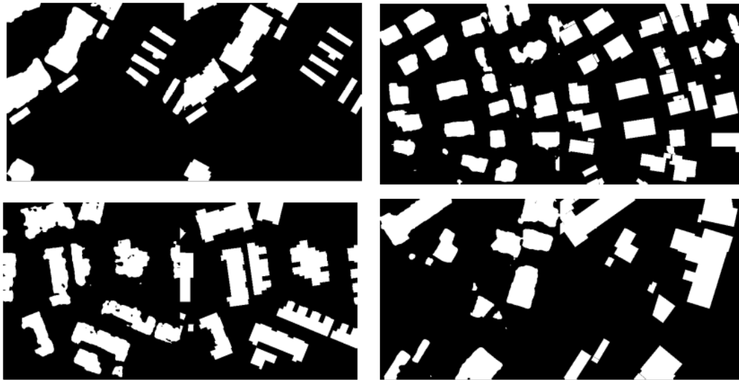
Slika 6.8: Primjeri nasumično odabranih predikcija modela na različitim domenama. Na lijevoj strani slike nalaze se predikcije, a na desnoj strani oznake kuća. Krenuvši od prvog stupca i retka ka drugom stupcu i retku u smjeru kazaljke na sat slike predstavljaju: model učen na Austinu i testiran na Austinu , model učen na Austinu i testiran na Tirolu , model učen na Tirolu i testiran na Austinu i konačno model učen na Tirolu i testiran na Tirolu .
