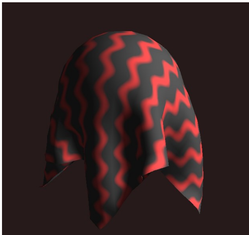
Slika 3.2.2 – Konstanta opruge je 10
