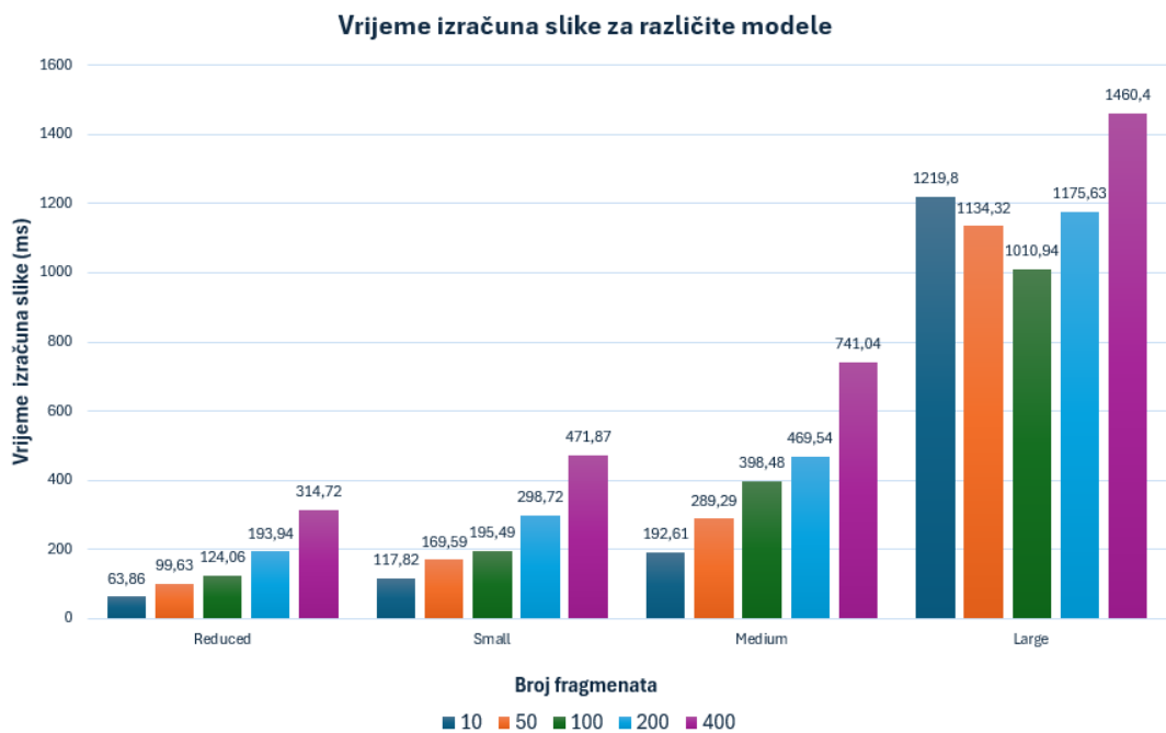
Slika 6.2 Vrijeme izračuna slike za različite modele
