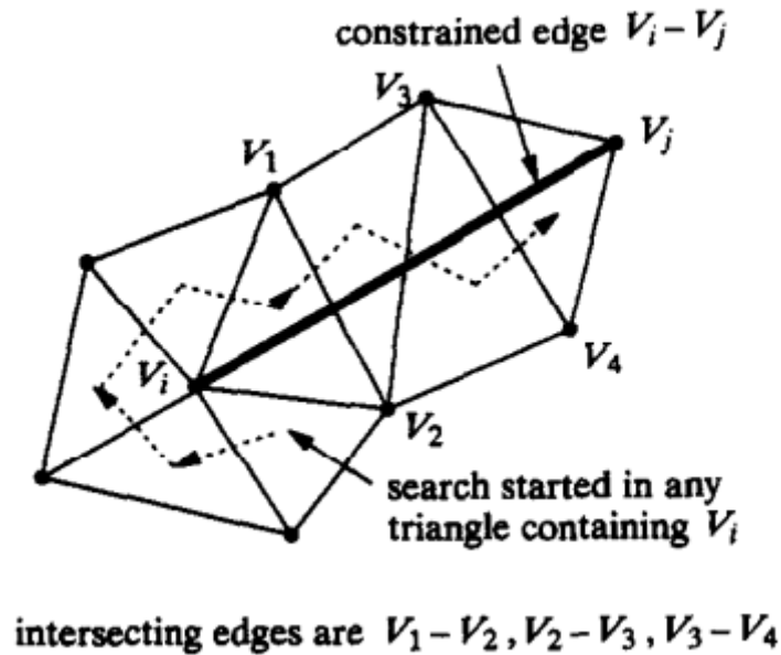
Slika 3.6 Pronalazak presjeka između stranica trokuta i ruba ograničenja[3]
