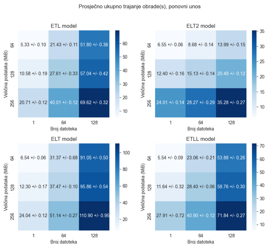
Slika 7.2. Toplinska mapa prosječnog ukupnog trajanja obrade u sekundama za ponovni unos.
