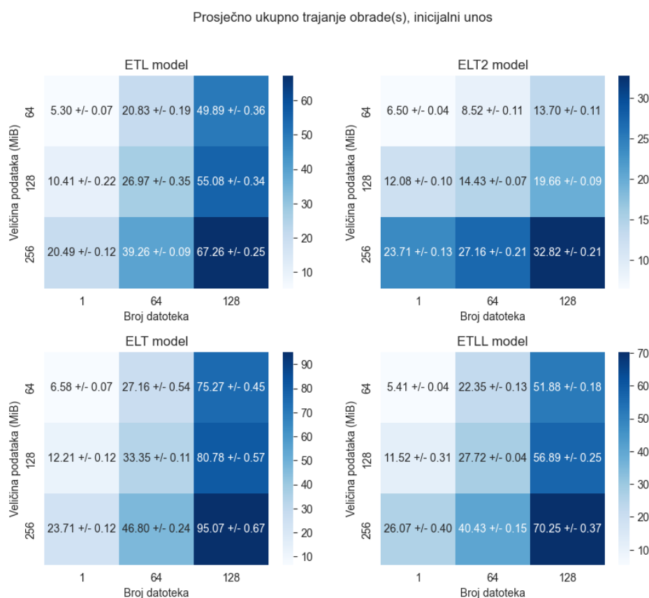
Slika 7.1. Toplinska mapa prosječnog ukupnog trajanja obrade u sekundama za inicijalni unos.
