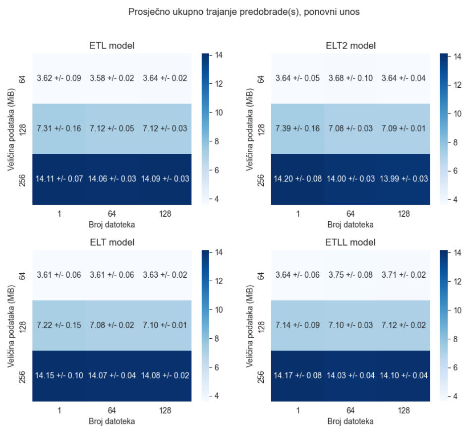
Slika 7.4. Toplinska mapa prosječnog ukupnog trajanja predobrade u sekundama za ponovni unos.
