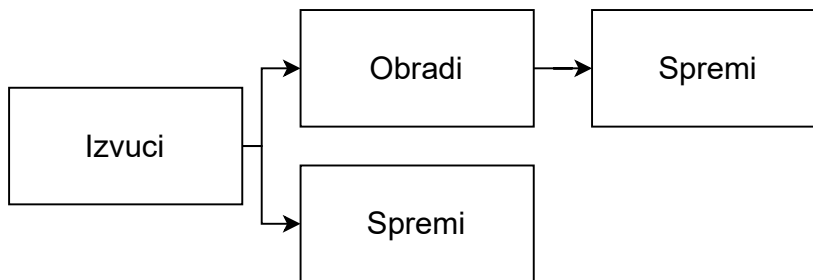
Slika 4.3. Model obrade podataka ETLL.
