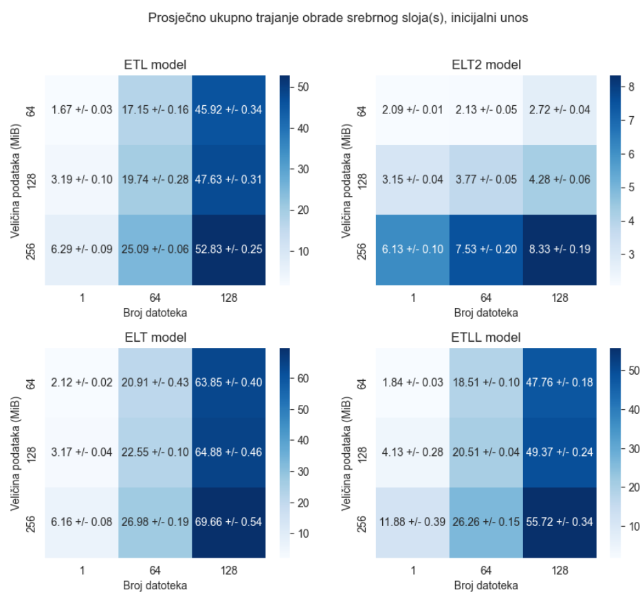
Slika 7.8. Toplinska mapa prosječnog ukupnog trajanja obrade srebrnog sloja u sekundama za inicijalni unos.
