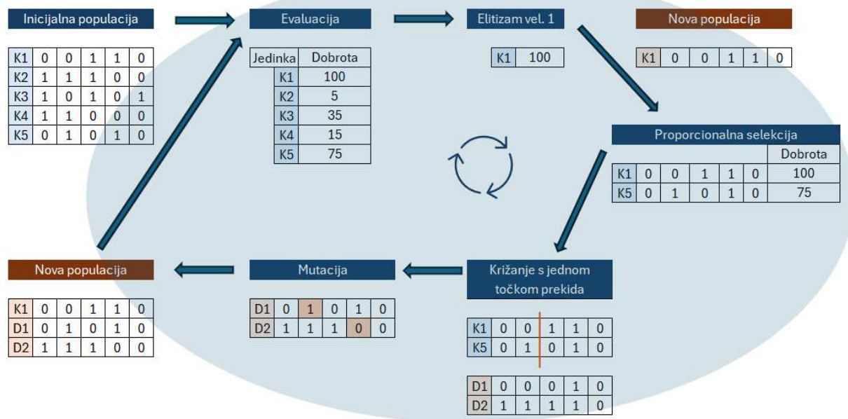
Slika 2.5: Iteracija genetskog algoritma
