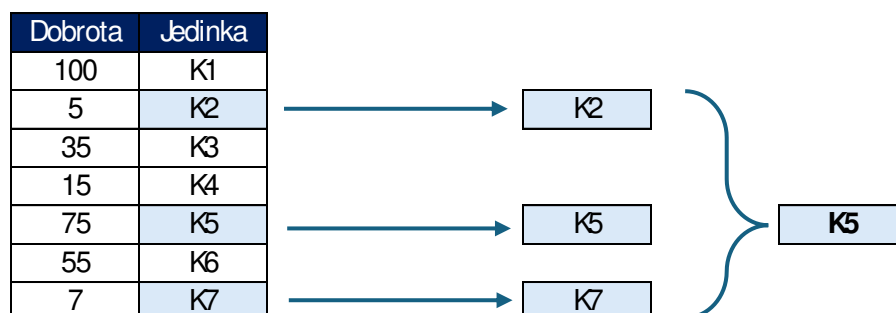
Slika 2.3: Turnirska selekcija
