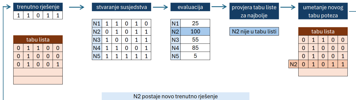
Slika 2.7 – Iteracija tabu-pretrage
