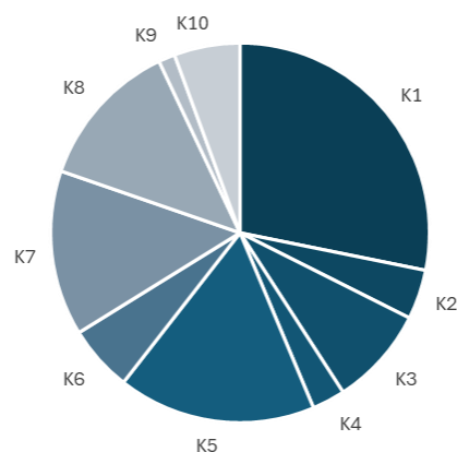
Slika 2.2: Proporcionalna selekcija
