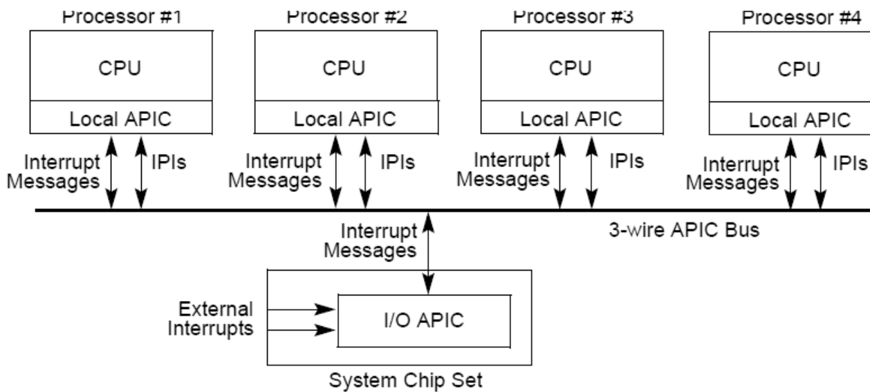
Slika 3.12. Sklopovlje za prihvatanje i proslijeđivanje prekida u Intelovim arhitekturama (izvor Intel)
