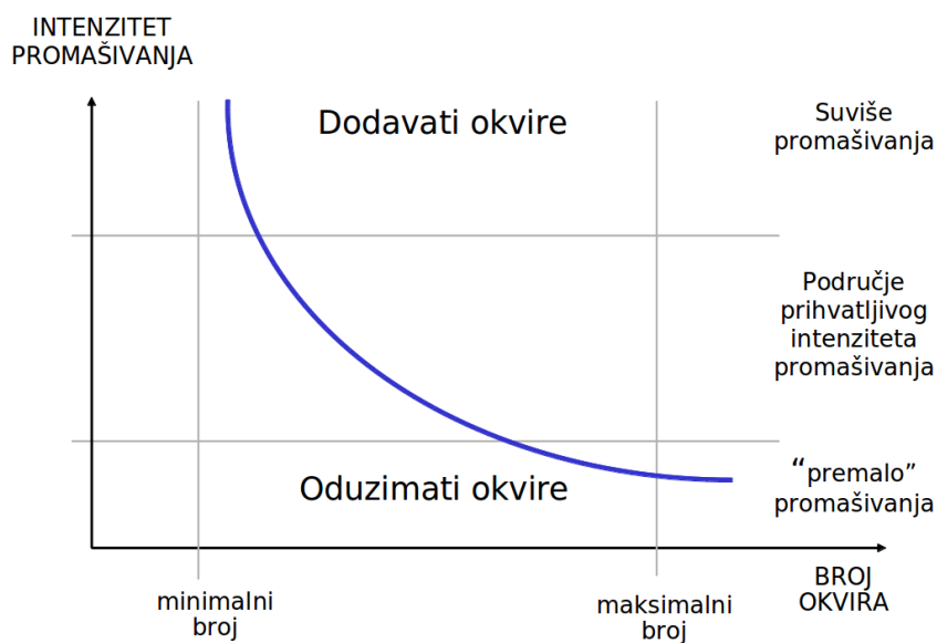
Slika 8.20. Dodjela okvira prema intenzitetu promašaja
