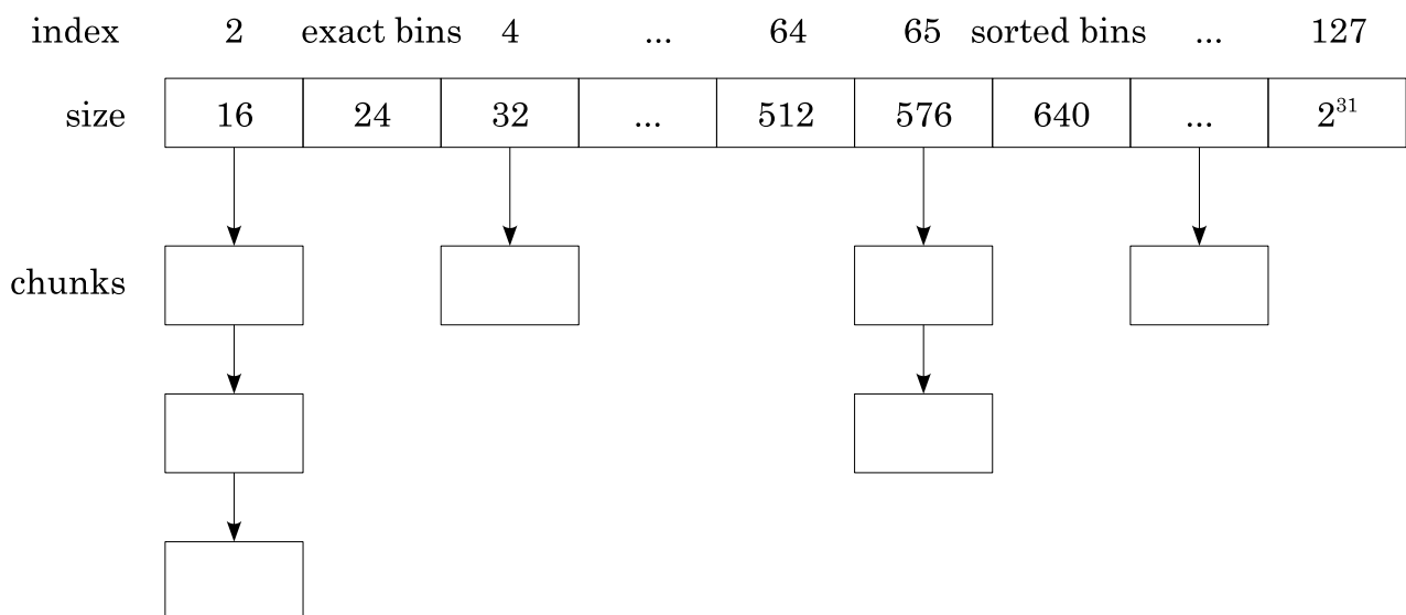
Slika 8.22. Liste slobodnih blokova kod Doug Lee malloc metode
