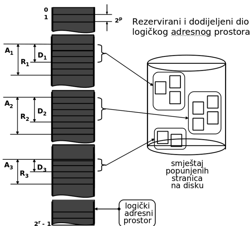
Slika 8.19. Rezervirani i dodijeljeni dijelovi adresnog prostora procesa
