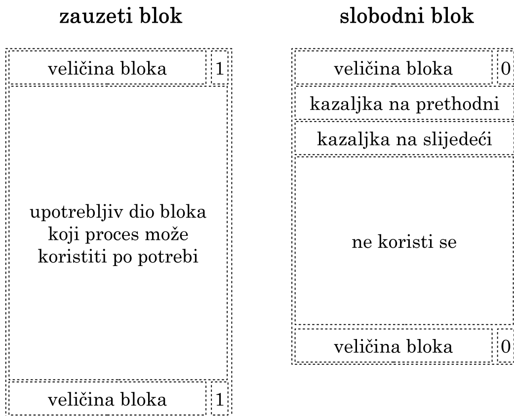
Slika 8.21. Primjer zaglavlja zauzetih i slobodnih blokova
