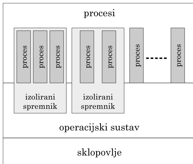
Slika 10.3. Virtualizacija na razini spremnika
