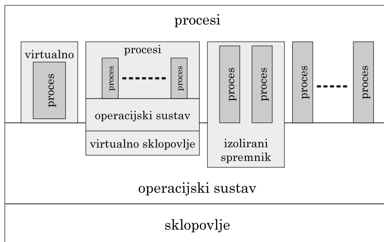
Slika 10.6. Paralelno korištenje različitih tipova virtualizacije
