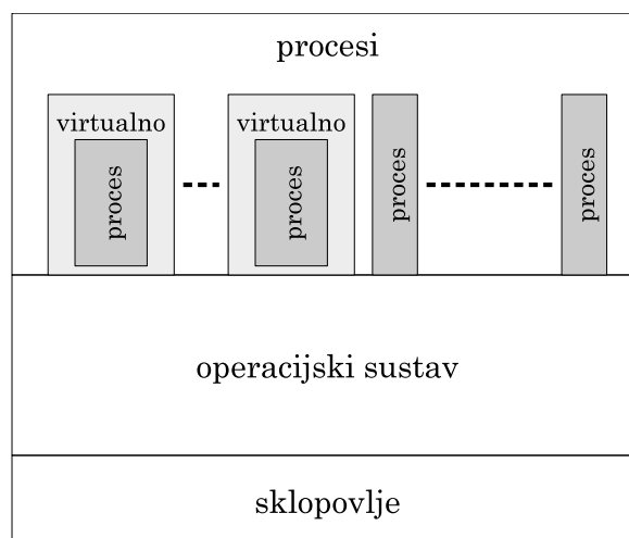
Slika 10.2. Virtualizacija na razini aplikacije
