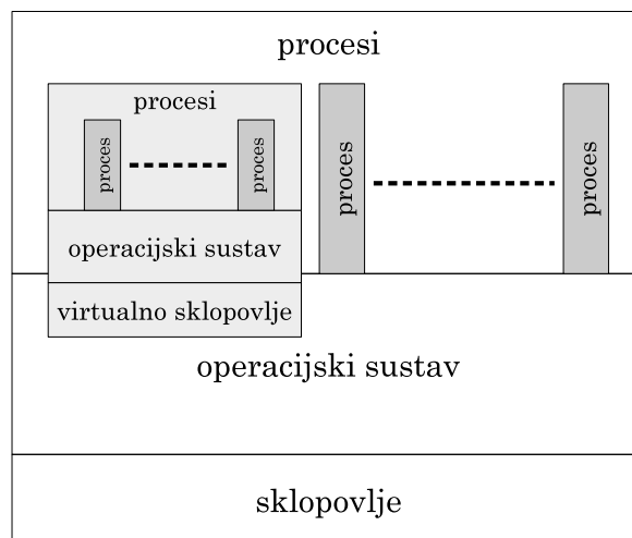
Slika 10.4. Virtualizacija na razini programa
