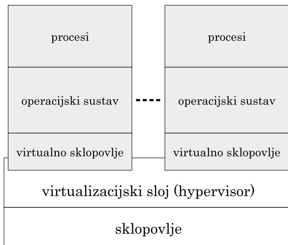
Slika 10.5. Virtualizacija na razini operacijskog sustava i sklopovlja
