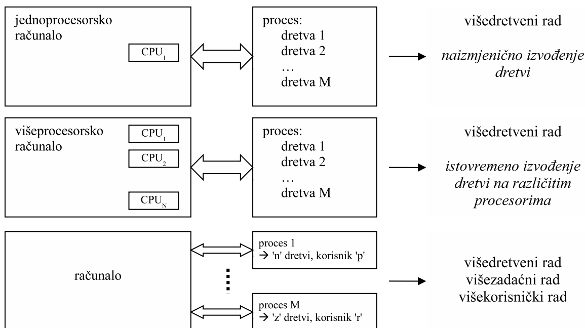
Slika 4.3. Usporedba raznih višedretvenih sustava
