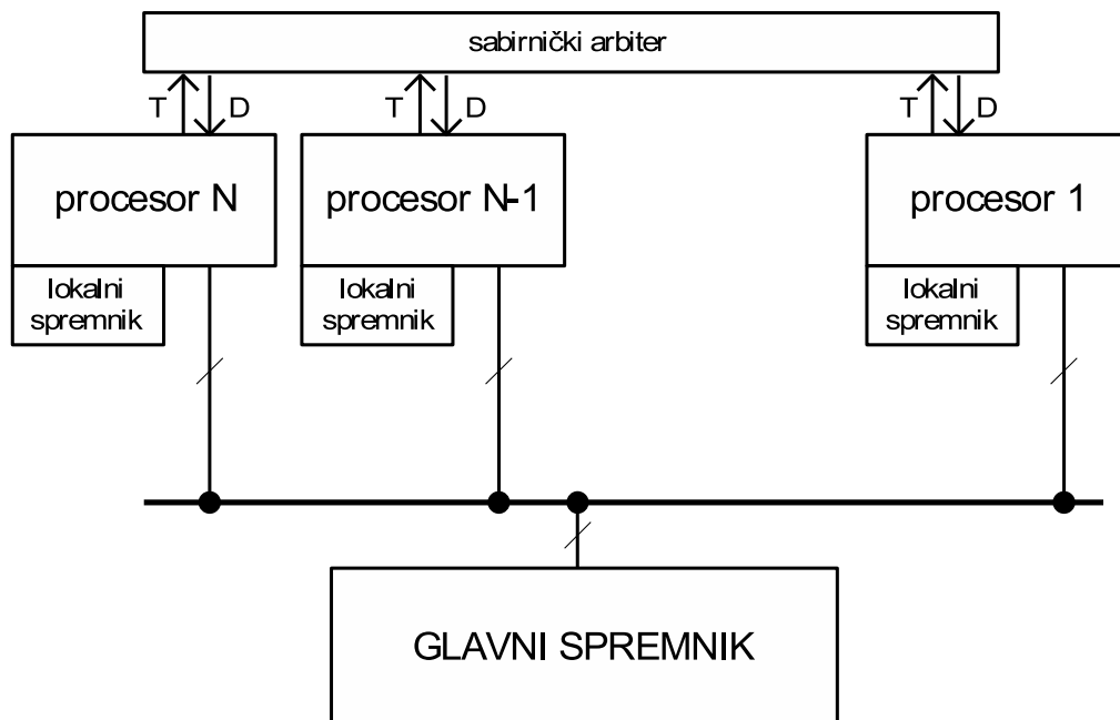
Slika 3.8. Višeprocessorski sustav
