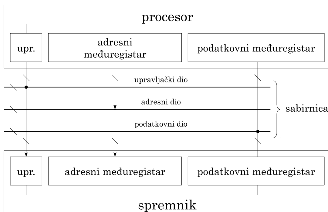
Slika 2.2. Model sabirnice
