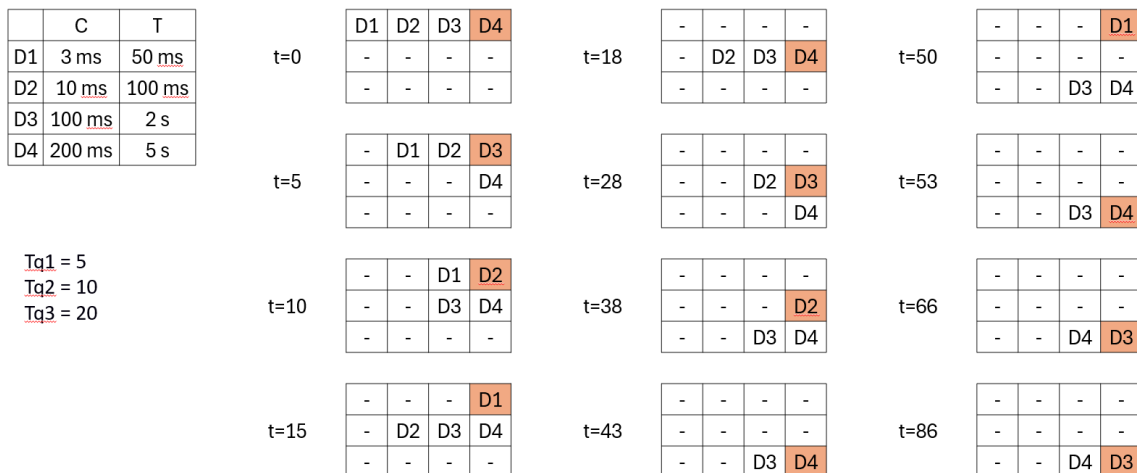
Slika 7.19. Primjer rada algoritma MFQ
