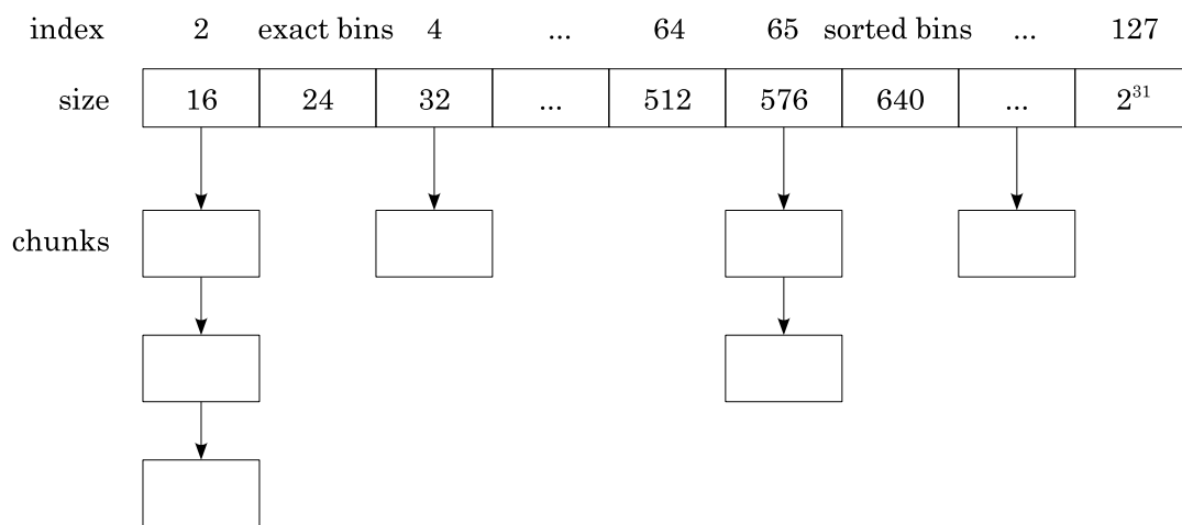
Slika 8.22. Liste slobodnih blokova kod Doug Lee malloc metode
