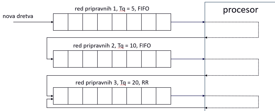
Slika 7.18. Primjer reda pripravnih kod algoritma MFQ
