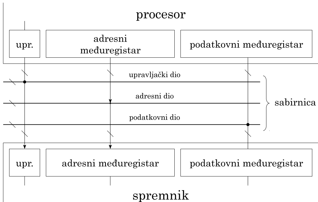
Slika 2.6. Model sabirnice
