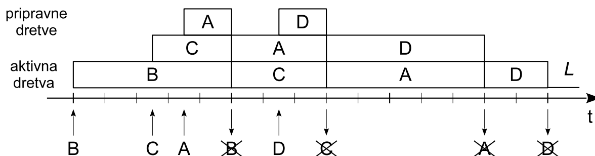
Slika 7.14. Raspoređivanje po redu prispjeća
