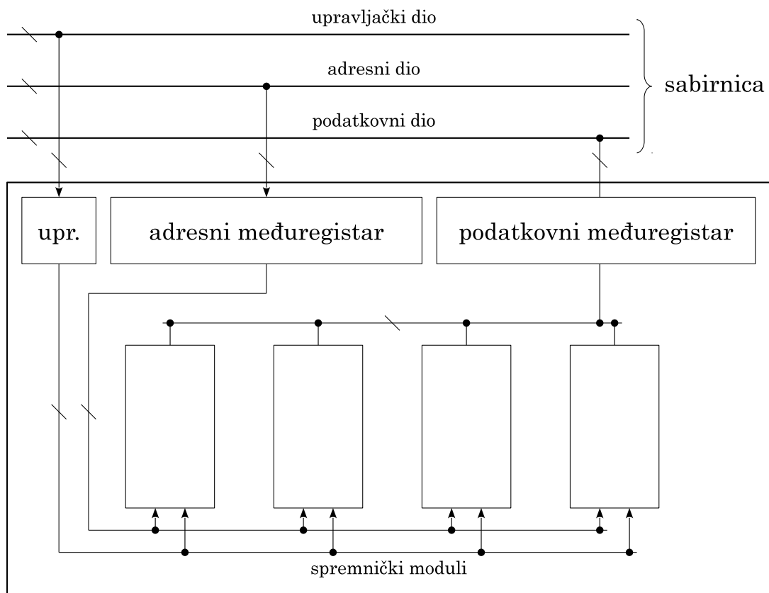
Slika 2.7. Model spremnika
