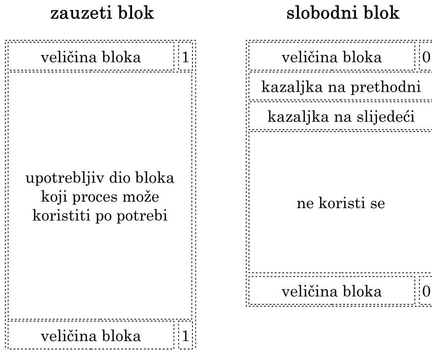
Slika 8.21. Primjer zaglavlja zauzetih i slobodnih blokova
