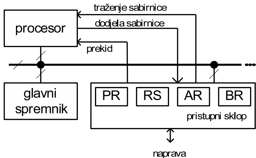
Slika 3.10. Pristupni sklop s izravnim pristupom spremniku
