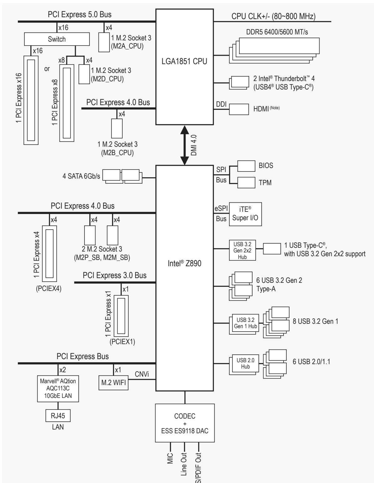
Slika 2.5. Primjer arhitekture matične ploče Z90 AORUS MASTER (izvor: GIGABYTE)
