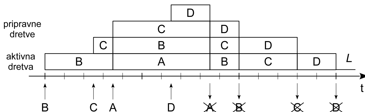
Slika 7.15. Raspoređivanje prema prioritetu
