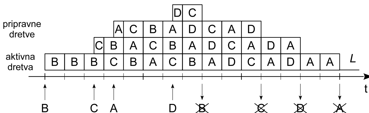
Slika 7.4. Kružno raspoređivanje
