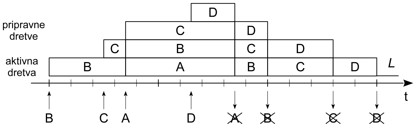
Slika 7.3. Raspoređivanje prema prioritetu
