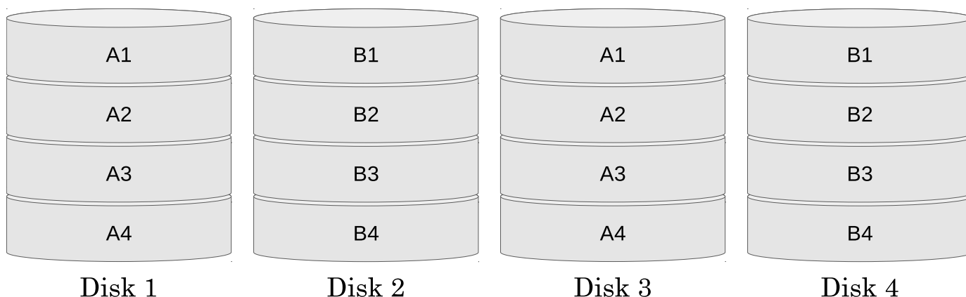
Slika 9.3. Primjer RAID 1 sustava
