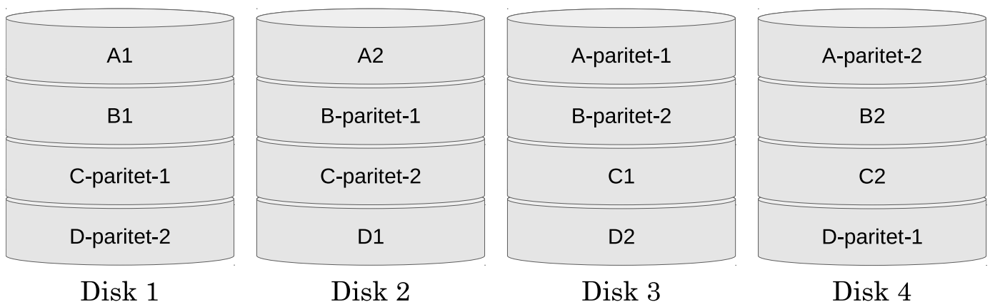
Slika 9.5. Primjer RAID 6 sustava
