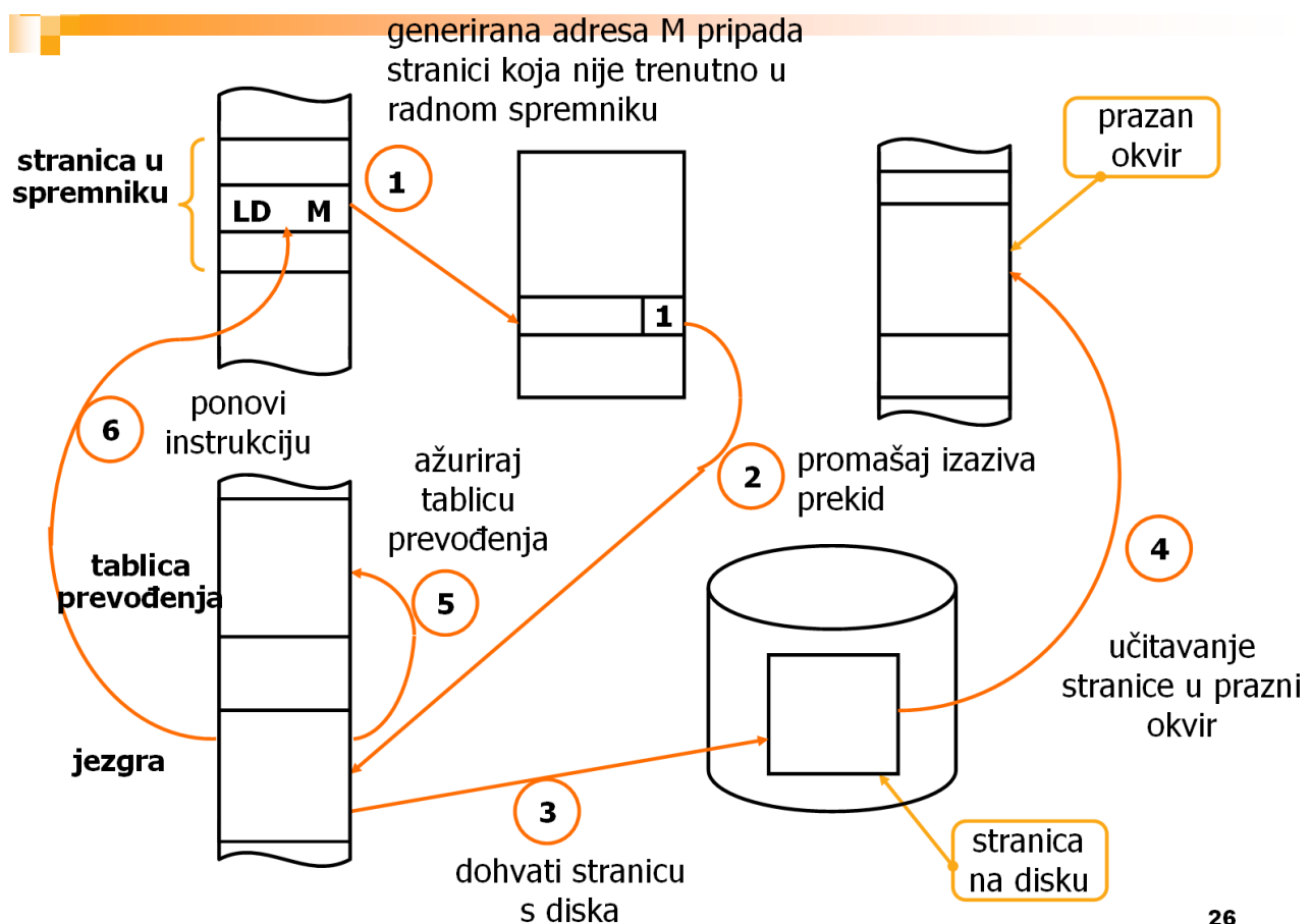
Slika 8.18. Operacije po promašaju
