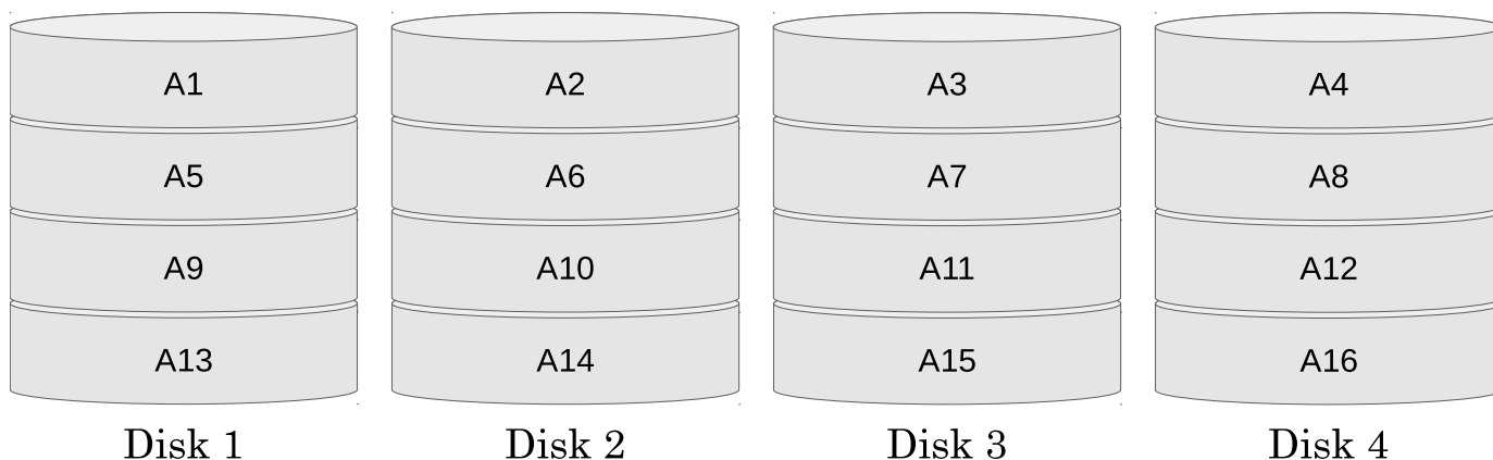
Slika 9.2. Primjer RAID 0 sustava
