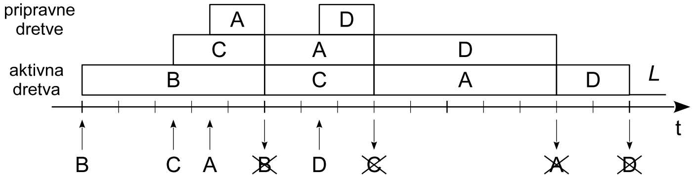
Slika 7.2. Raspoređivanje po redu prispjeća
