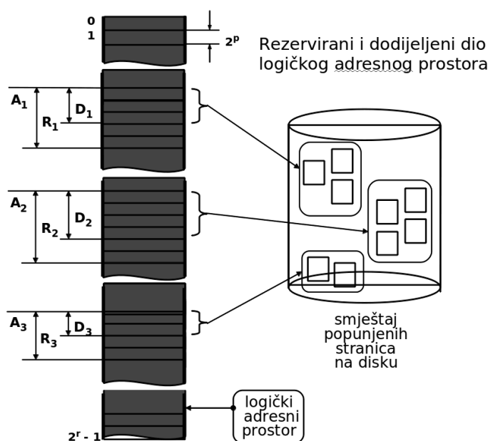
Slika 8.20. Rezervirani i dodijeljeni dijelovi adresnog prostora procesa
