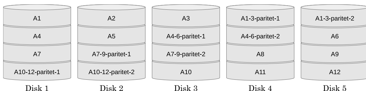
Slika 9.9. Primjer RAID 6 sustava
