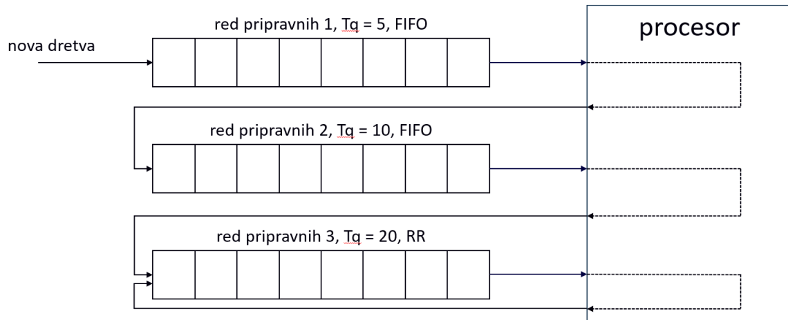
Slika 7.18. Primjer reda pripravnih kod algoritma MFQ
