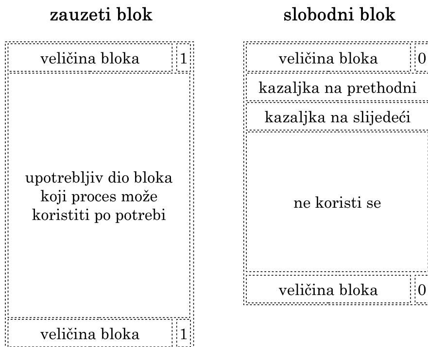
Slika 8.22. Primjer zaglavlja zauzetih i slobodnih blokova
