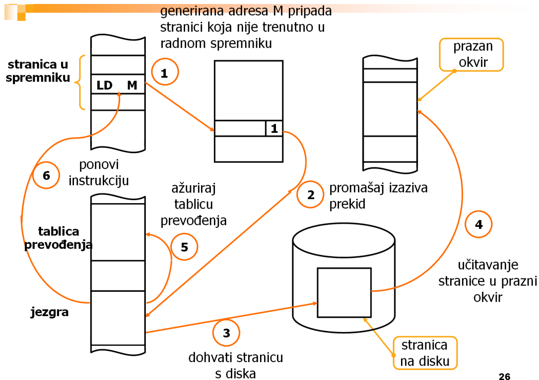
Slika 8.19. Operacije po promišaju
