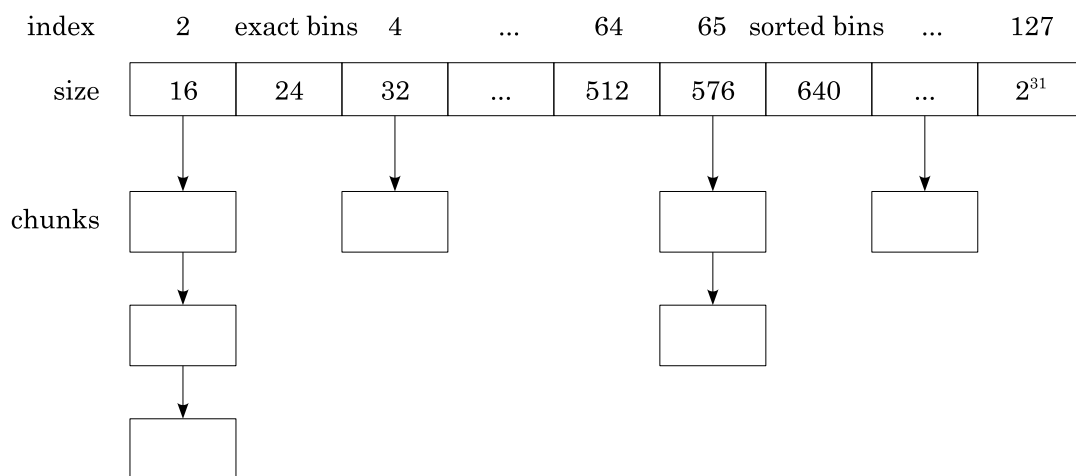
Slika 8.23. Liste slobodnih blokova kod Doug Lee malloc metode
