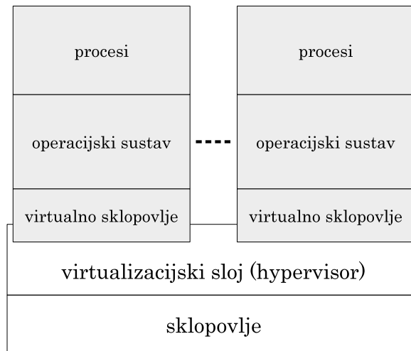
Slika 11.5. Virtualizacija na razini operacijskog sustava i sklopovlja
