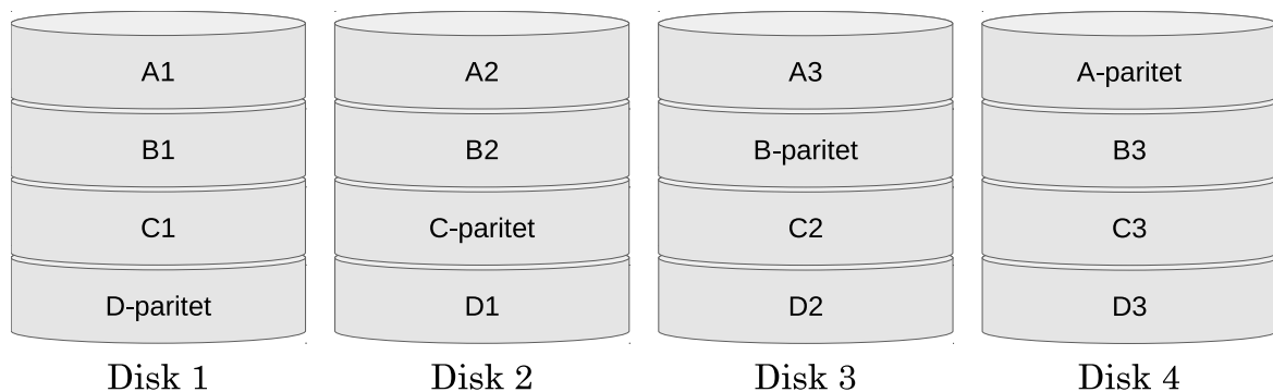
Slika 9.8. Primjer RAID 5 sustava
