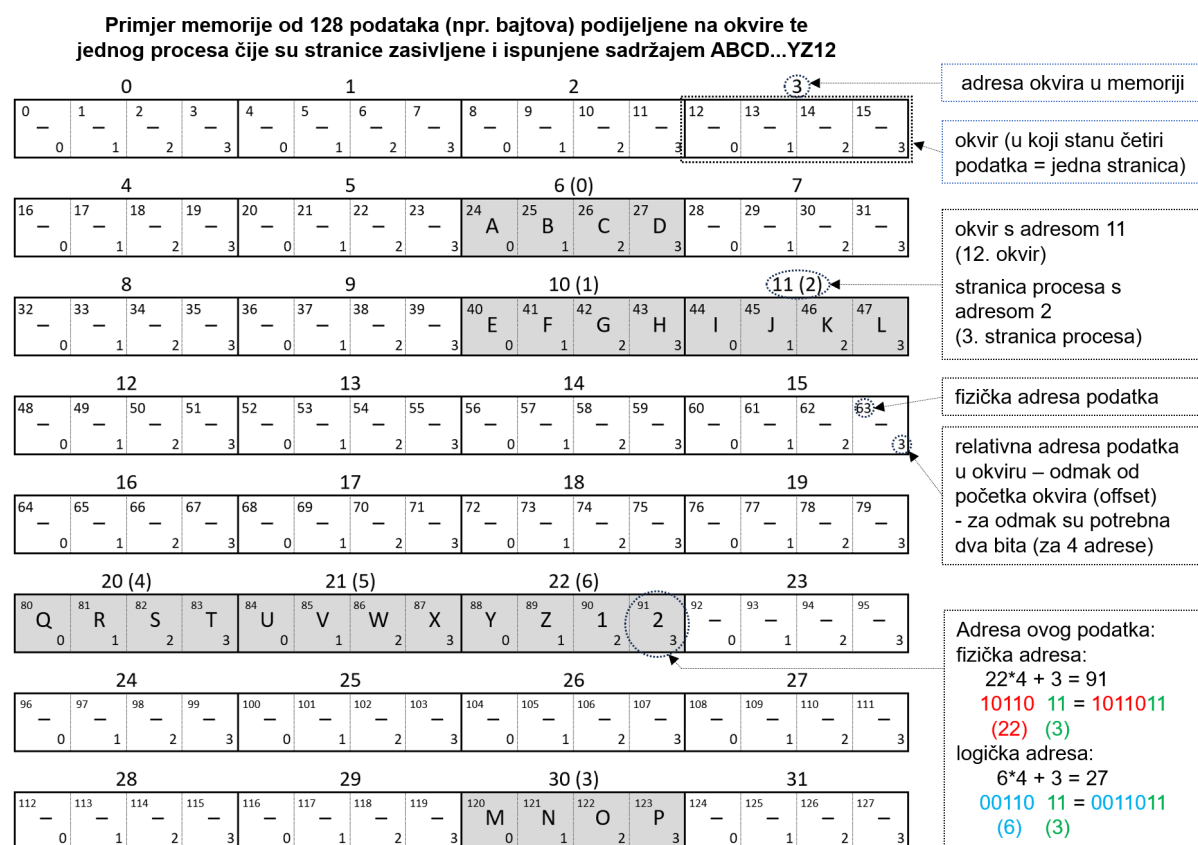
Slika 8.11. Ilustrativni primjer s malim spremnikom i malim okvirima
