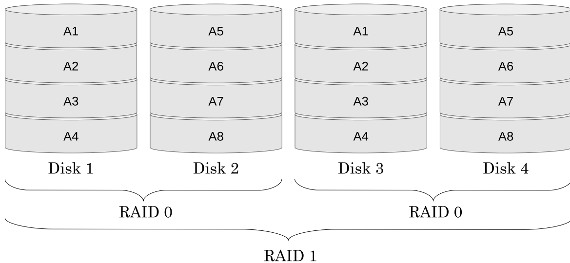
Slika 9.7. Primjer RAID 0+1 sustava
