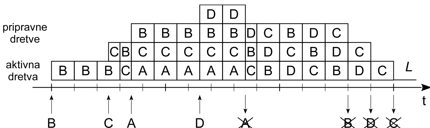
Slika 7.21. Raspoređivanje prema SCHED_RR
