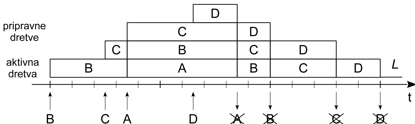
Slika 7.20. Raspoređivanje prema SCHED_FIFO
