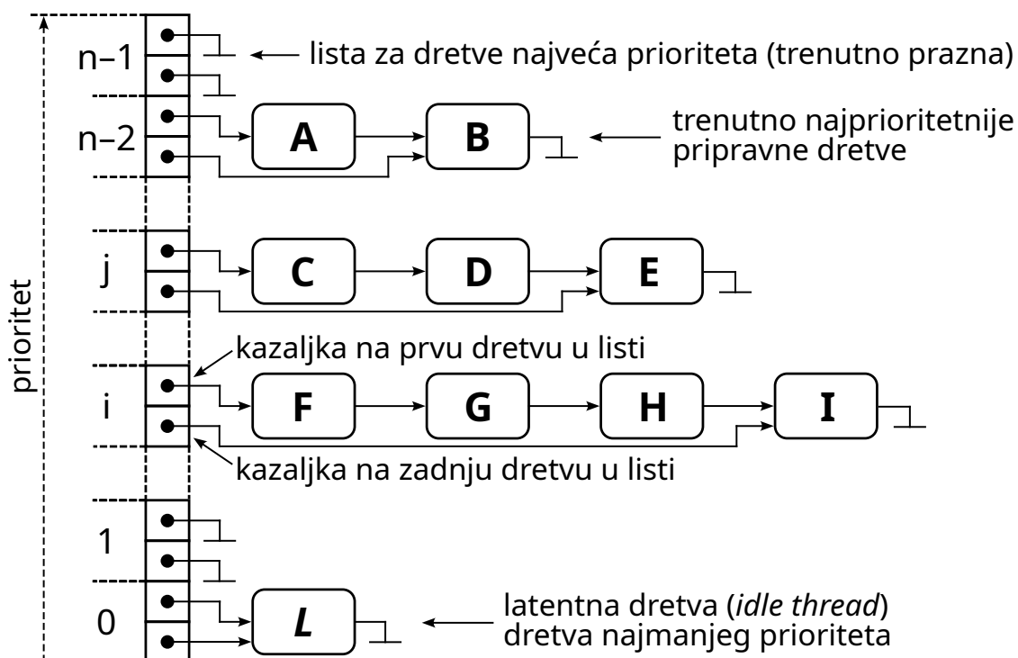
Slika 7.17. Sustav pripravnih dretvi raspodijeljen prema prioritetu
