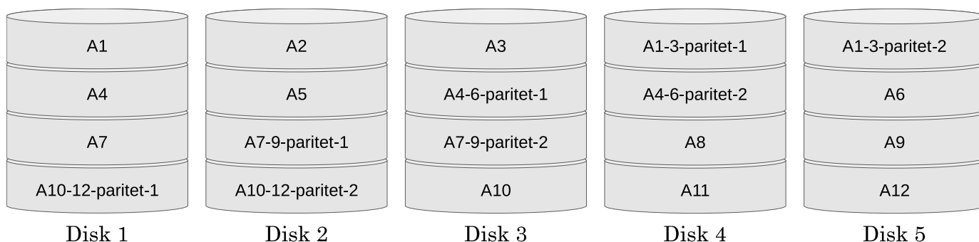
Slika 9.9. Primjer RAID 6 sustava
