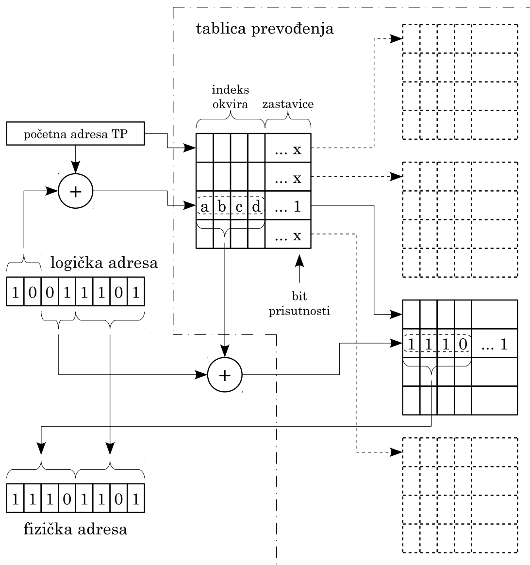
Slika 8.16. Primjer dvorazinske organizacije tablice prevođenja
