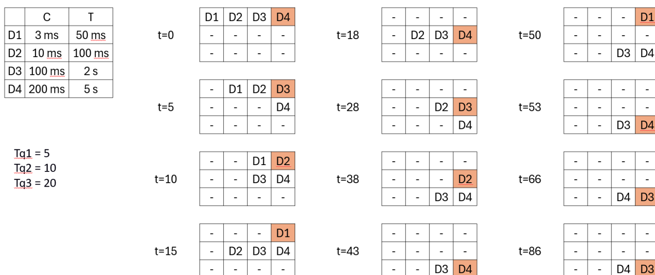
Slika 7.19. Primjer rada algoritma MFQ
