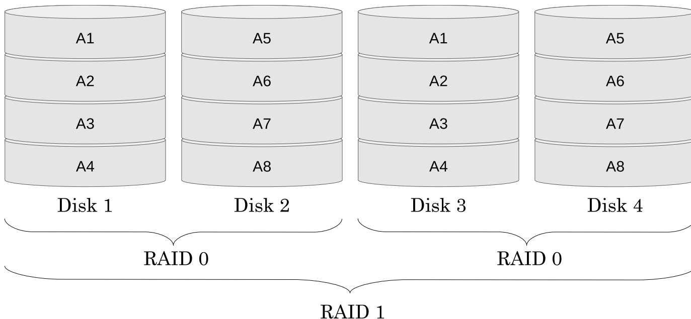
Slika 9.7. Primjer RAID 0+1 sustava
