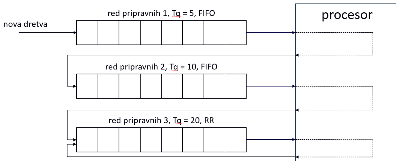
Slika 7.18. Primjer reda pripravnih kod algoritma MFQ
