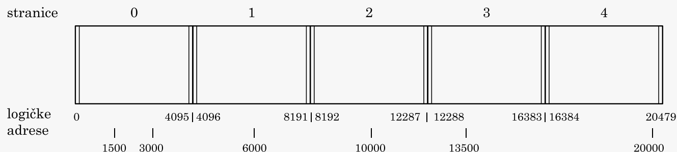
Slika 8.14. Proces, u logičkom adresnom prostoru
