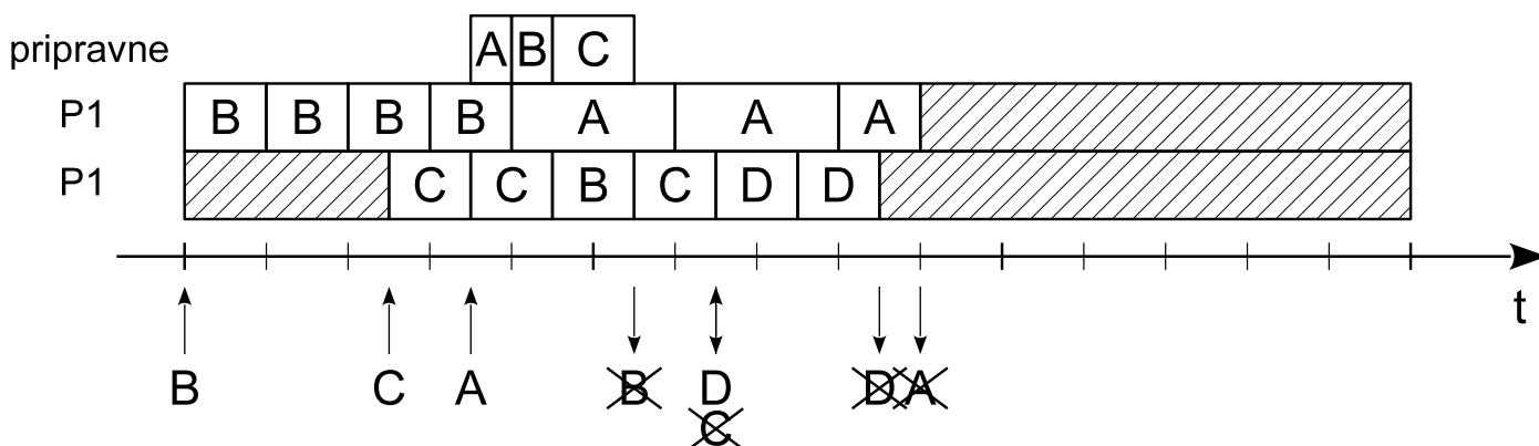
Slika 7.25. Raspoređivanje prema SCHED_OTHER
