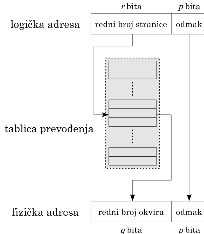
Slika 8.12. Pretvorba adrese kod straničenja
