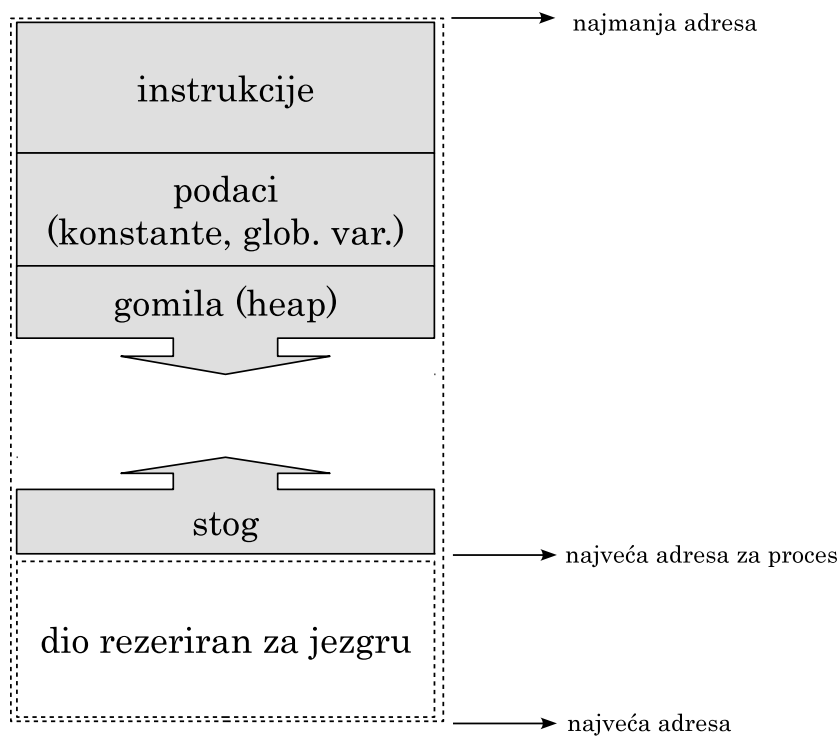
Slika 8.15. Struktura procesa (logički adresni prostor)
