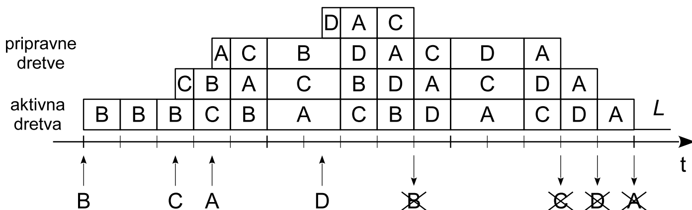
Slika 7.22. Raspoređivanje prema SCHED_OTHER
