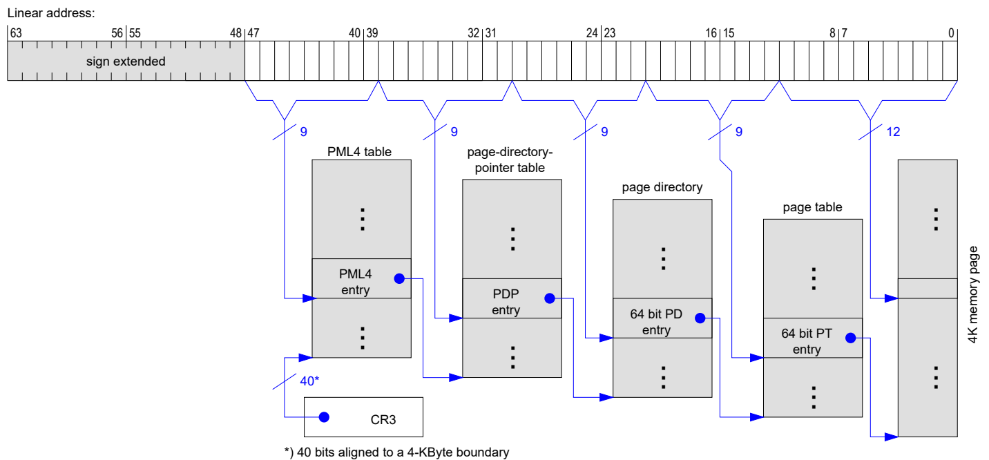
Slika 8.18. Primjer 5-razinske organizacije tablice prevođenja kod arhitekture x86-64 ( izvor )
