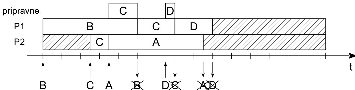
Slika 7.23. Raspoređivanje prema SCHED_FIFO
