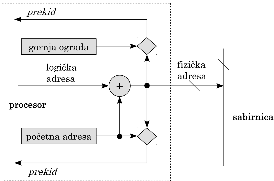
Slika 8.8. Pretvorba adresa s zaštitom spremnika
