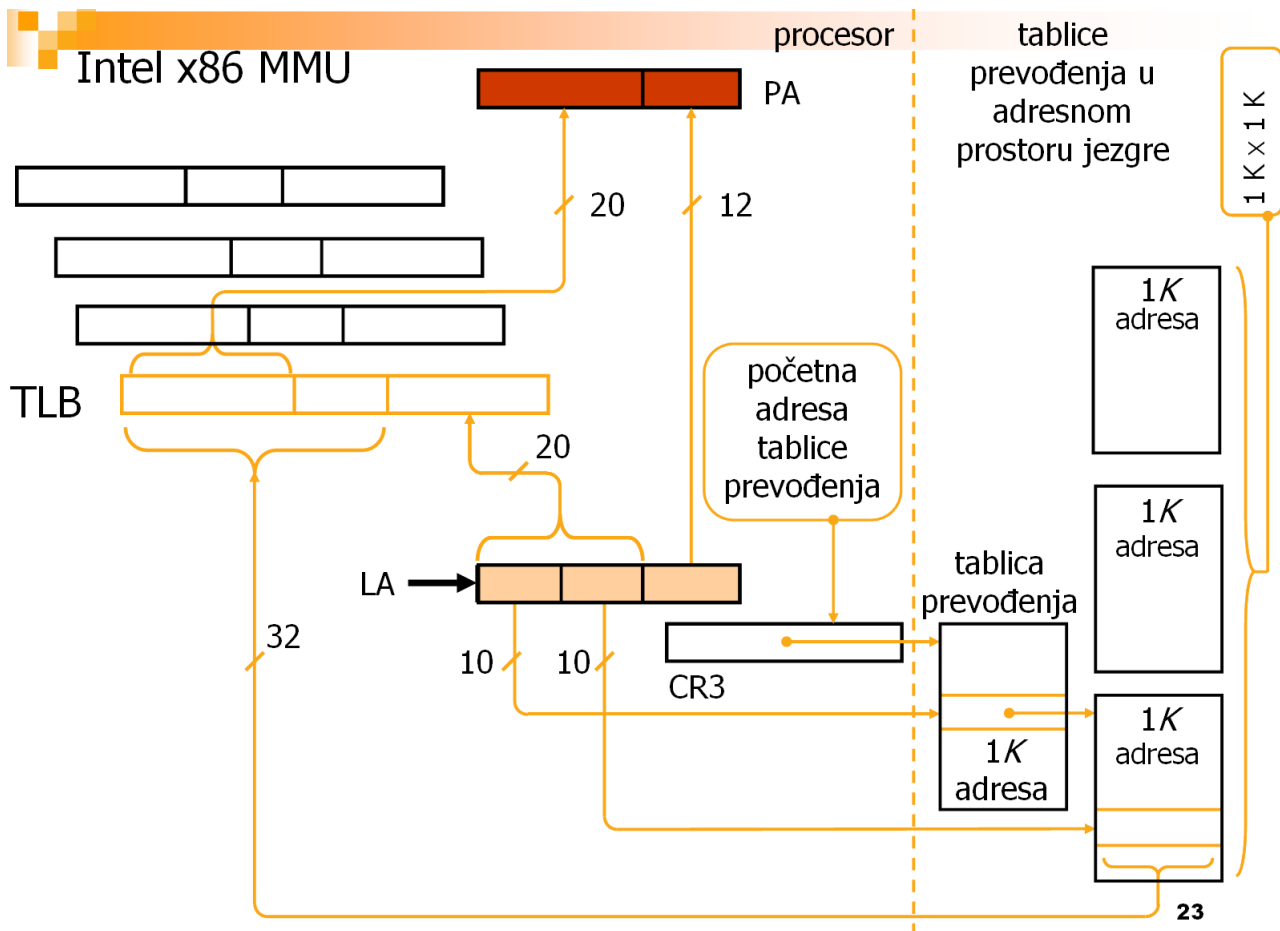
Slika 8.17. Primjer dvorazinske organizacije kod x86 arhitekture
