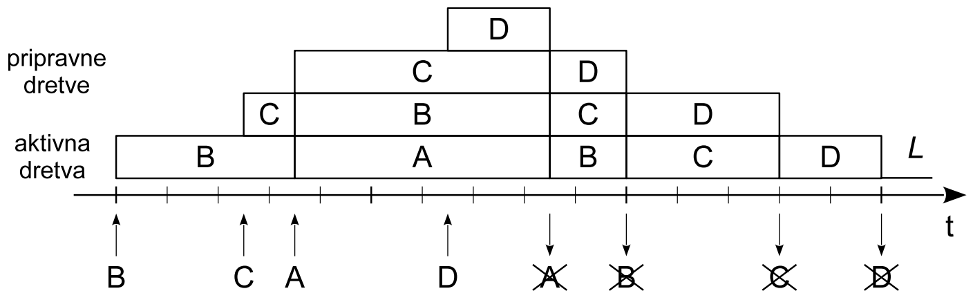
Slika 7.15. Raspoređivanje prema prioritetu
