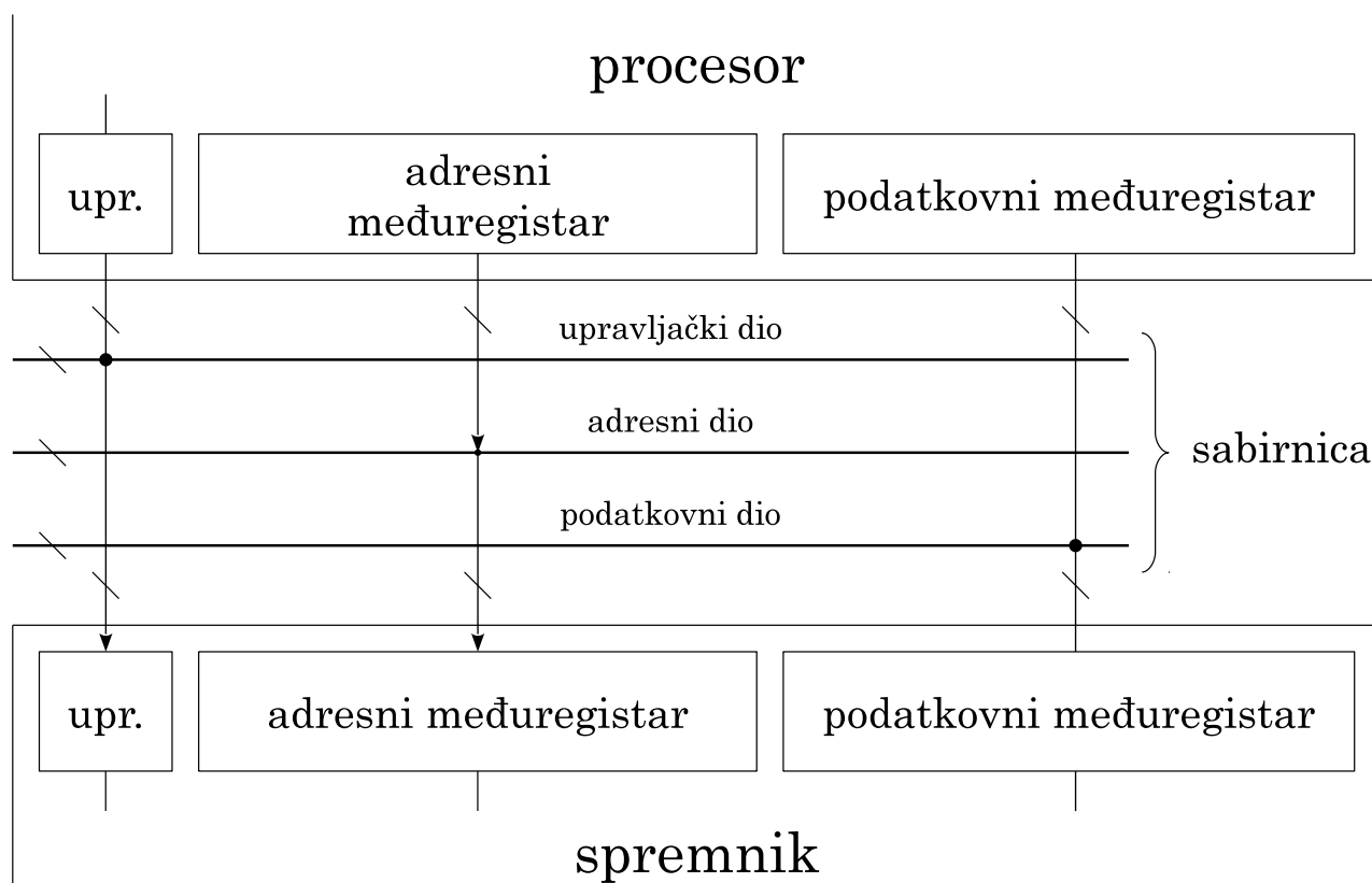
Slika 2.6. Model sabirnice
