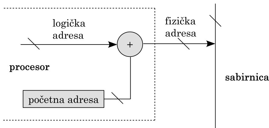
Slika 8.6. Sklop za pretvorbu logičke adrese u fizičku
