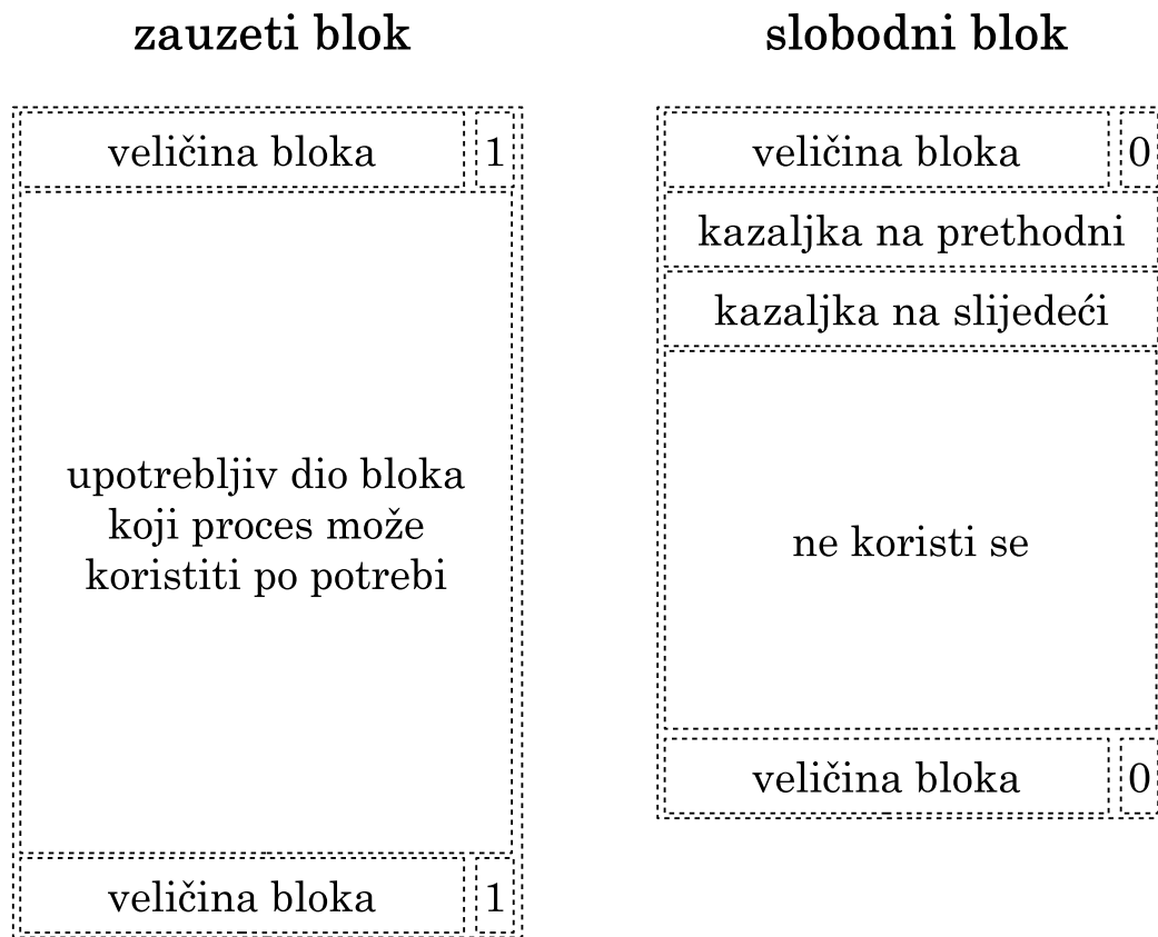
Slika 8.22. Primjer zaglavlja zauzetih i slobodnih blokova
