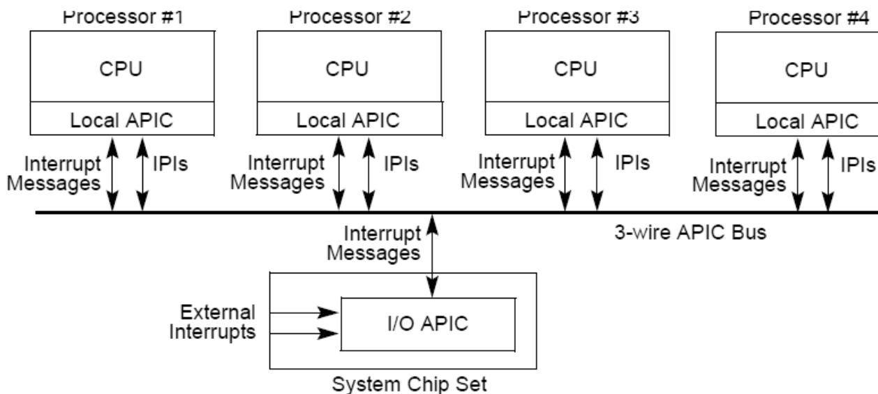
Slika 3.12. Sklopovlje za prihvrat i prosljeđivanje prekida u Intelovim arhitekturama (izvor Intel)
