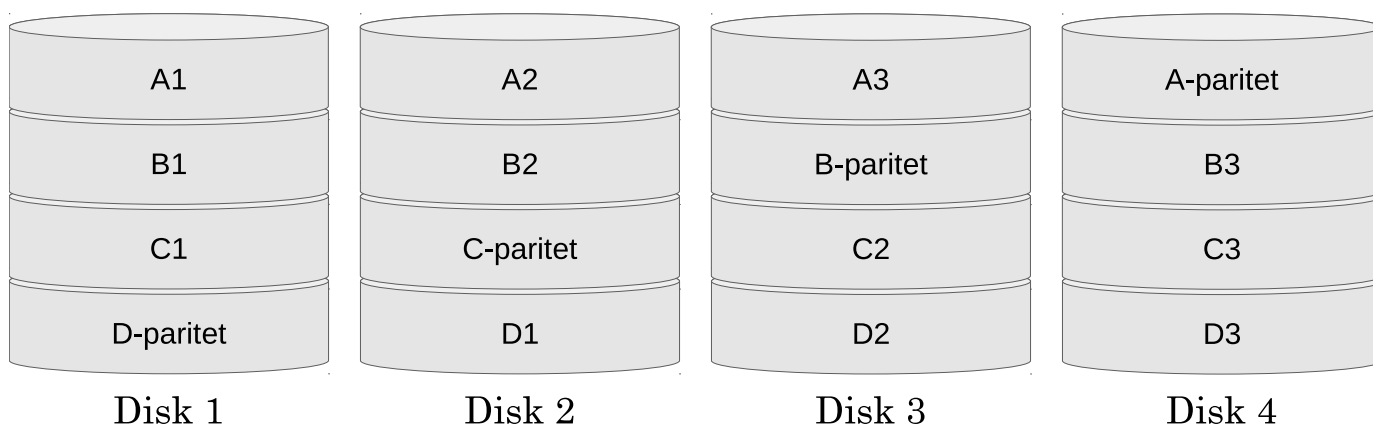
Slika 9.8. Primjer RAID 5 sustava
