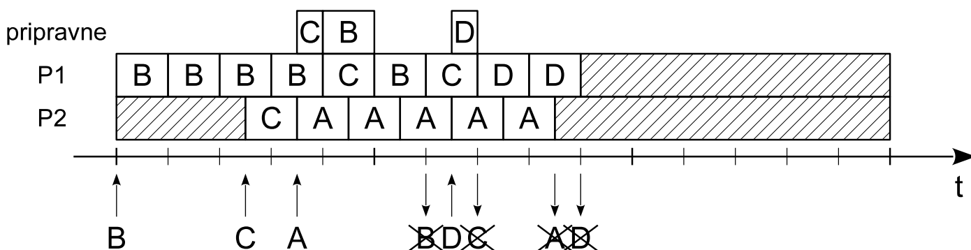
Slika 7.24. Raspoređivanje prema SCHED_RR
