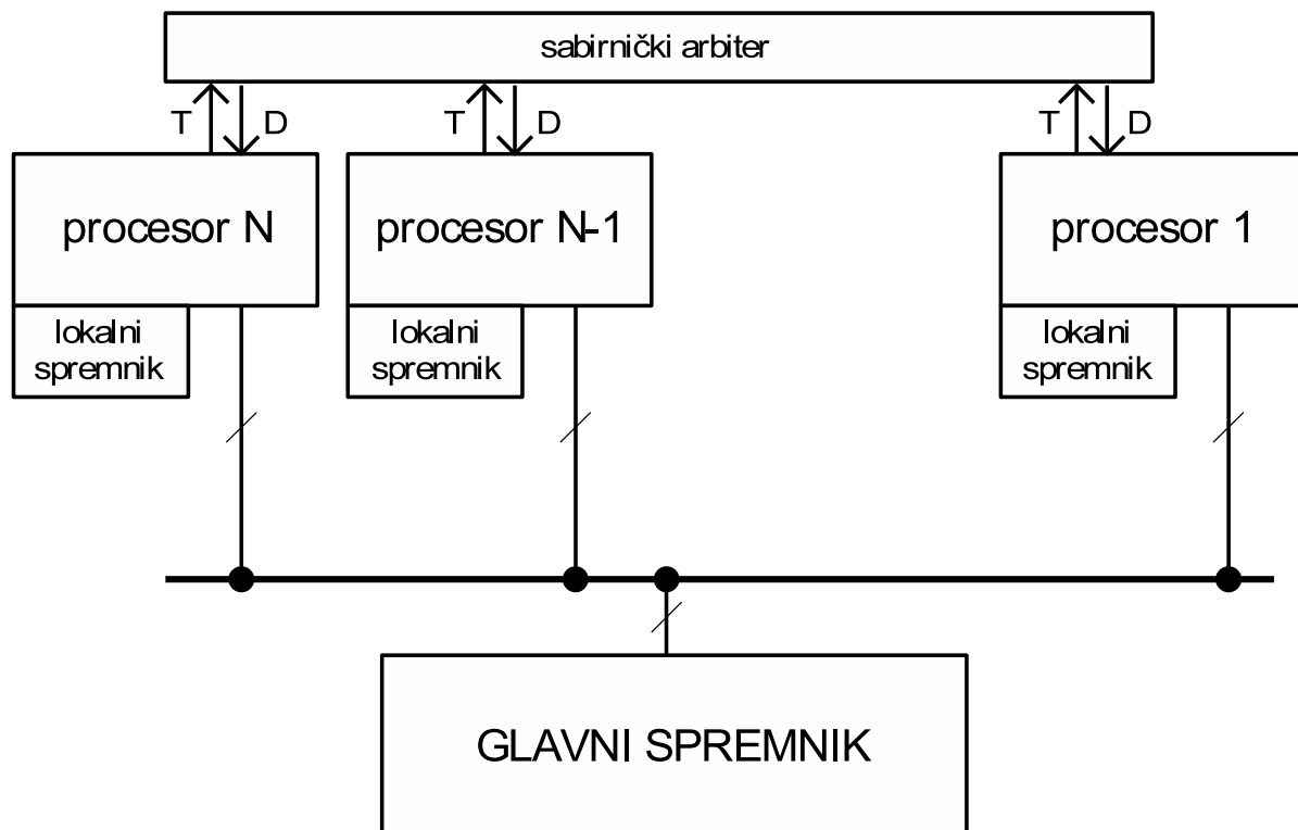
Slika 3.11. Višeprocorski sustav
