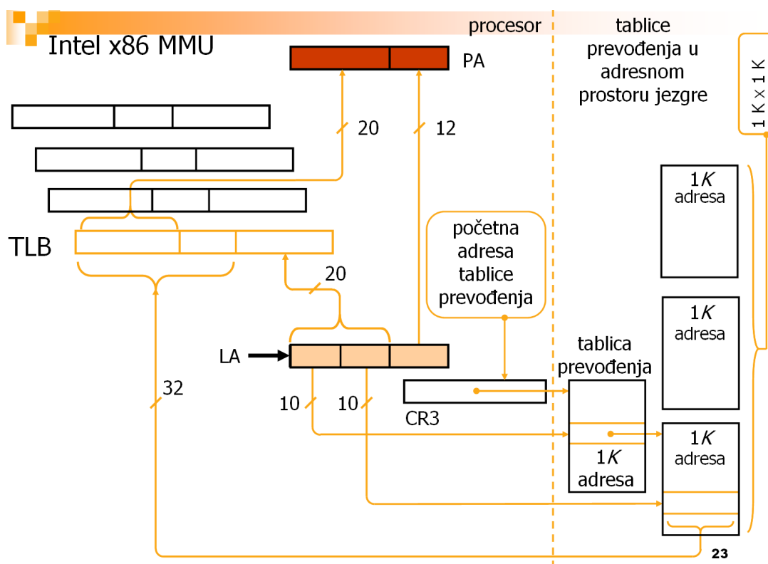
Slika 8.13. Primjer dvorazinske organizacije kod x86 arhitekture
