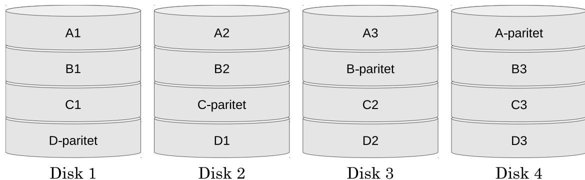
Slika 9.5. Primjer RAID 5 sustava
