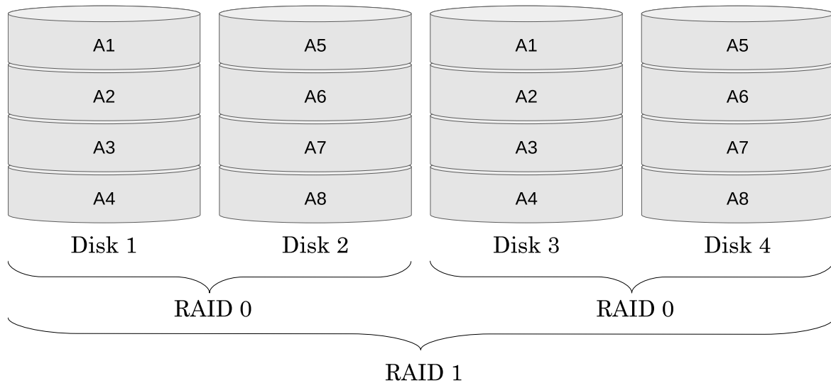
Slika 9.4. Primjer RAID 0+1 sustava
