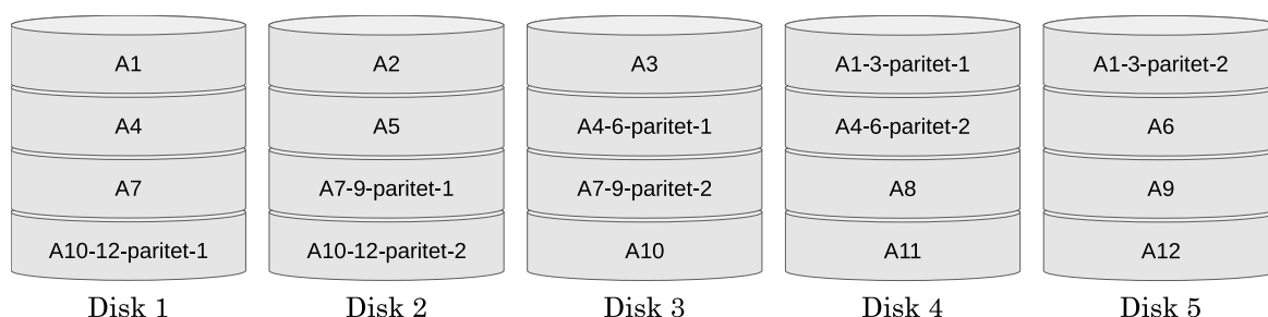
Slika 9.6. Primjer RAID 6 sustava
