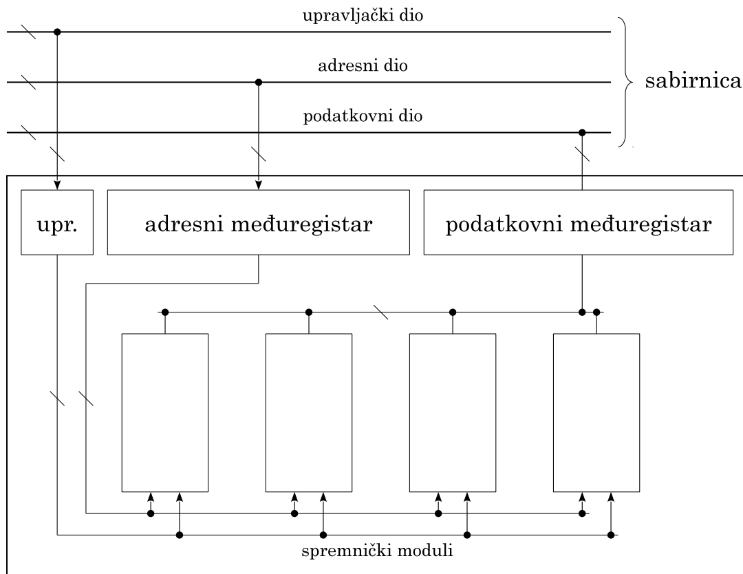
Slika 2.5. Model spremnika
