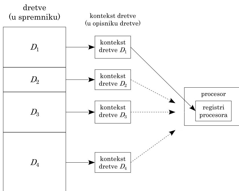
Slika 2.8. Višedretvenost na jednoprocesorskom sustavu
