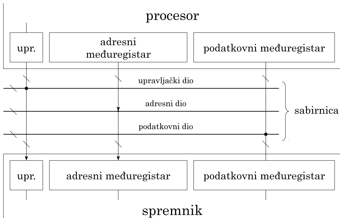
Slika 2.4. Model sabirnice
