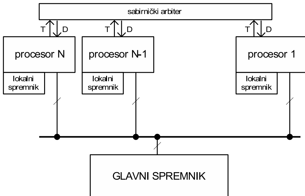
Slika 3.11. Višeprocorski sustav
