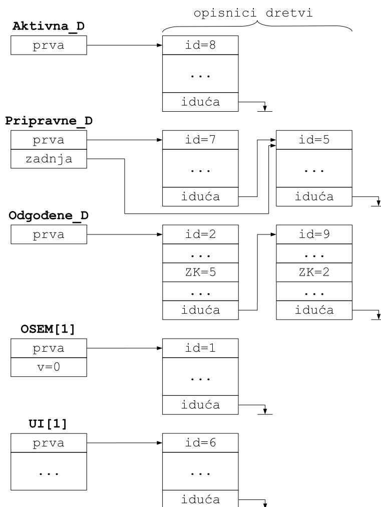
Slika 5.4. Primjer strukture podataka jezgre vizualizacijom objekata
