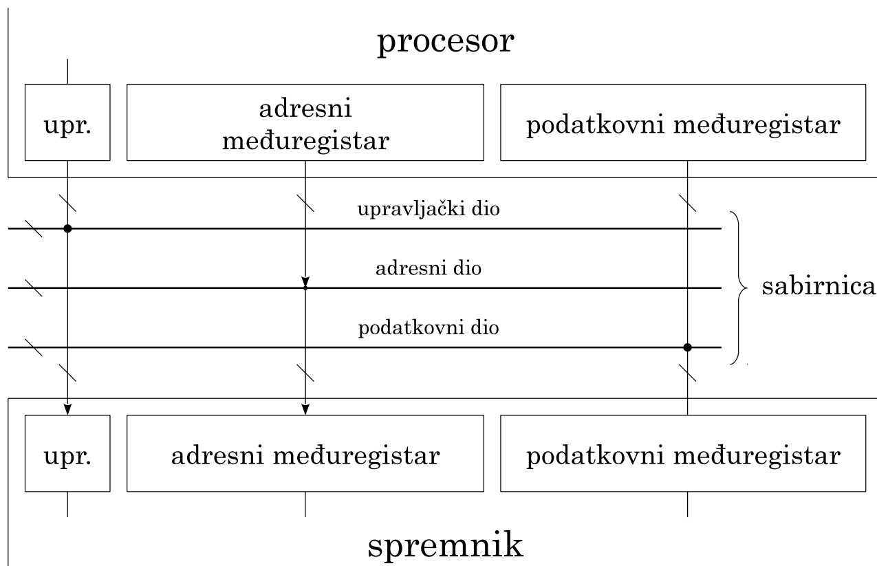
Slika 2.4. Model sabirnice
