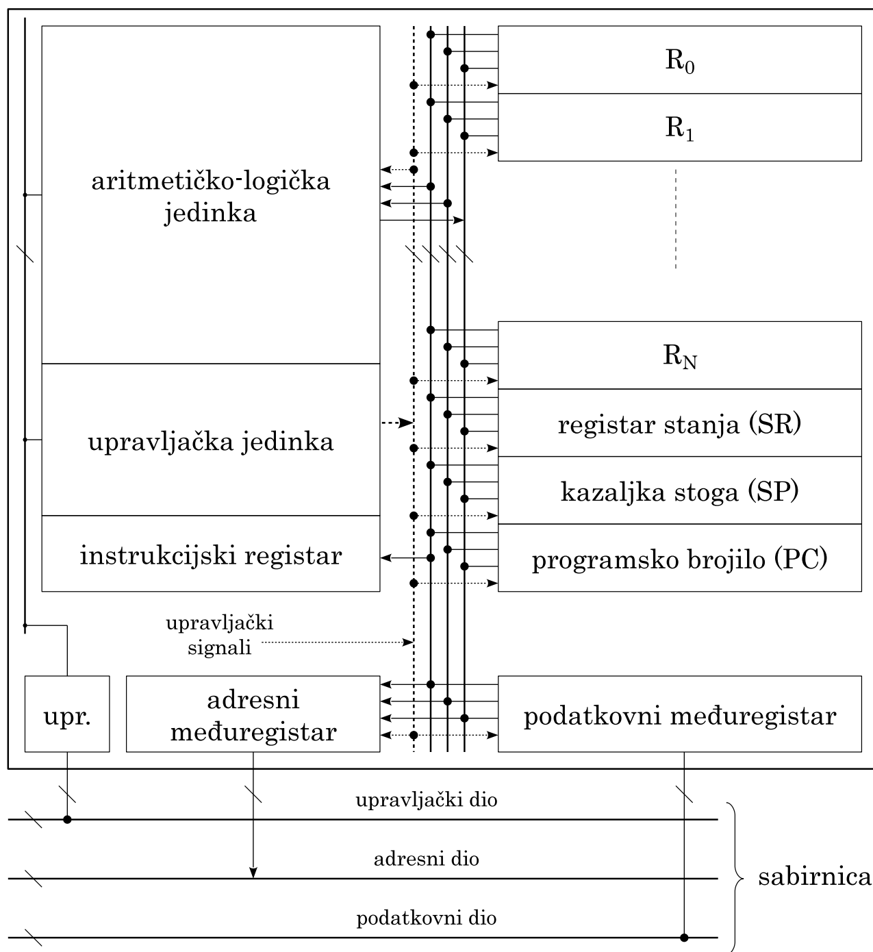
Slika 2.6. Model procesora
