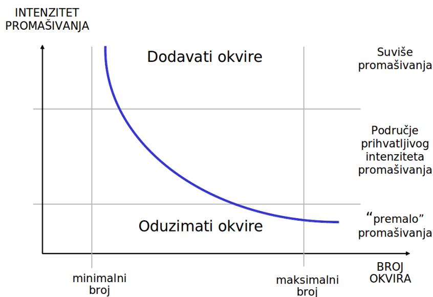
Slika 8.19. Dodjela okvira prema intenzitetu promašaja
