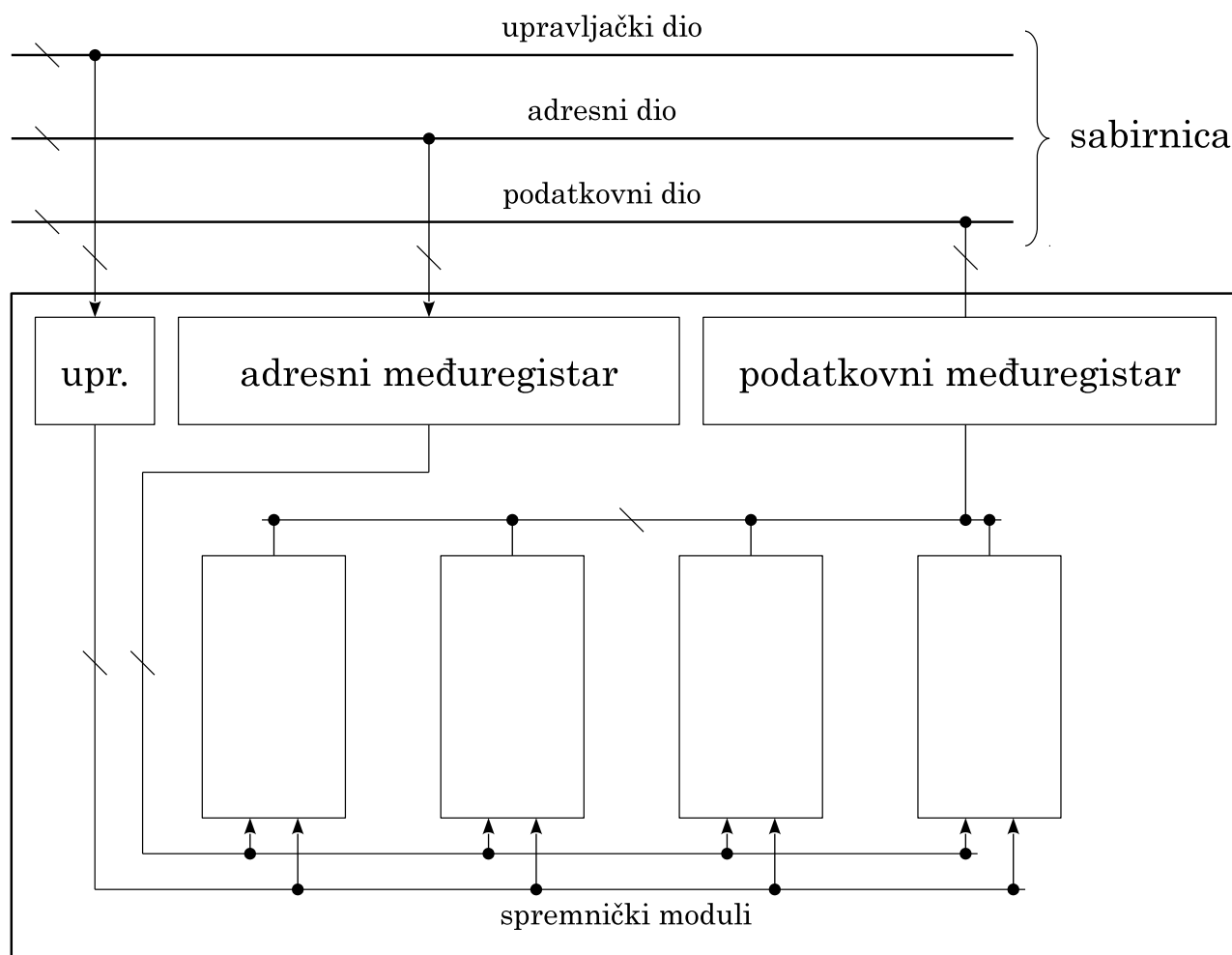
Slika 2.5. Model spremnika
