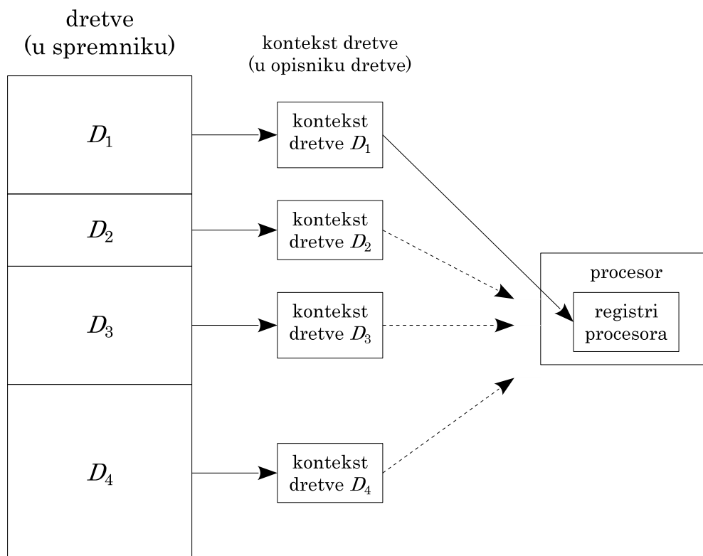
Slika 2.8. Višedretvenost na jednoprocesorskom sustavu
