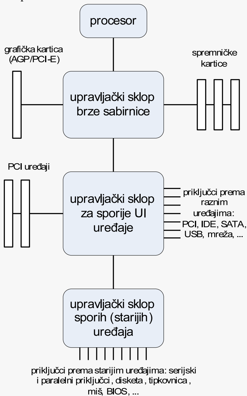
Slika 2.2. Primjer modela računala
