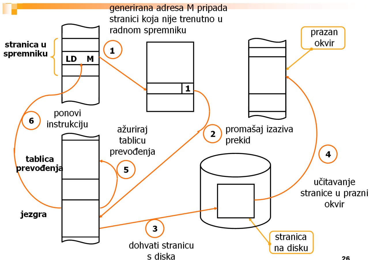
Slika 8.17. Operacije po promišaju
