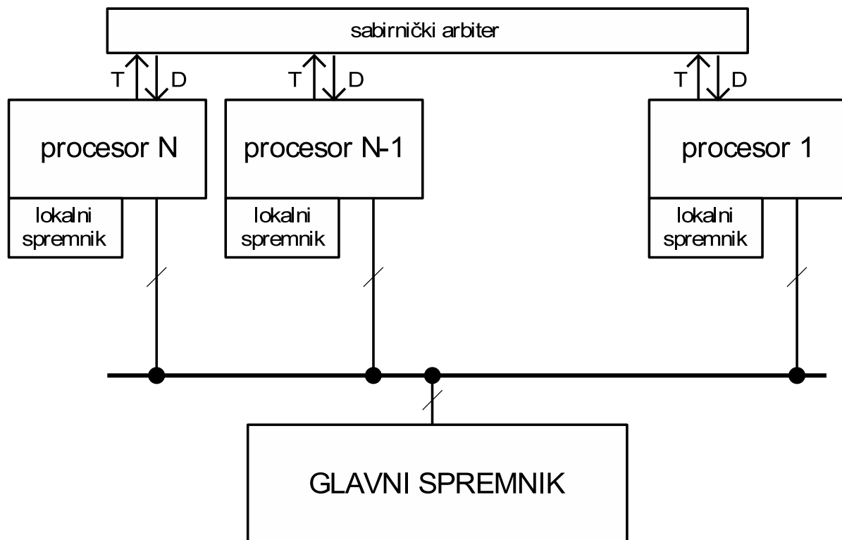
Slika 3.11. Višeprocorski sustav
