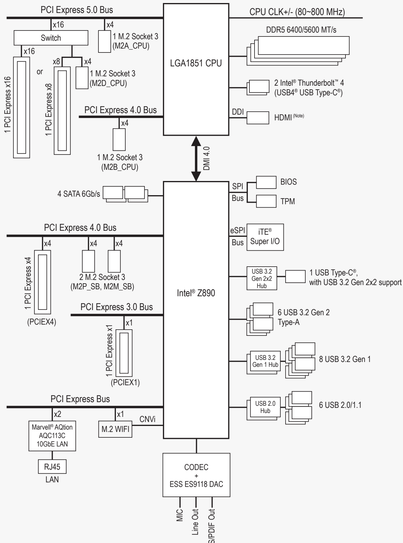
Slika 2.3. Primjer arhitekture matične ploče Z890 AORUS MASTER (izvor: GIGABYTE)
