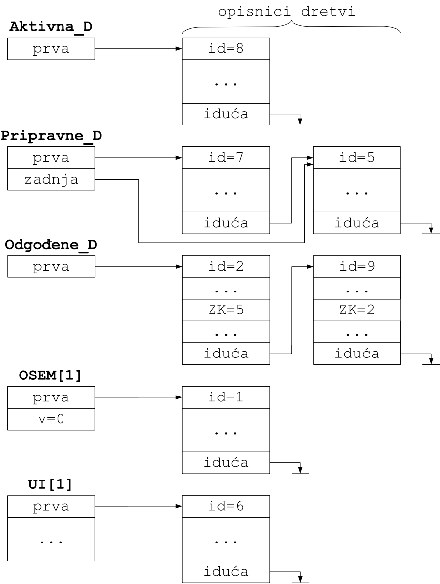
Slika 5.4. Primjer strukture podataka jezgre vizualizacijom objekata
