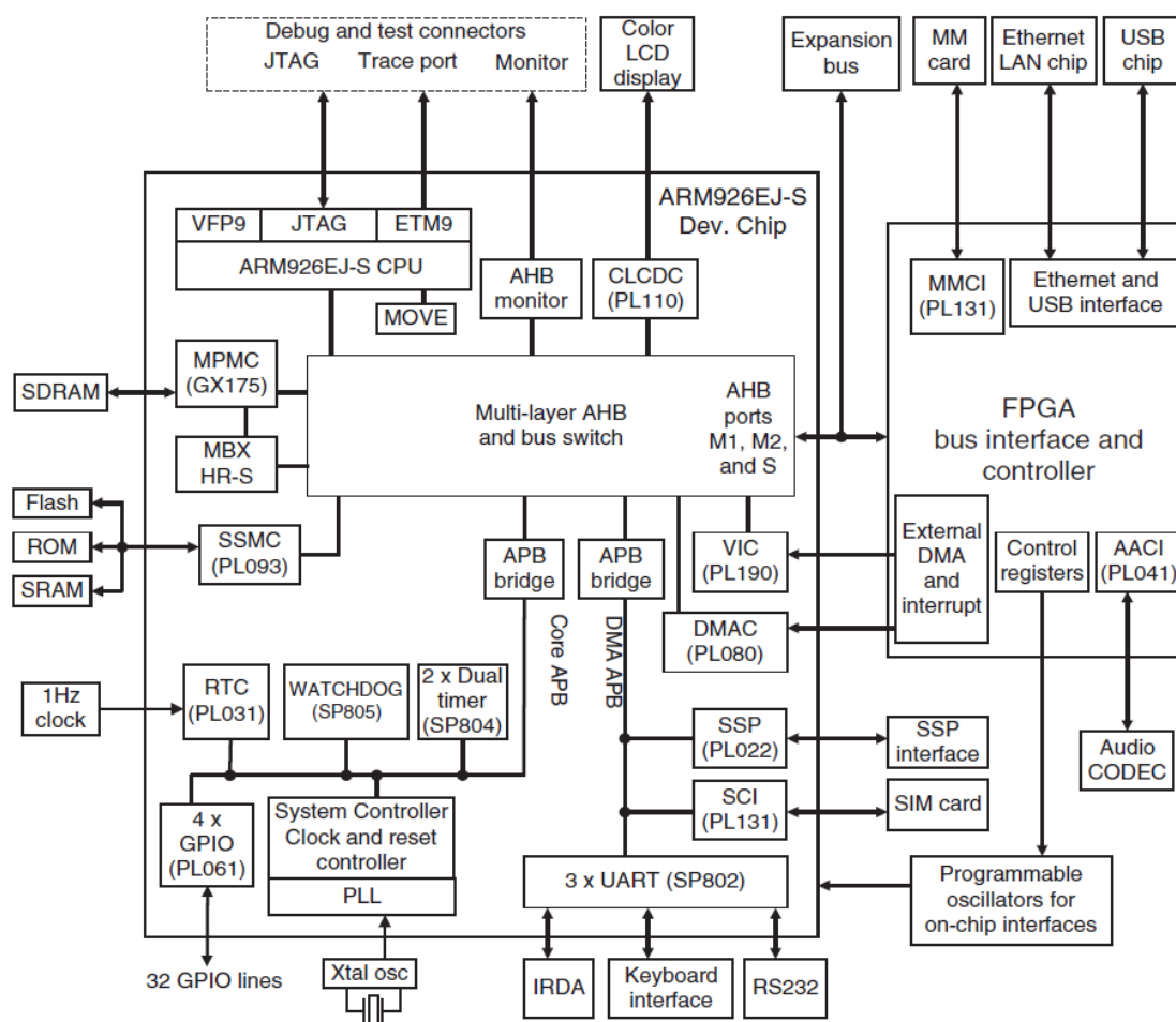
Slika A.2. Versatile PB926EJ-S razvojno okruženje
