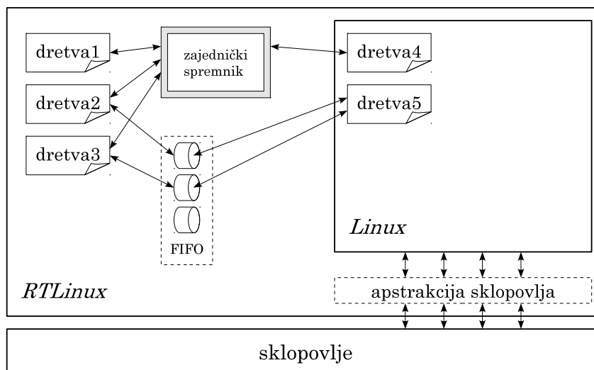
Slika 13.3. RTLinux arhitektura
