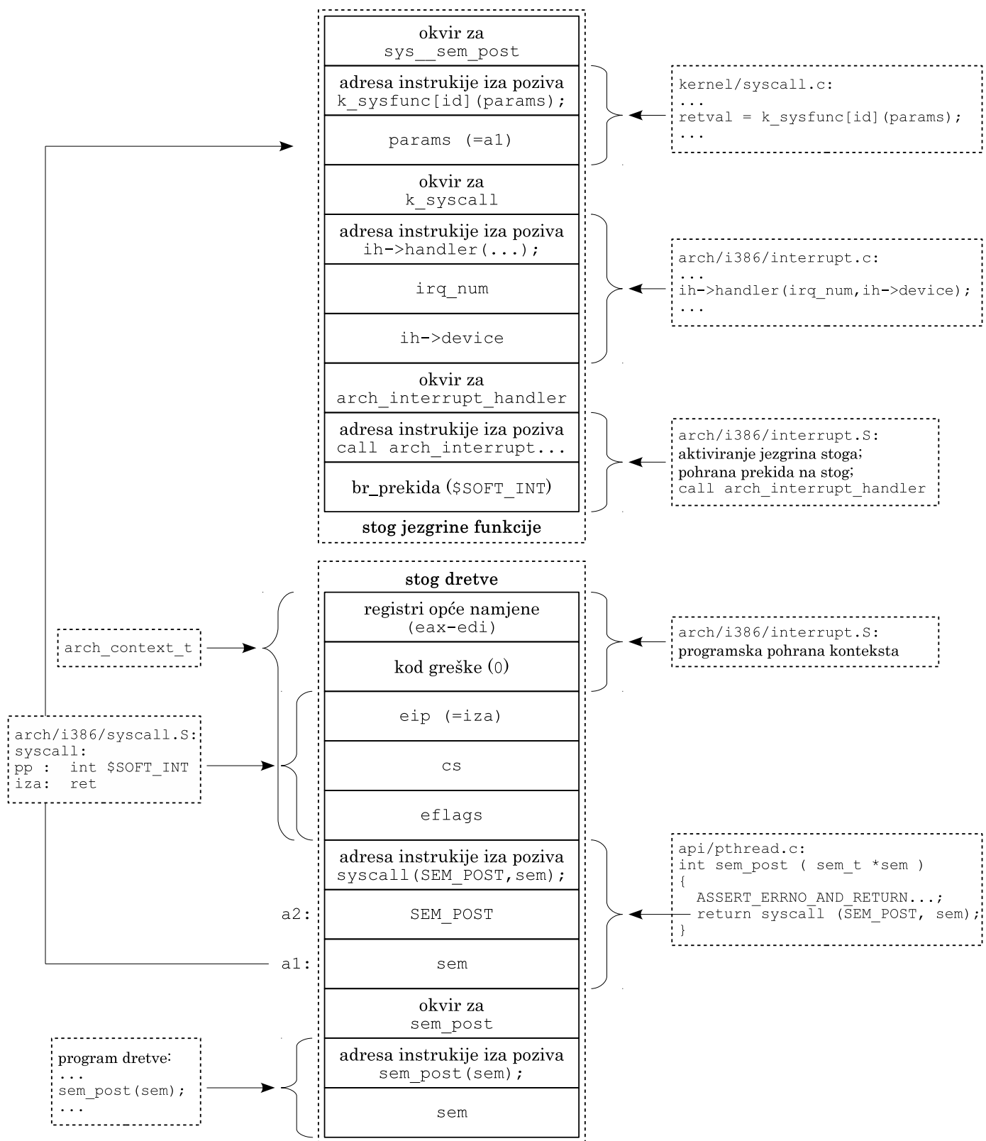
Slika 12.1. Izgled stoga pri pozivu jezgrine funkcije sem_post
