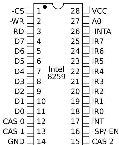
Slika 6.2. Sklop Intel 8259
