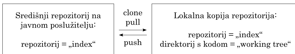
Slika B.1. Središnji i lokalni git repozitoriji
