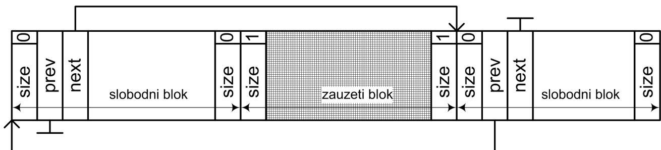
Slika 7.4. Primjer slobodnih i zauzetih blokova i njihova zaglavlja
