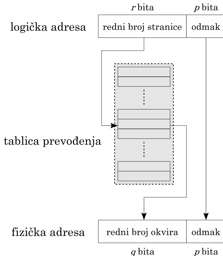
Slika 12.5. Pretvorba adresa putem tablice prevođenja
