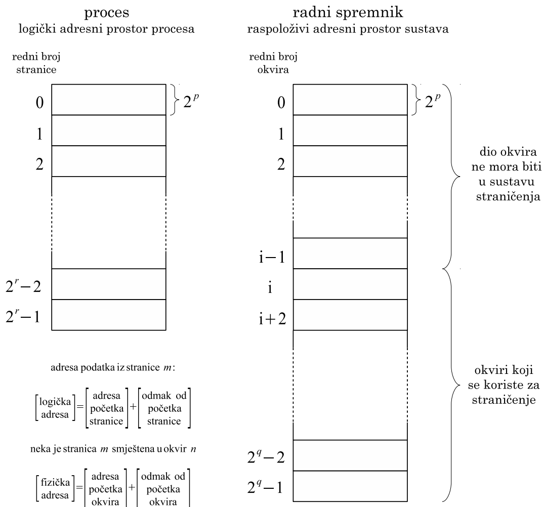
Slika 12.4. Podjela na stranice i okvire
