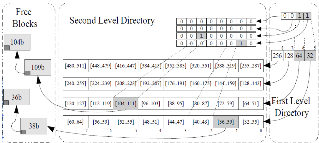
Slika 7.5. Primjer rada TLSF algoritma 2
