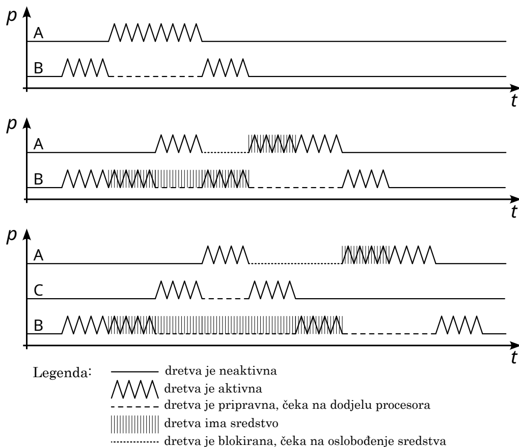
Slika E.1. Problem inverzije prioriteta
