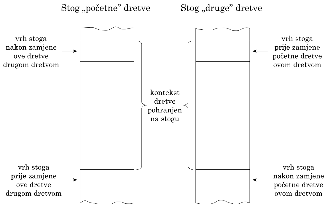
Slika 11.3. Stanje stoga prije i poslije zamjene dretvi
