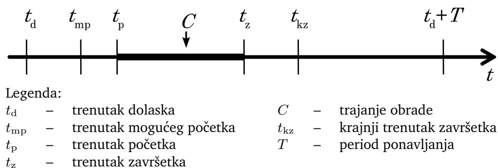
Slika 1.3. Svojstveni trenuci u životnom ciklusu jednog zadatka
