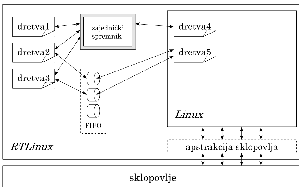
Slika 13.3. RTLinux arhitektura
