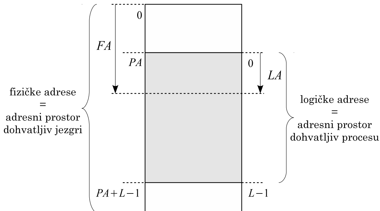
Slika 12.2. Odnos fizičke i logičke adrese
