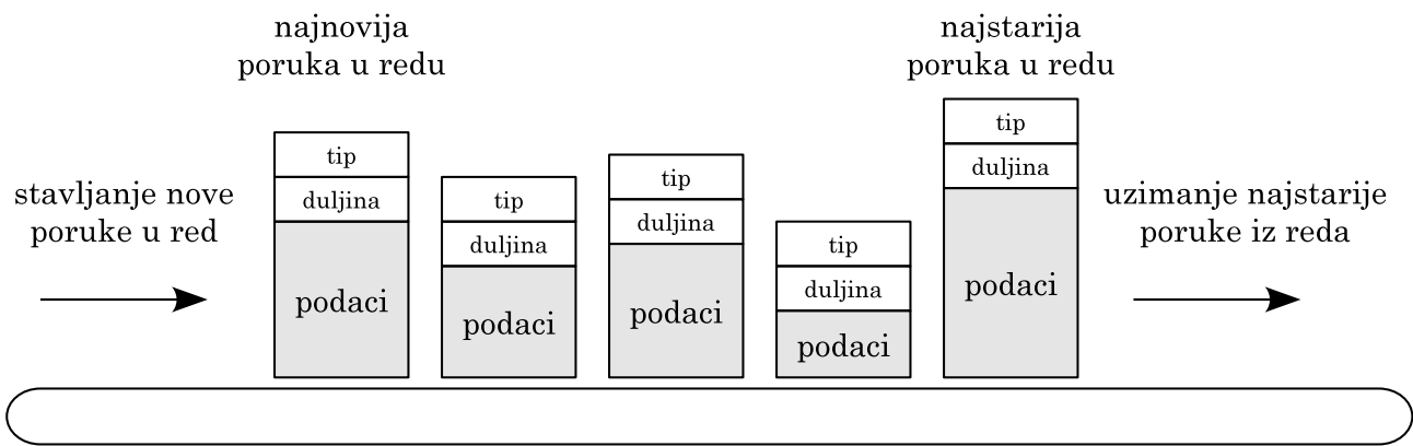
Slika 11.6. Idejni prikaz reda poruka
