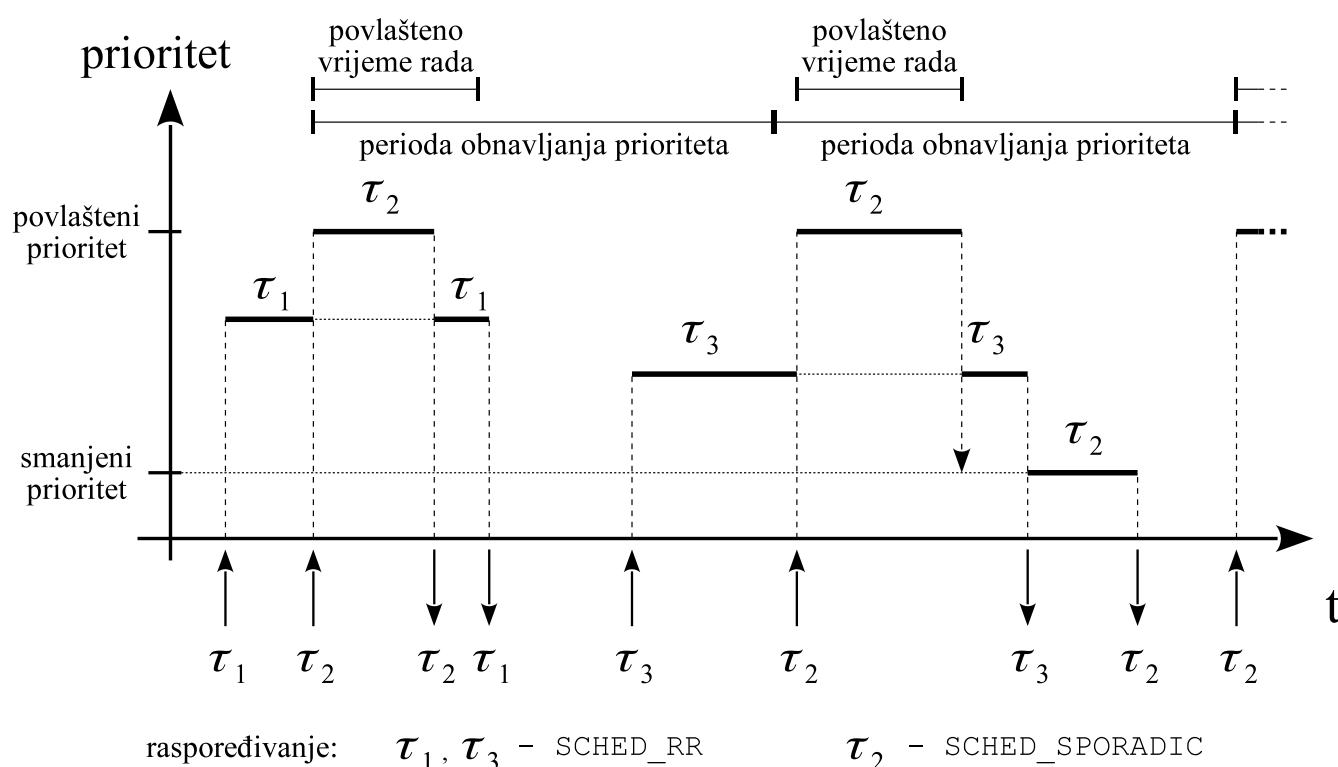
Slika F.2. Primjer sporadičnog raspoređivanja
