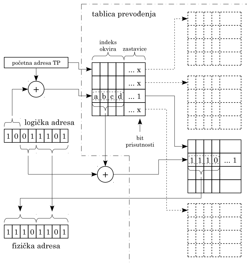
Slika 12.6. Primjer prevođenja korištenjem hijerarhijske tablice
