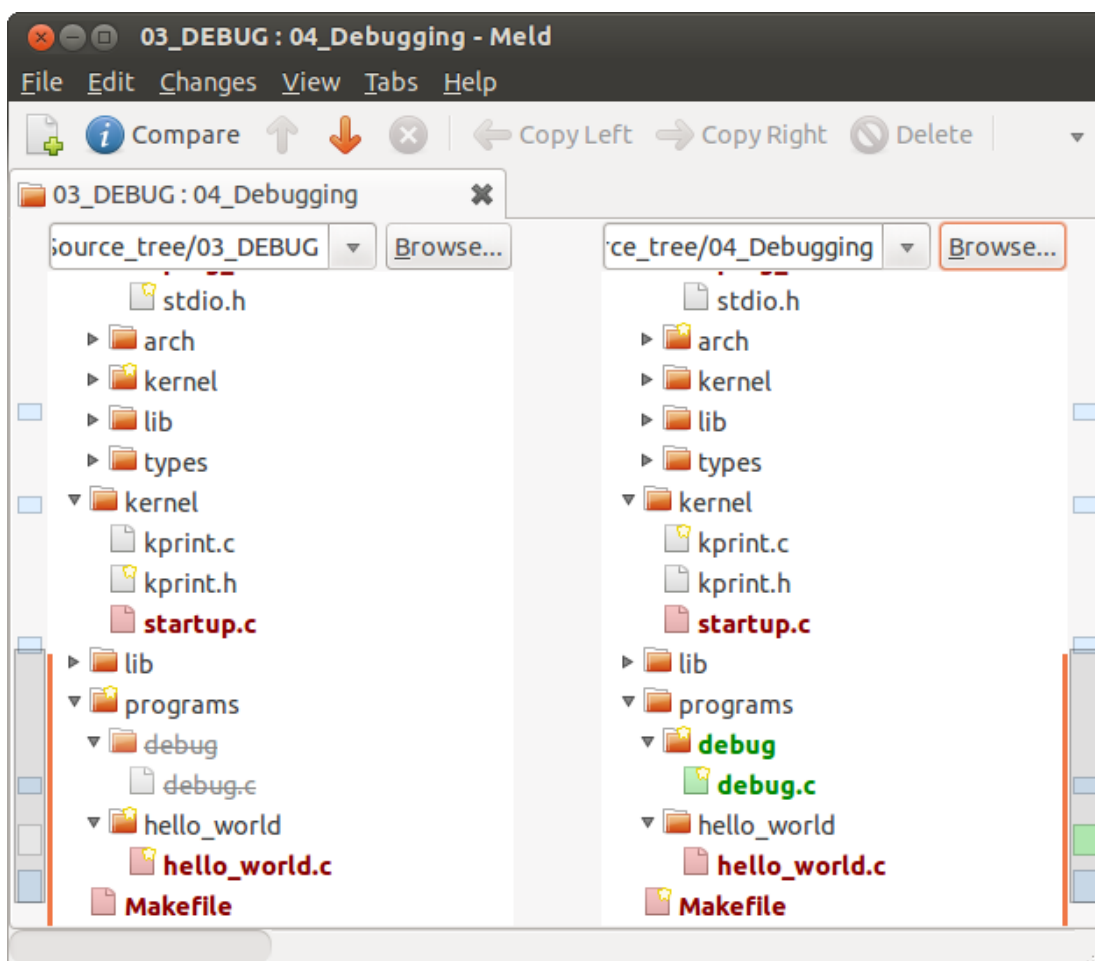
Slika 3.2. Prikaz usporedbe direktorija korištenjem programa Meld
