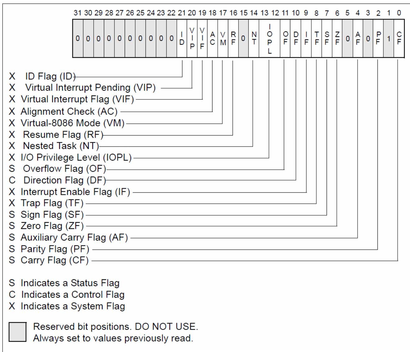
Slika 6.1. Registar stanja ( eflags )
