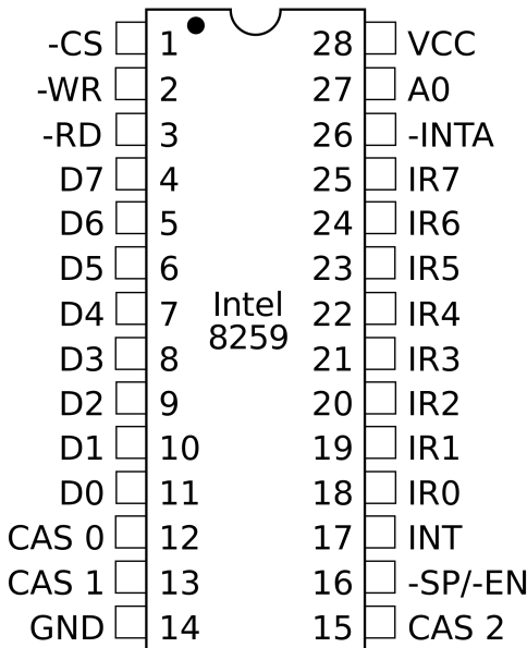
Slika 6.2. Sklop Intel 8259
