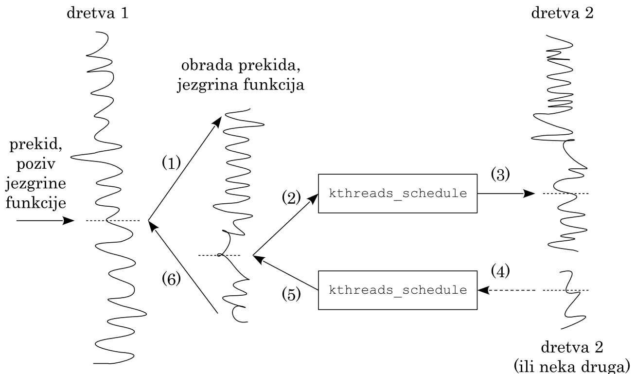
Slika 11.5. Zamjena dretve u prekidu i jezgrinoj funkciji
