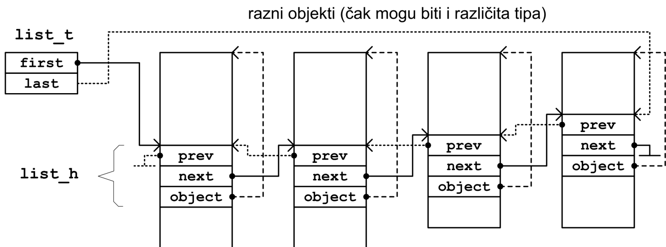
Slika 7.6. Primjer liste
