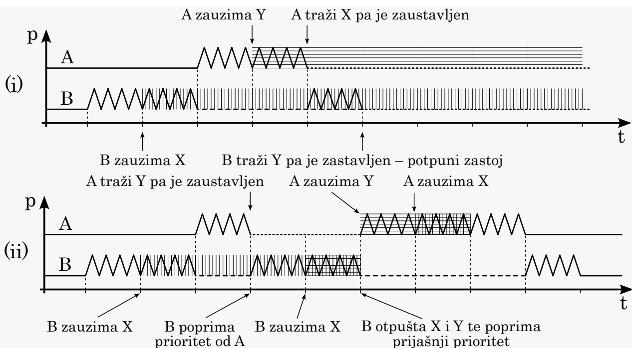
Slika E.3. Primjer potpunog zastoja i kako ga stropni protokol izbjegava
