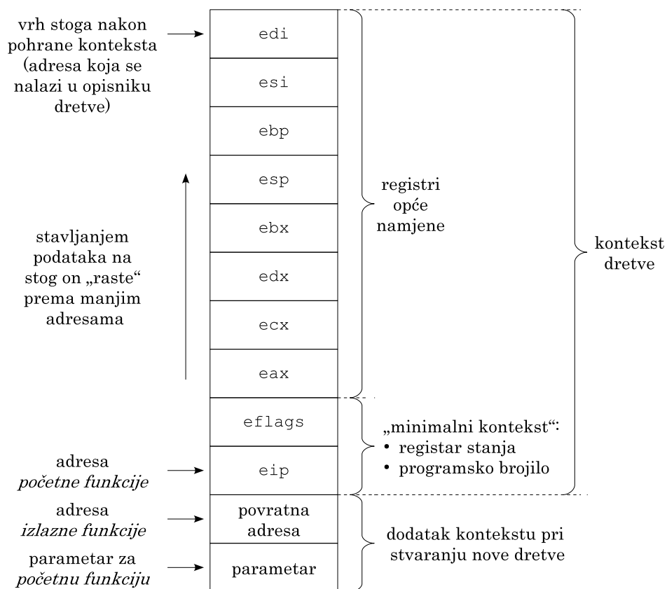
Slika 11.4. Kontekst dretve i sadržaj stoga pri stvaranju nove dretve
