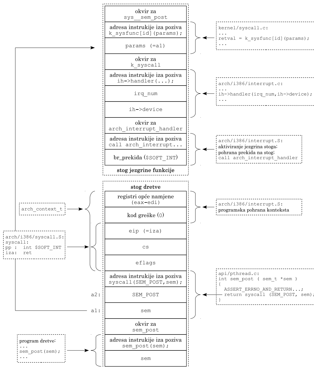
Slika 12.1. Izgled stoga pri pozivu jezgrine funkcije sem_post
