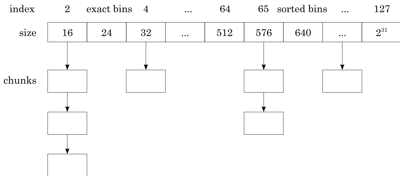
Slika 7.2. Liste slobodnih blokova kod dlmalloc algoritma
