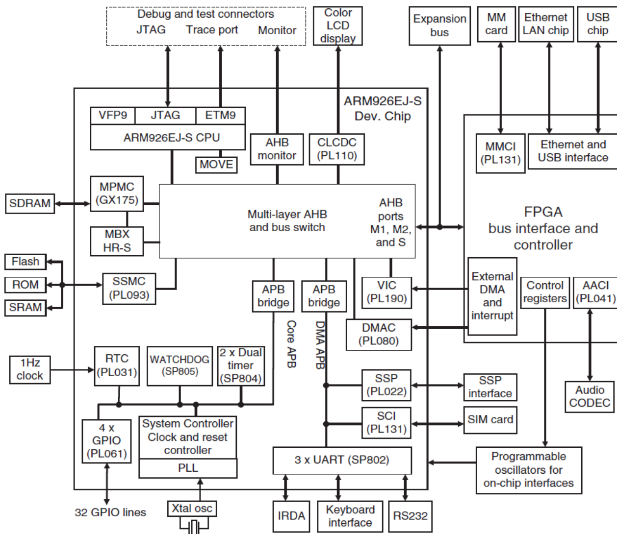
Slika A.2. Versatile PB926EJ-S razvojno okruženje
