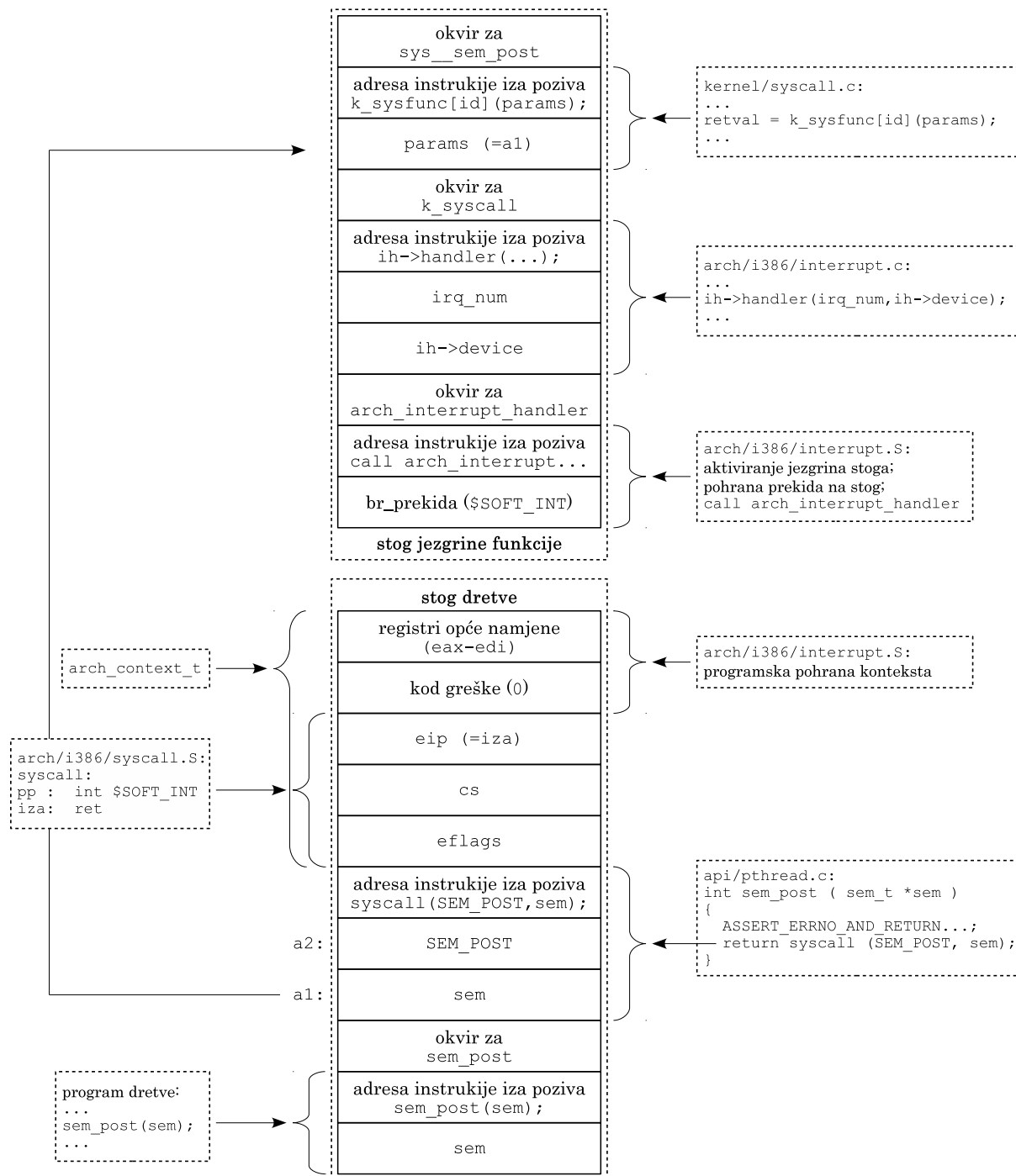
Slika 12.1. Izgled stoga pri pozivu jezgrine funkcije sem_post
