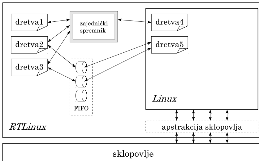
Slika 13.3. RTLinux arhitektura
