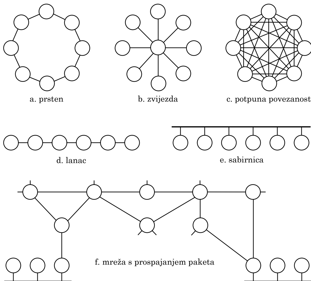
Slika 8.1. Primjeri načina spajanja računala u mreži
