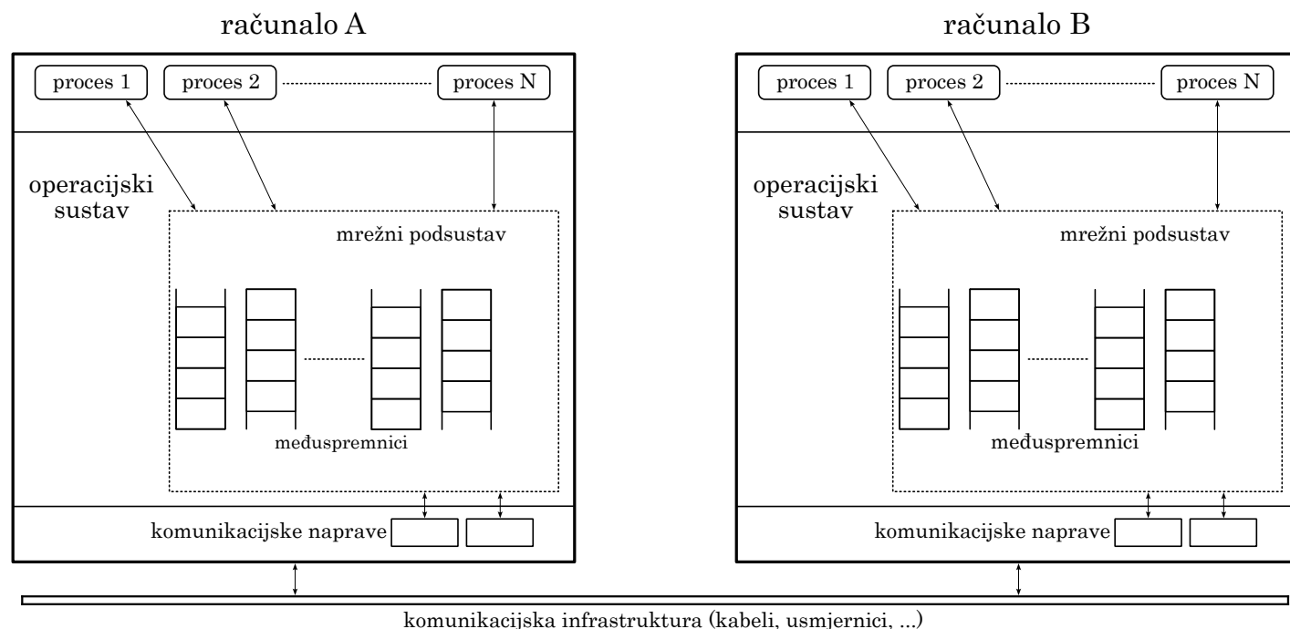
Slika 8.2. Model komunikacije u raspodijeljenom sustavu
