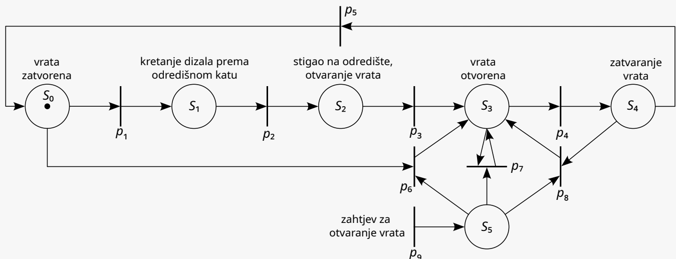
Slika 2.12. Stanja vrata dizala
