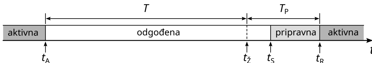
Slika 6.1. Stanje dretve pri odgodi
