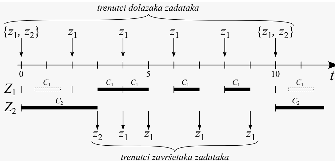
Slika 4.6. Veći prioritet zadatcima koji se rjeđe pojavljuju
