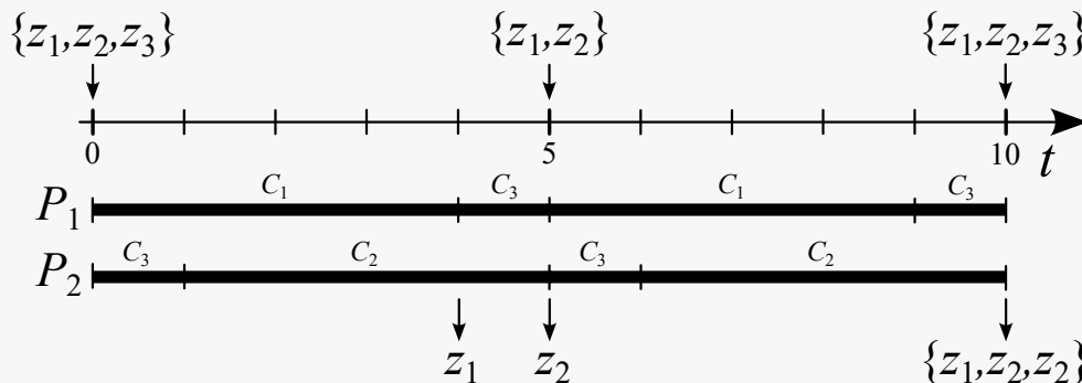
Slika 4.32. Raspored (ručni) koji zadovoljava sva ograničenja
