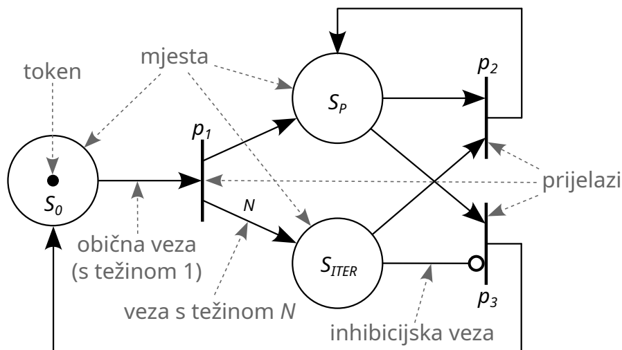
Slika 2.8. Primjer Petrijeve mreže
