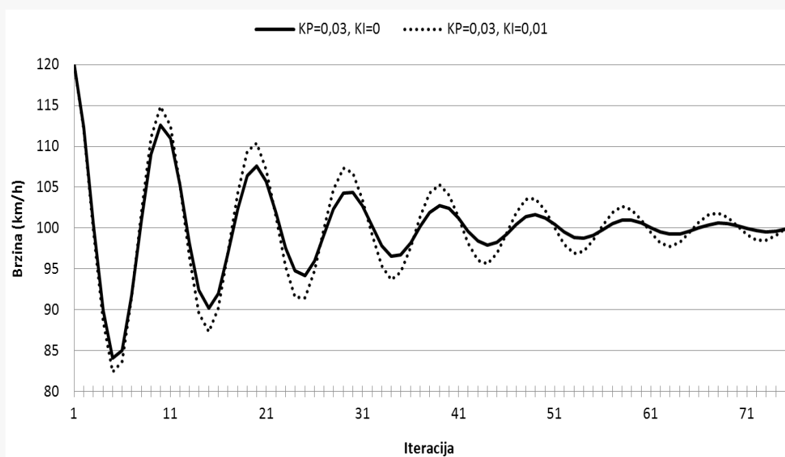
Slika 3.13. PI regulator
