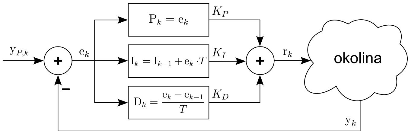
Slika 3.10. Diskretni PID regulator
