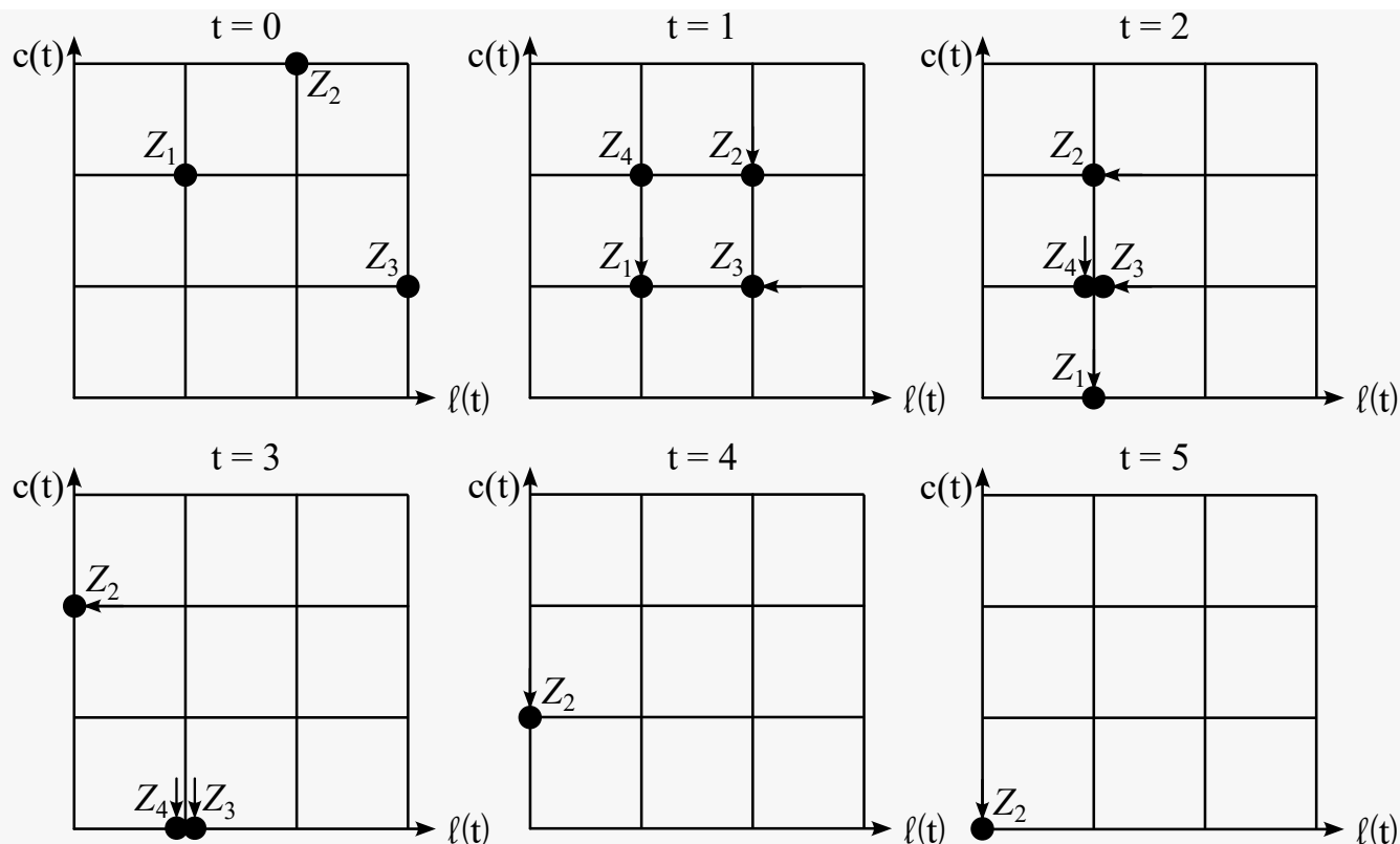
Slika 4.28. Raspoređivanje prema najmanjoj labavosti
