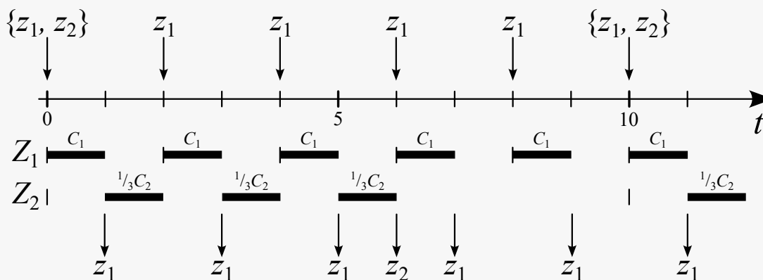
Slika 4.7. Veći prioritet zadatcima koji se češće javljaju
