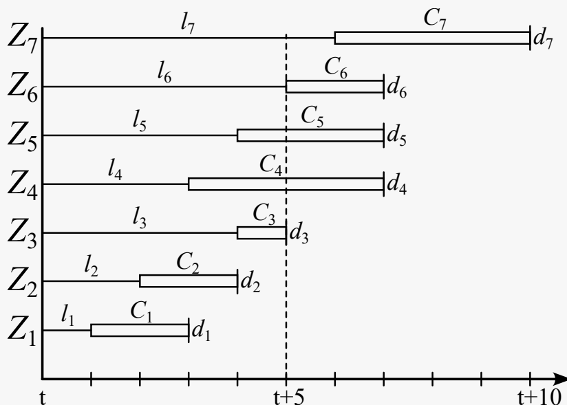
Slika 4.26. Svojstva pojedinih zadataka u trenutku t
