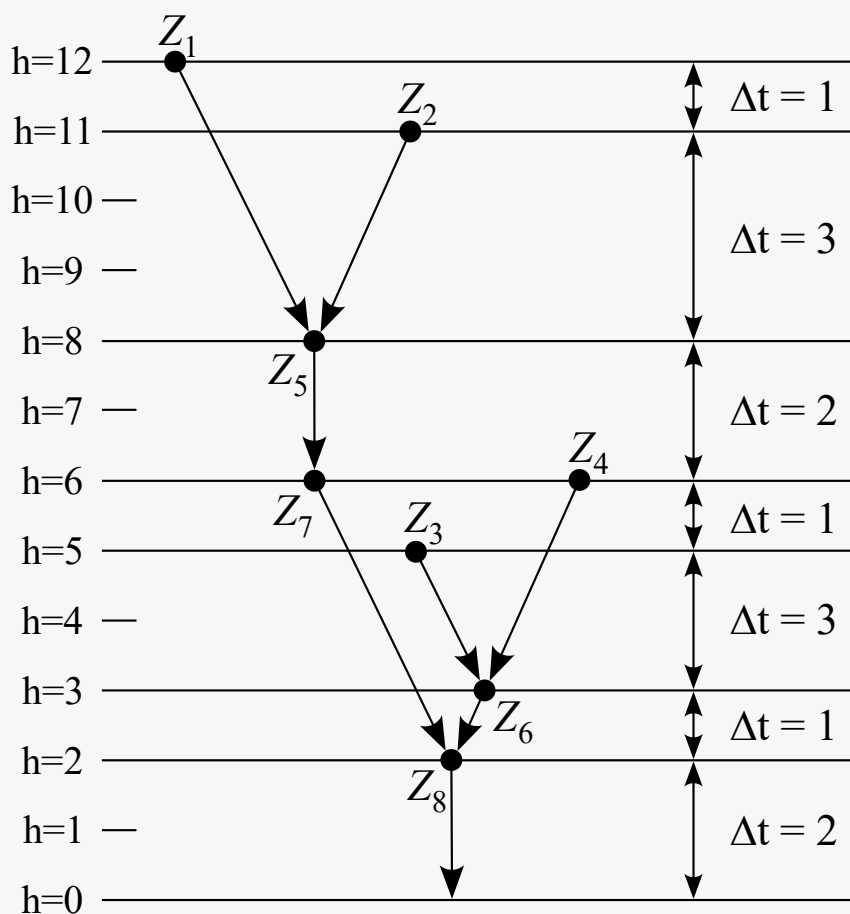
Slika 4.23. Raspoređivanje stablastom strukturom na dvoprocorskom računalu
