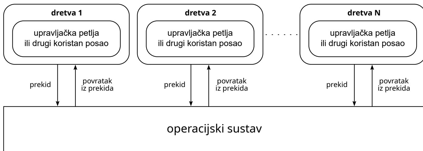
Slika 3.5. Ostvarenje upravljanja pomoću operacijskog sustava i višedretvenosti
