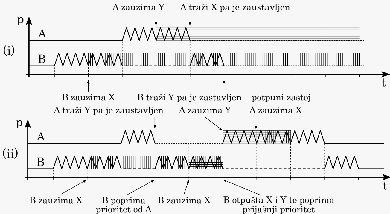
Slika 7.3. Primjer potpunog zastoja i kako ga stropni protokol izbjegava
