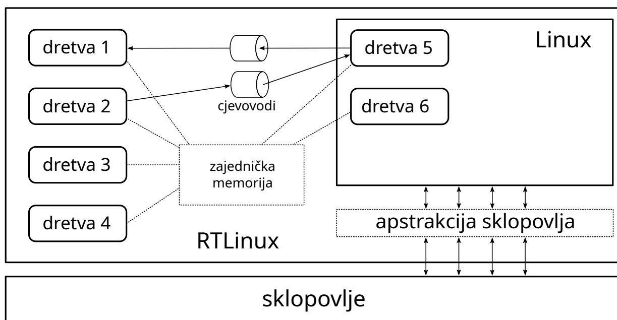
Slika 10.4. RTLinux arhitektura
