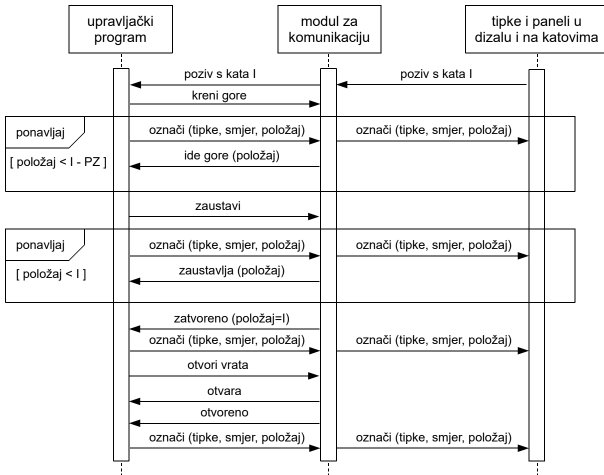
Slika 2.5. Primjer sekvencijskog UML dijagrama
