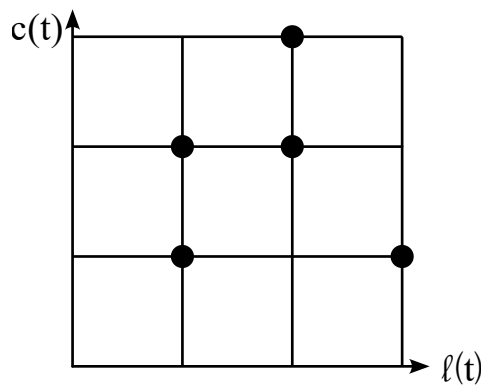
Slika 4.30. Primjer sustava u \ell - c grafu gdje RZ ne uspijeva, a NL uspijeva rasporediti sustav zadataka na dvoprocesorskom računalu
