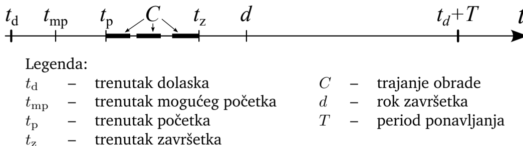
Slika 4.4. Svojstveni trenutci u životnom ciklusu jednog zadatka
