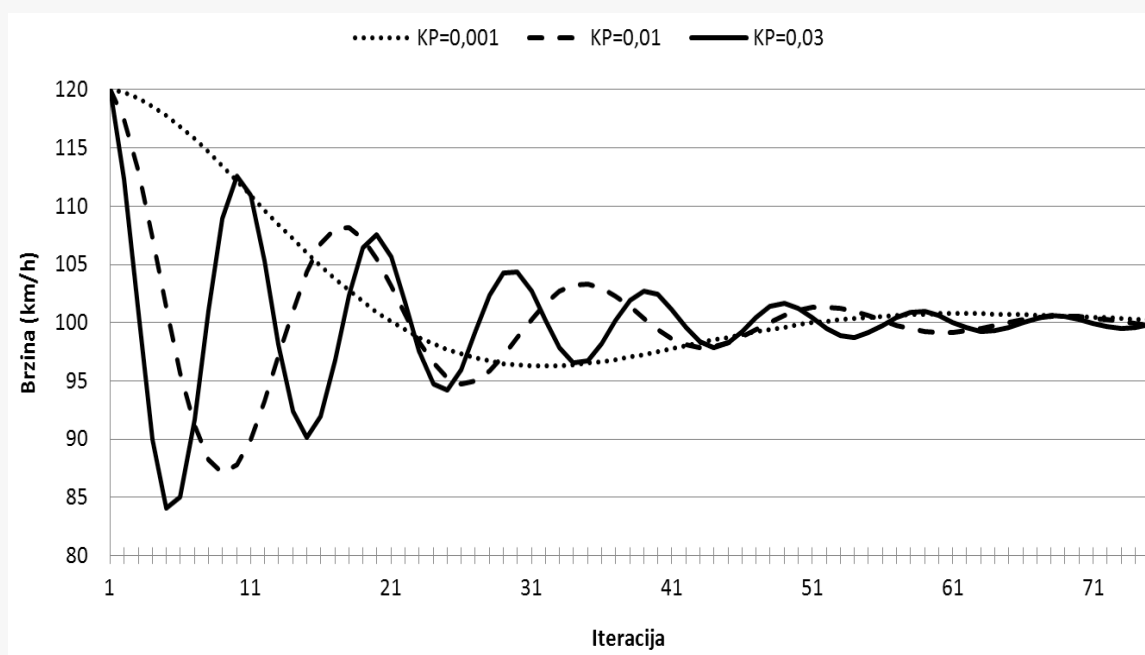
Slika 3.12. P regulator
