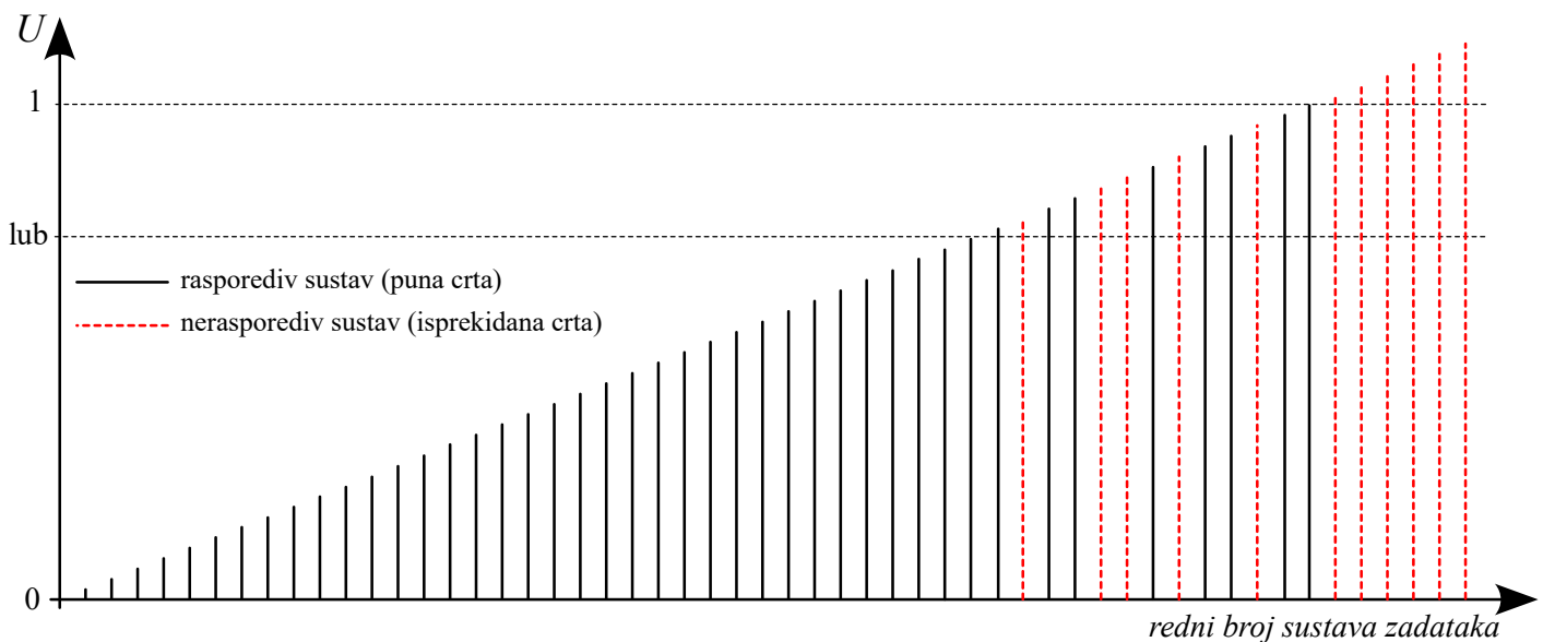
Slika 4.12. Primjeri sustava zadataka različitih faktora procesorskog iskorištenja
