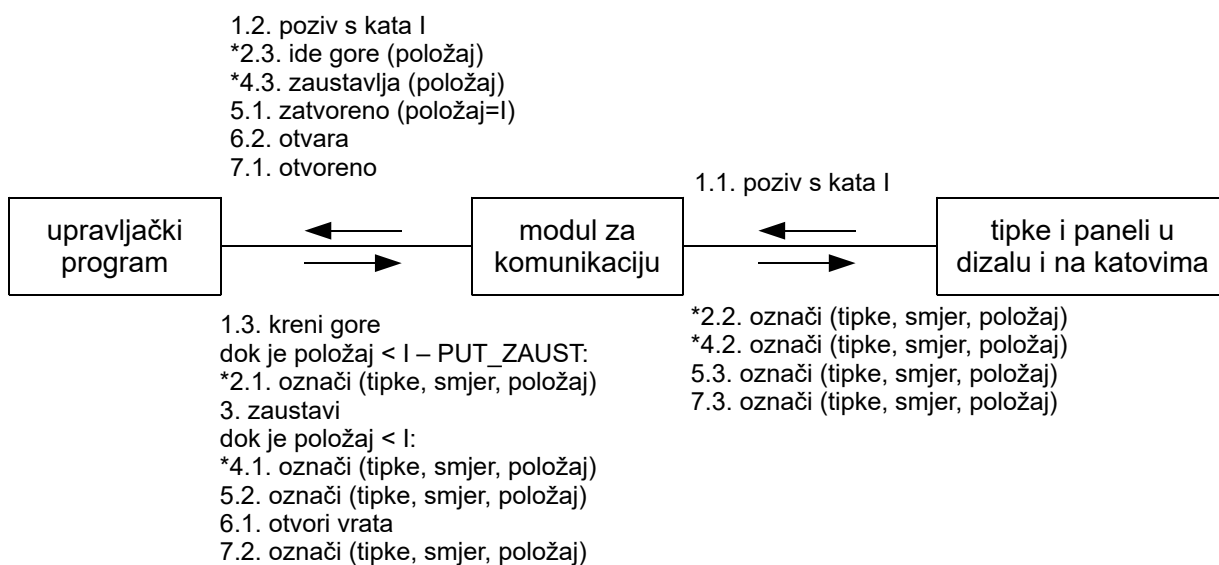
Slika 2.6. Primjer komunikacijskog UML dijagrama
