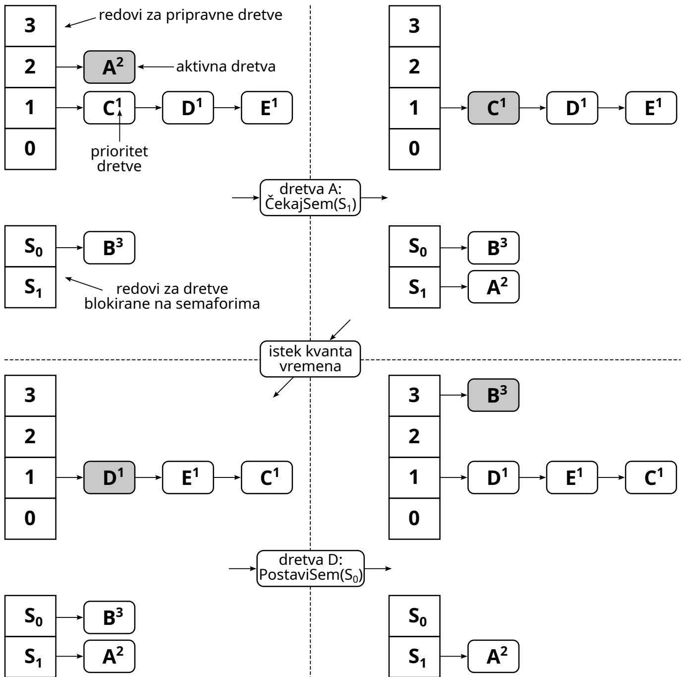
Slika 5.2. Primjeri raspoređivanja prema prioritetu i podjeli vremena
