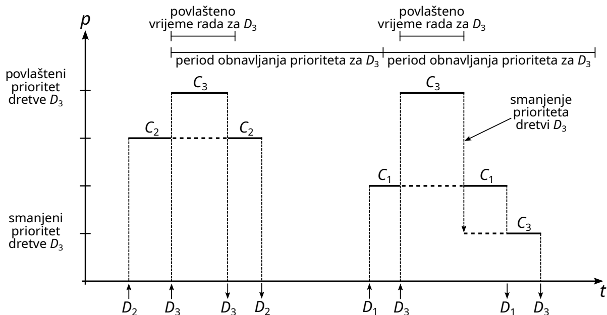
Slika 5.3. Primjer sporadičnog raspoređivanja
