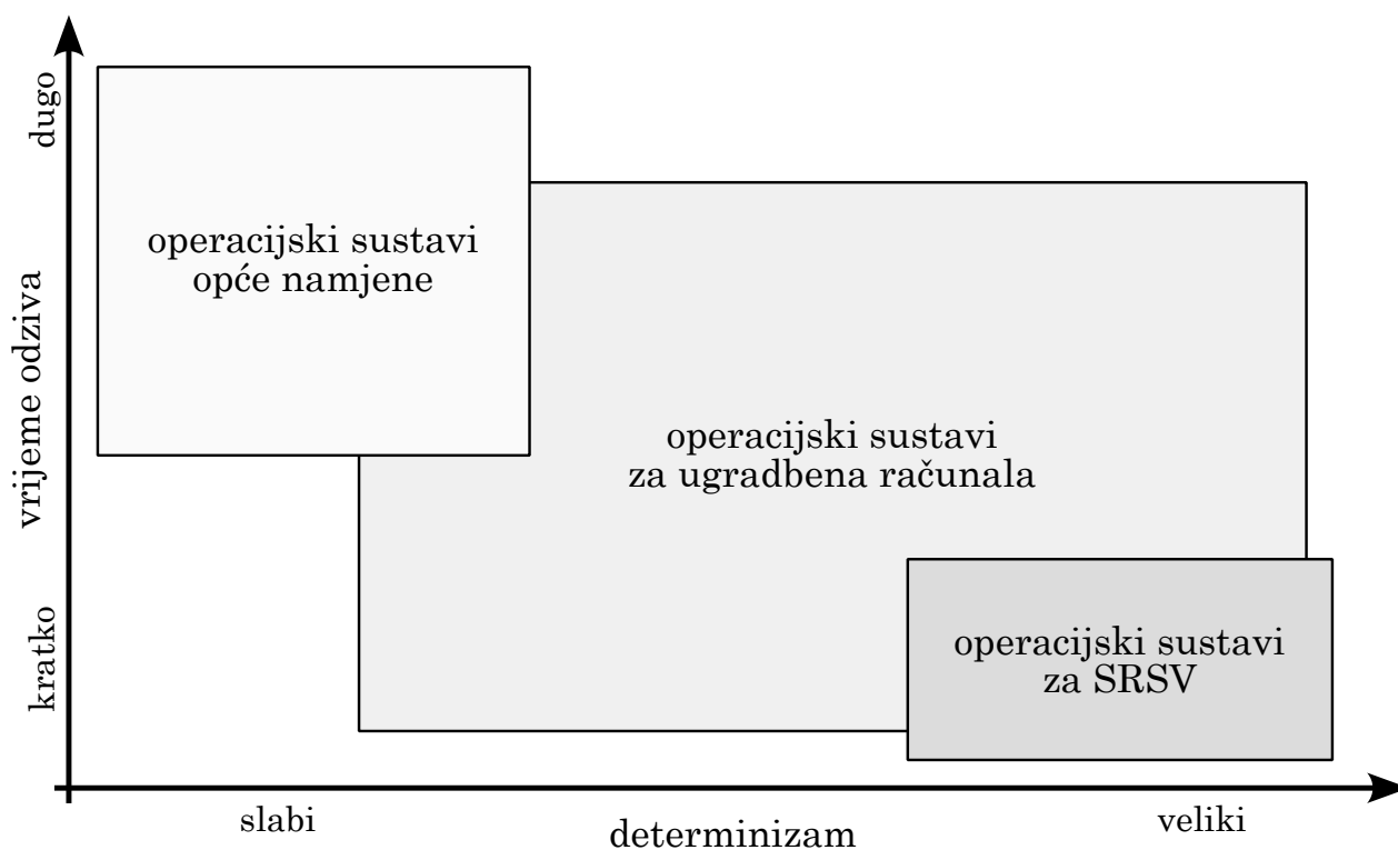
Slika 10.2. Vremenska svojstva različitih sustava
