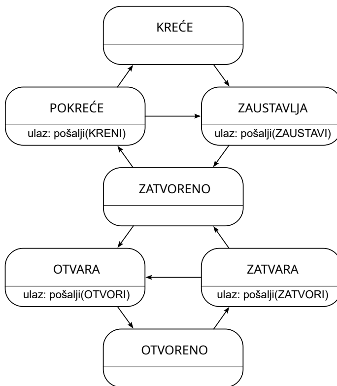
Slika 2.7. Primjer UML dijagrama stanja
