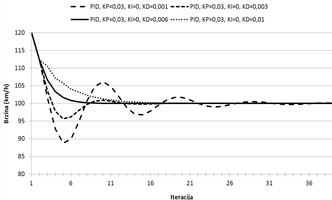
Slika 3.14. PD regulator
