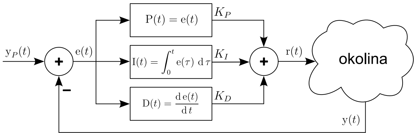
Slika 3.7. PID regulator
