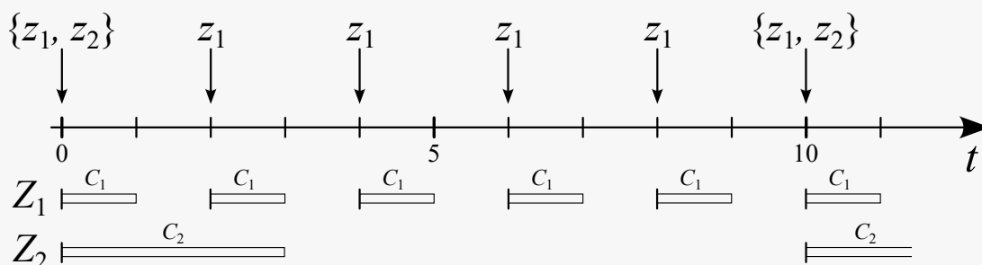
Slika 4.5. Sustav s dva zadatka
