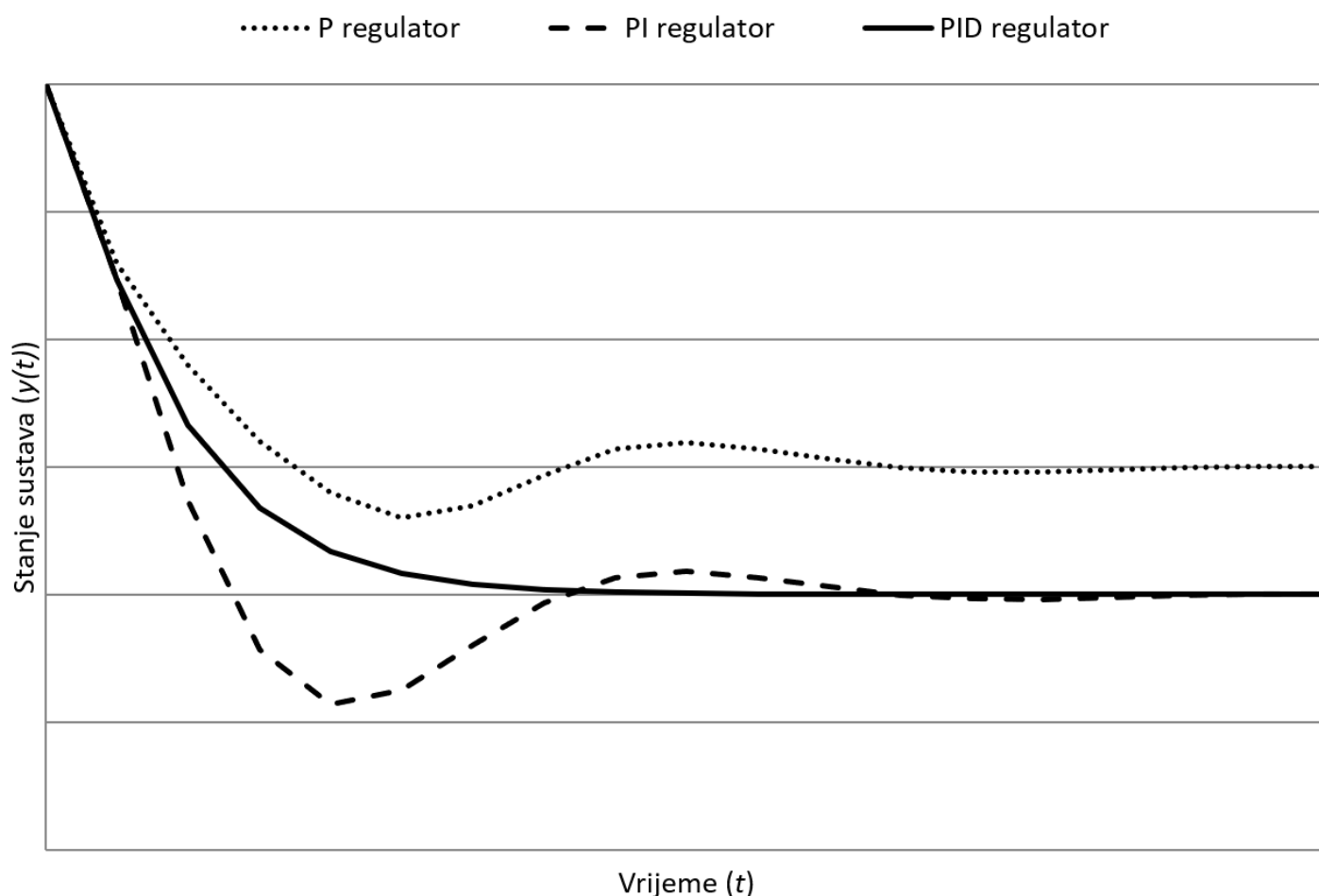
Slika 3.9. Načelni utjecaj komponenata PID regulatora
