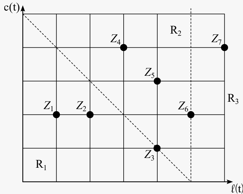
Slika 4.25. Podjela \ell - c grafa u područja pri određivanju zalihosti
