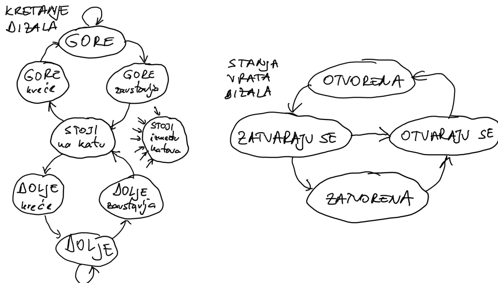
Slika 2.2. Dijagram stanja dizala, vrata u dizalu i vrata na katu
