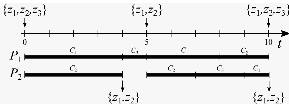
Slika 4.31. NL raspoređivanje uz indeks zadatka kao drugi kriterij
