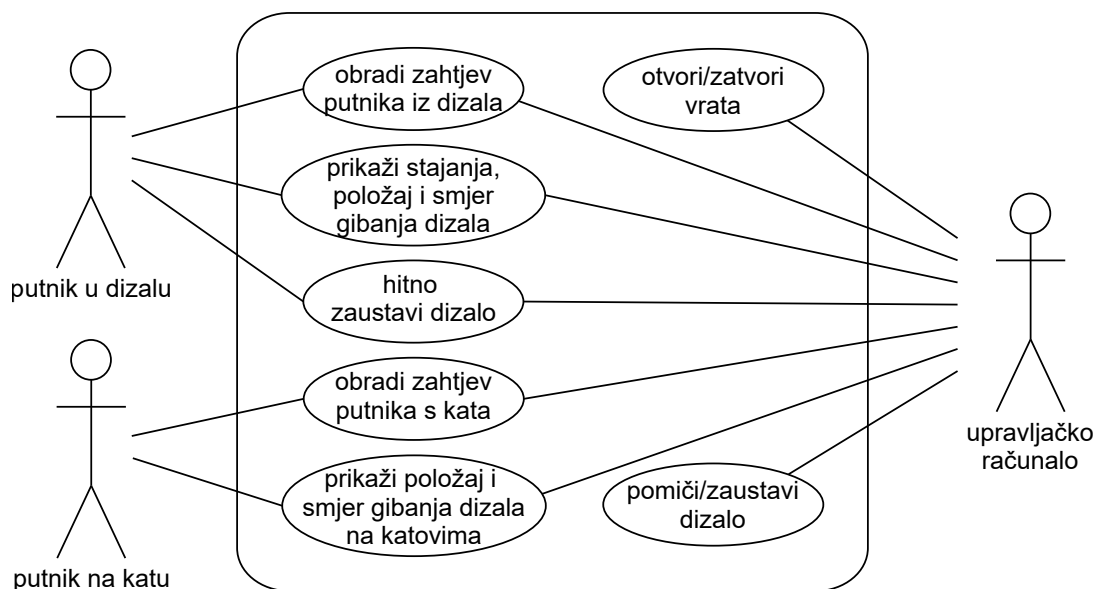
Slika 2.4. Primjer UML dijagrama obrazaca uporabe
