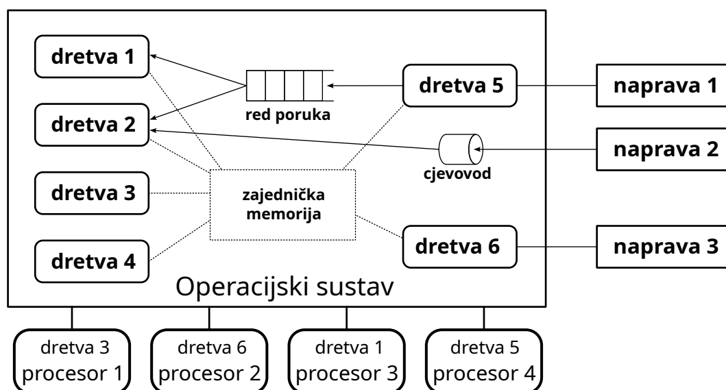
Slika 4.1. Primjer višedretvenog upravljačkog sustava
