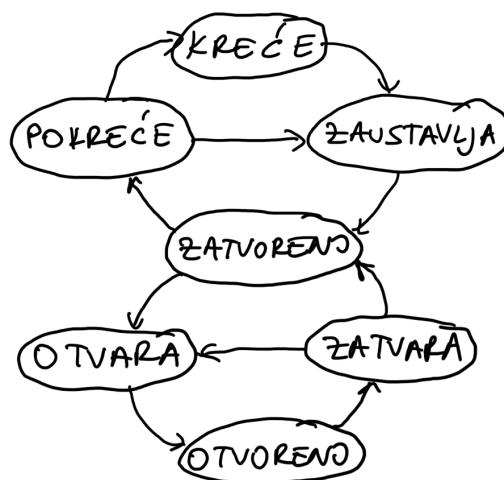
Slika 2.3. Dijagram stanja dizala, nakon spajanja
