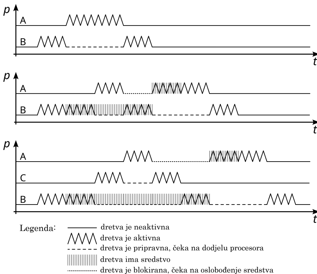
Slika 7.1. Problem inverzije prioriteta
