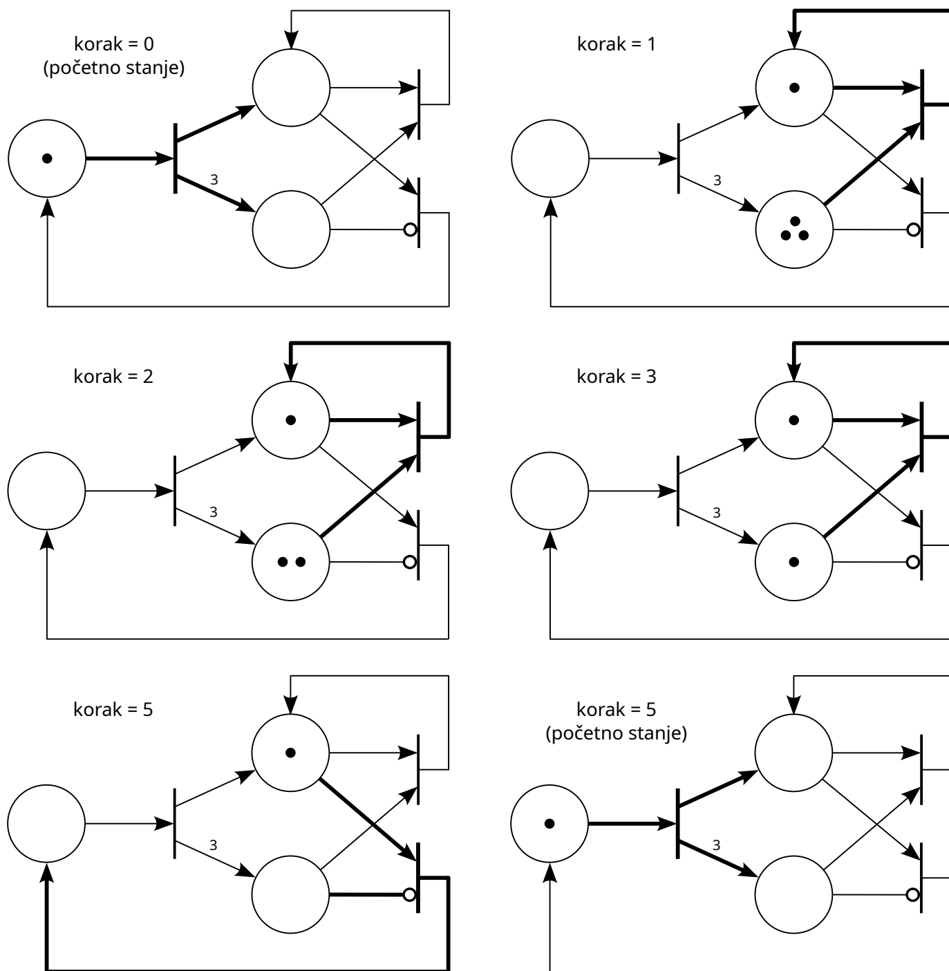
Slika 2.9. Primjer rada Petrijeve mreže
