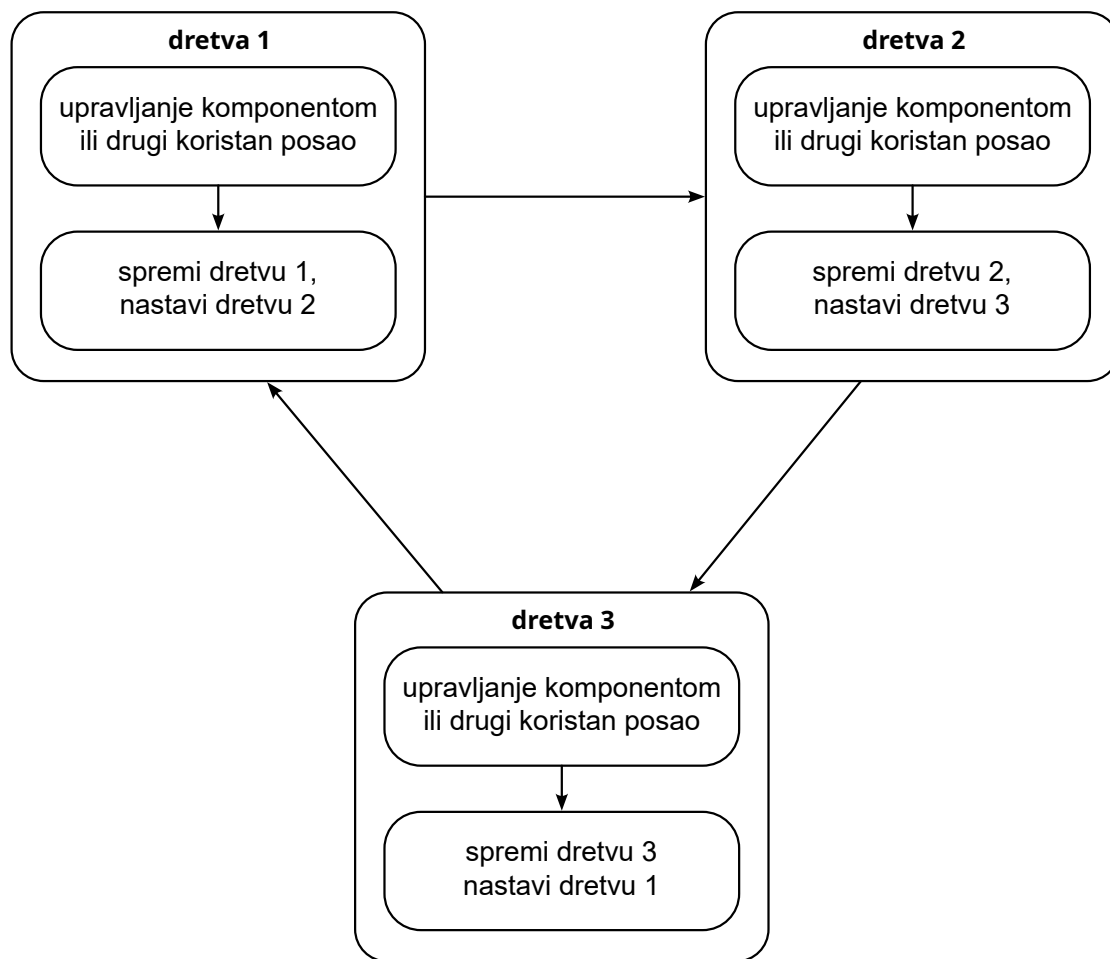
Slika 3.4. Ostvarenje upravljanja kooperativnom višedretvenošću
