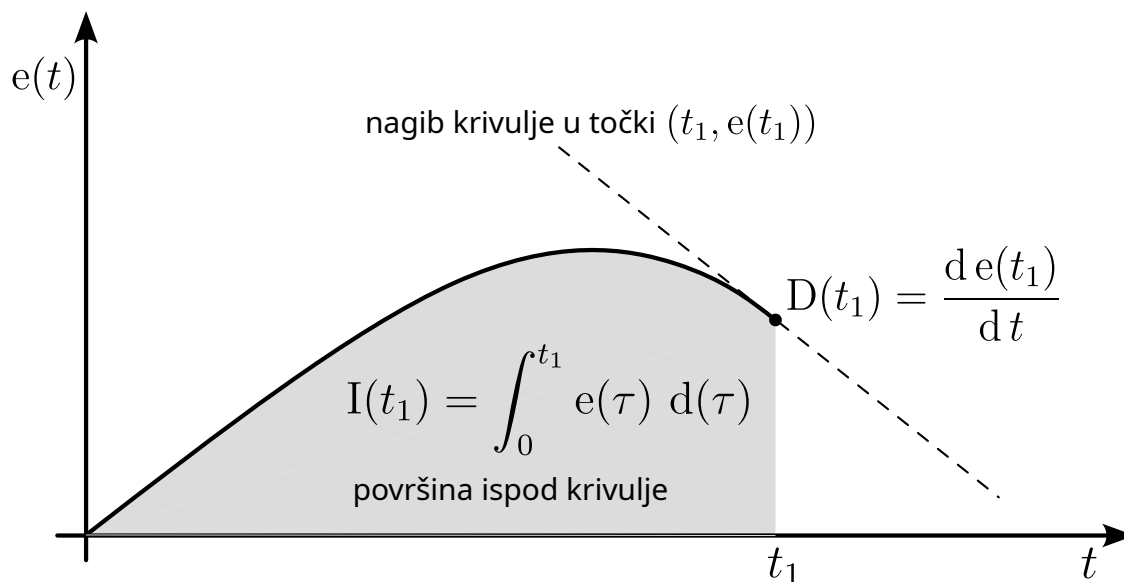
Slika 3.8. Izračunavanje integracijske i derivacijske komponente
