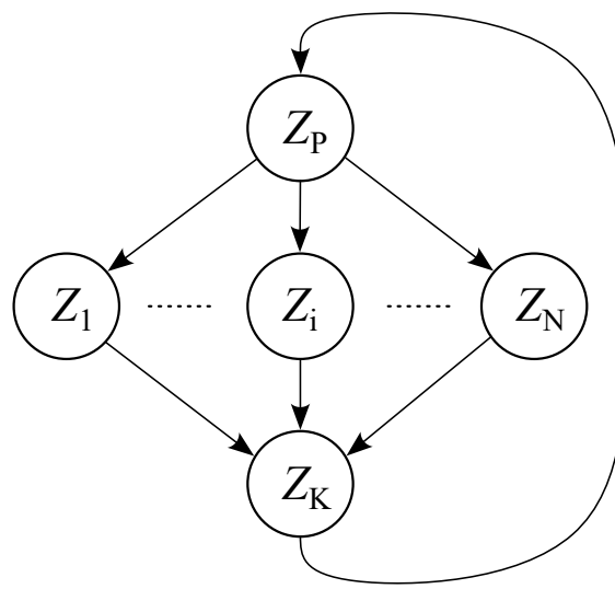
Slika 4.3. Uobičajena podjela posla na paralelne zadatke
