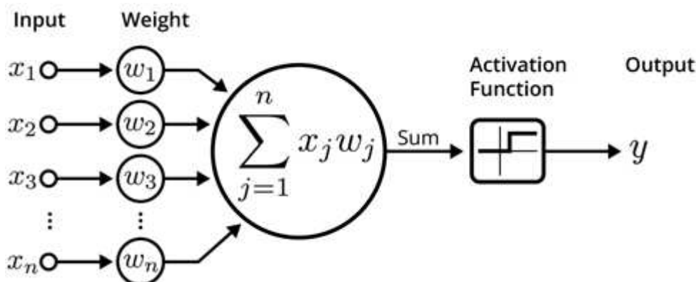
Slika 1. Vizualni prikaz modela neurona. [25]
