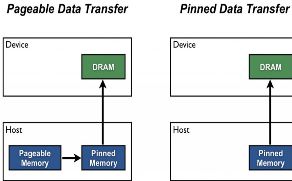
Slika 8.: Prikaz straničene i prikvačene memorije te prijenos s CPU na GPU [12]
