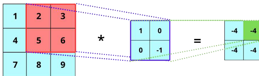
Slika 2.6. Primjer konvolucije 2x2. Objašnjenje rezultata: 2 \cdot 1 + 3 \cdot 0 + 5 \cdot 0 + 6 \cdot (-1) = -4
